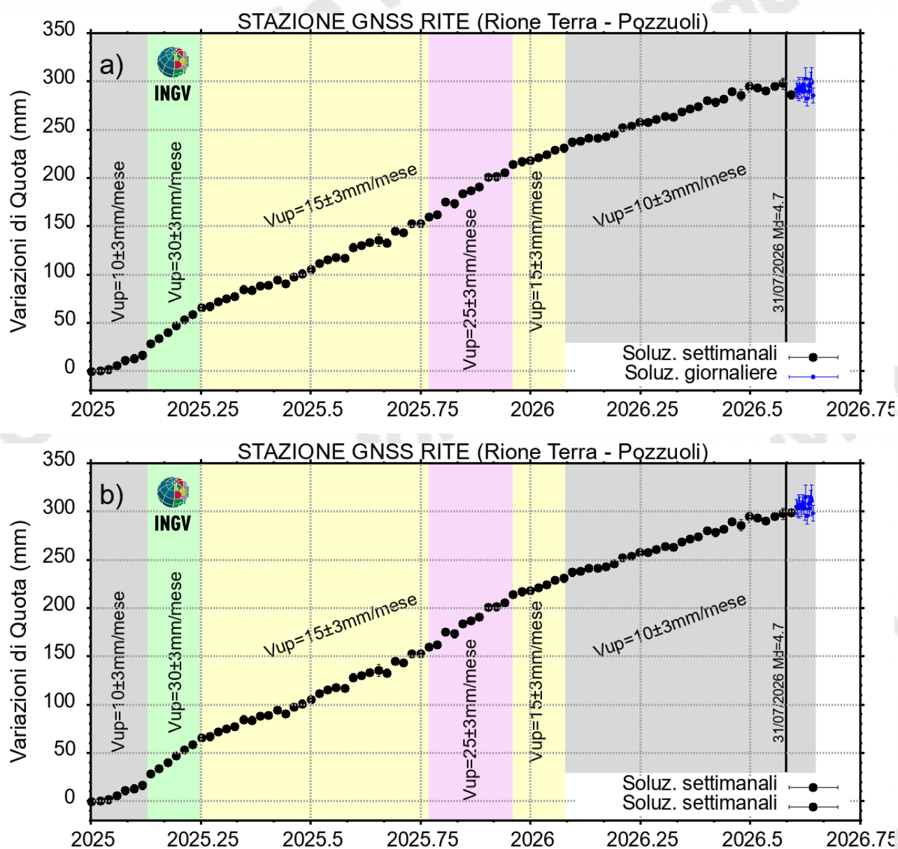
Figura 4.2 – Serie temporale delle variazioni in quota della stazione GNSS di RITE dal 01/01/2025 al 23/08/2026, con (a) e senza (b) la discontinuità cosismica del 31/07. Elaborazione dati in modalità differenziale singola baseline con software GNSS Spider.
