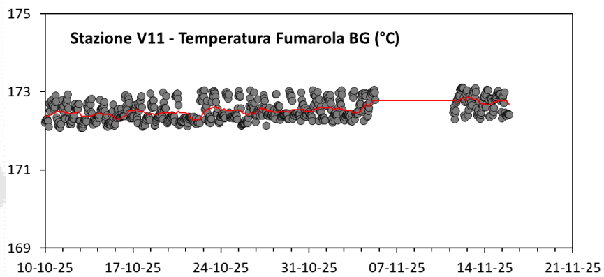
Figura 5.3 Valori della temperatura della fumarola BG misurati dalla stazione FLXOV5 (in alto) e dalla stazione V11 (in basso) installate nel cratere della Solfatara a pochi metri dalla fumarola principale BG. Si noti il trend di aumento degli ultimi anni misurato dalla stazione FLXOV5.
