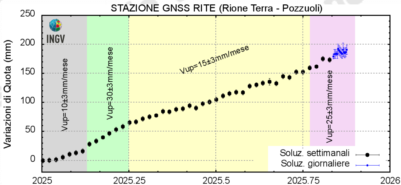
Figura 4.2 – Serie temporale delle variazioni in quota della stazione GNSS di RITE dal 01/01/2025 al 16/11/2025. Elaborazione dati in modalità differenziale singola baseline con software GNSS Spider.
