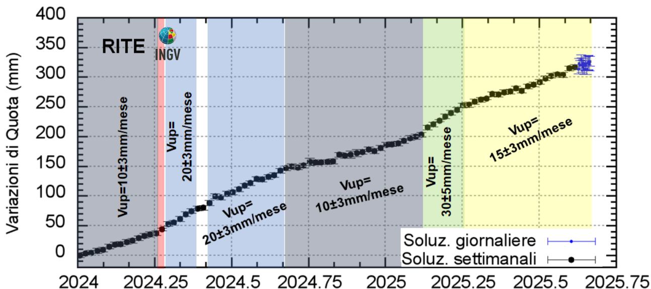
Figura 4.2 – Serie temporale delle variazioni in quota della stazione GNSS di RITE dal 01/01/2024 al 31/08/2025. Elaborazione dati in modalità differenziale singola baseline con software GNSS Spider.
