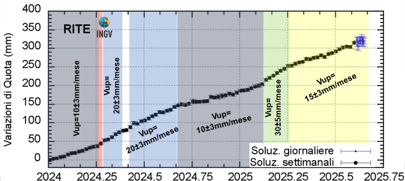
Figura 4.2 – Serie temporale delle variazioni in quota della stazione GNSS di RITE dal 01/01/2024 al 25/08/2025. Elaborazione dati in modalità differenziale singola baseline con software GNSS Spider.
