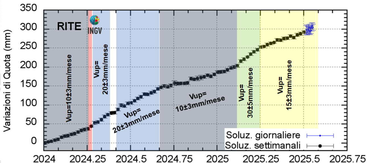
Figura 4.2 – Serie temporale delle variazioni in quota della stazione GNSS di RITE dal 01/01/2024 al 21/07/2025. Elaborazione dati in modalità differenziale singola baseline con software GNSS Spider.
