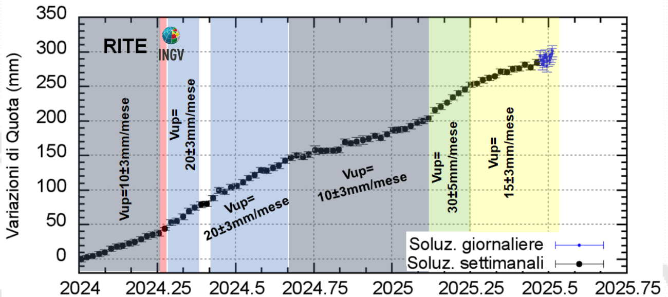
Figura 4.2 – Serie temporale delle variazioni in quota della stazione GNSS di RITE dal 01/01/2024 al 06/07/2025. Elaborazione dati in modalità differenziale singola baseline con software GNSS Spider.
