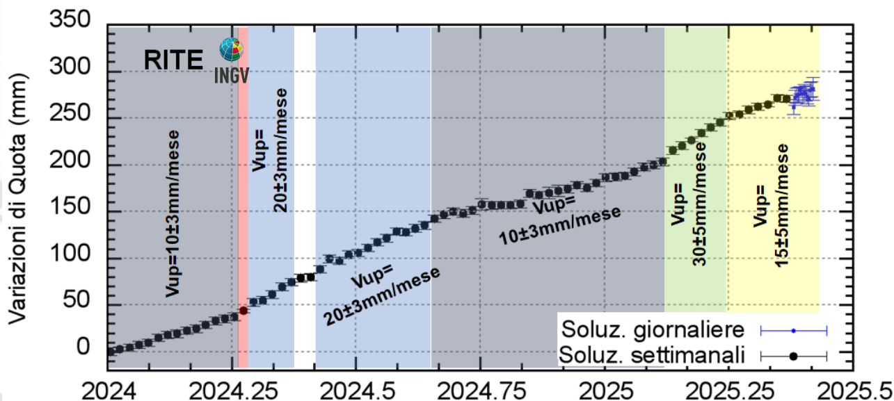
Figura 4.2 – Serie temporale delle variazioni in quota della stazione GNSS di RITE dal 01/01/2024 al 02/06/2025. Elaborazione dati in modalità differenziale singola baseline con software GNSS Spider.
