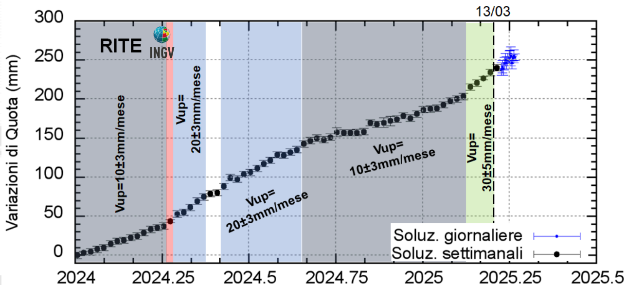
Figura 4.2 – Serie temporale delle variazioni in quota della stazione GNSS di RITE dal 01/01/2024 al 07/04/2025. Elaborazione dati in modalità differenziale singola baseline con software GNSS Spider.
