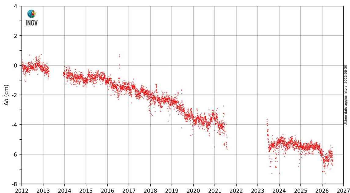
Figura 2.3.2 – Movimenti verticali del suolo, nel periodo gennaio 2012 – giugno 2026, ottenuti dall'analisi dei dati acquisiti dalla stazione mareografica di Torre del Greco, molo Redentore (TRDG). Le variazioni, riportate in cm, rappresentano le medie giornaliere e sono riferite alla stazione mareografica di Napoli, molo San Vincenzo (NAMM).
