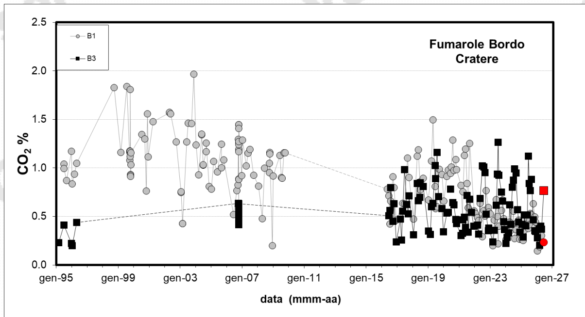
Figura 4.2 - Cronogramma della concentrazione di CO 2 delle fumarole di bordo cratere B1 (area anemometro) e B3 (settore SW). I campioni delle fumarole B1 e B3 del mese di giugno 2026 sono riportati con il simbolo rosso.
