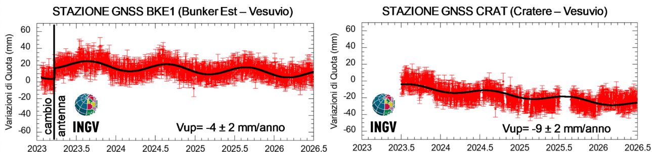
Figura 2.1.2 - Serie temporali delle variazioni giornaliere della componente verticale delle stazioni BKE1 e CRAT (Vesuvio) da gennaio 2023 a giugno 2026.
