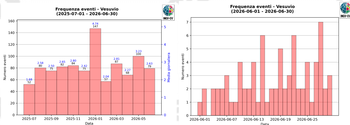
Figura 1.2 - A sinistra il numero di eventi registrati al Vesuvio nel corso degli ultimi 12 mesi (in totale 986), mentre a destra quelli avvenuti nell'ultimo mese (in totale 79).
