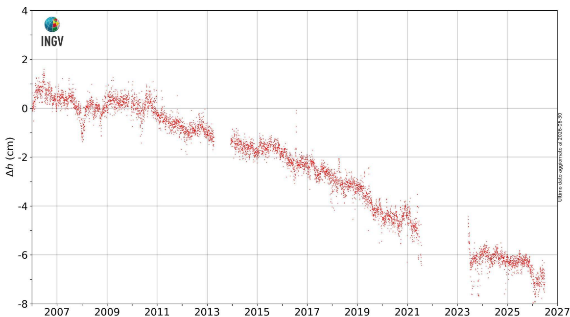
Figura 2.3.3 - Movimenti verticali del suolo, nel periodo gennaio 2006 – giugno 2026, ottenuti dall'analisi dei dati acquisiti dalla stazione mareografica di Torre del Greco, molo Redentore (TRDG). Le variazioni, riportate in cm, rappresentano le medie giornaliere e sono riferite alla stazione mareografica di Napoli molo San Vincenzo (NAMM).
