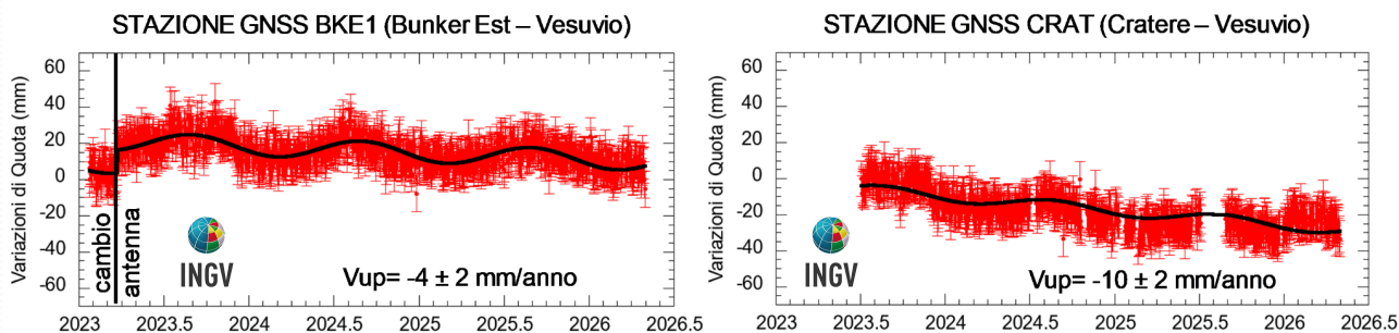
Figura 2.1.2 - Serie temporali delle variazioni giornaliere della componente verticale delle stazioni BKE1 e CRAT (Vesuvio) da gennaio 2023 ad aprile 2026.
