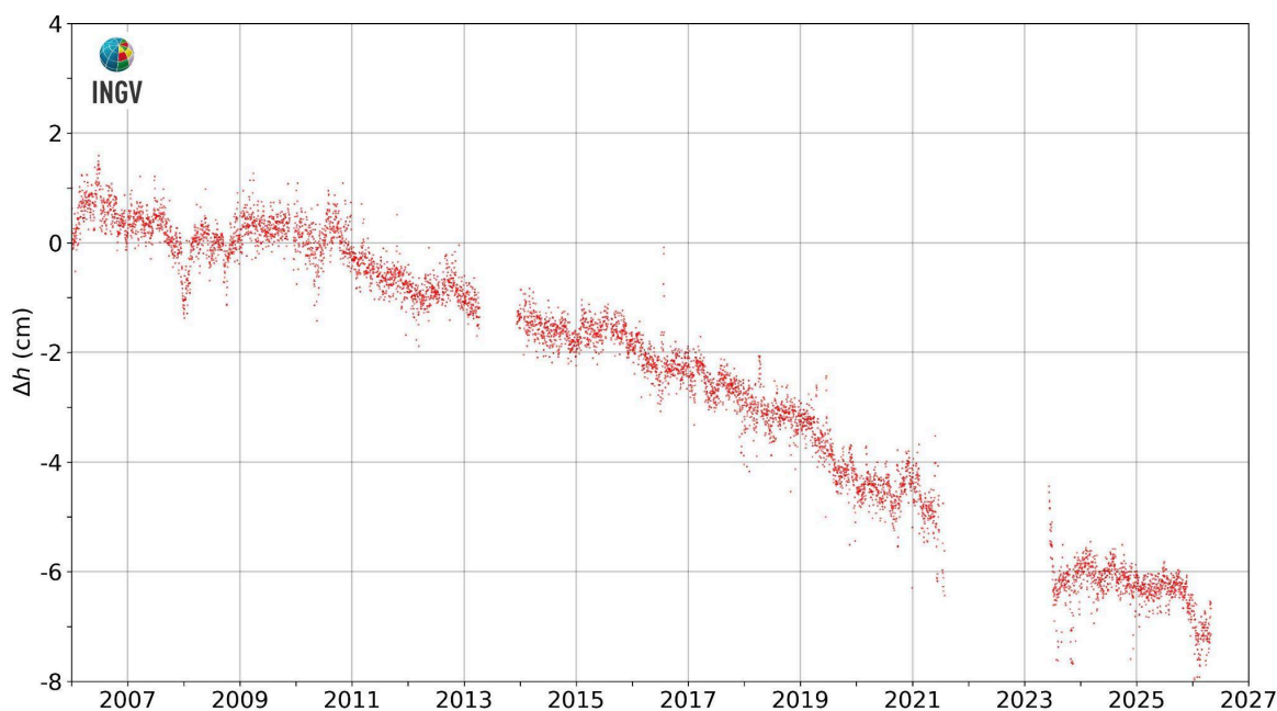
Figura 2.3.3 - Movimenti verticali del suolo, nel periodo gennaio 2006 – aprile 2026, ottenuti dall'analisi dei dati acquisiti dalla stazione mareografica di Torre del Greco, molo Redentore (TRDG). Le variazioni, riportate in cm, rappresentano le medie giornaliere e sono riferite alla stazione mareografica di Napoli molo San Vincenzo (NAMM).
