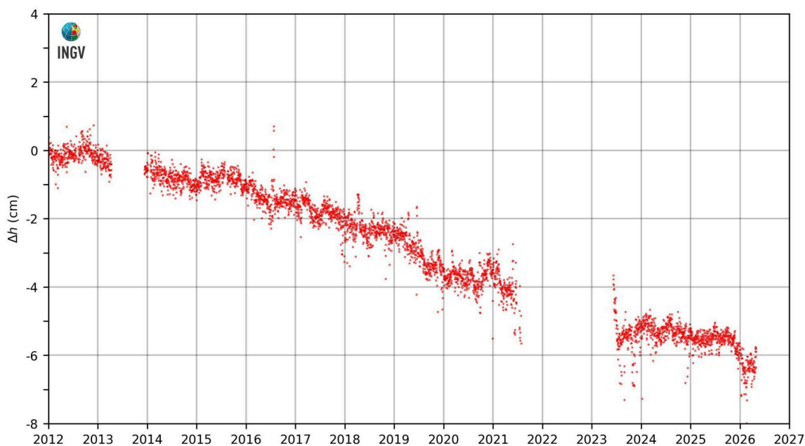
Figura 2.3.2 – Movimenti verticali del suolo, nel periodo gennaio 2012 – aprile 2026, ottenuti dall'analisi dei dati acquisiti dalla stazione mareografica di Torre del Greco, molo Redentore (TRDG). Le variazioni, riportate in cm, rappresentano le medie giornaliere e sono riferite alla stazione mareografica di Napoli, molo San Vincenzo (NAMM).
