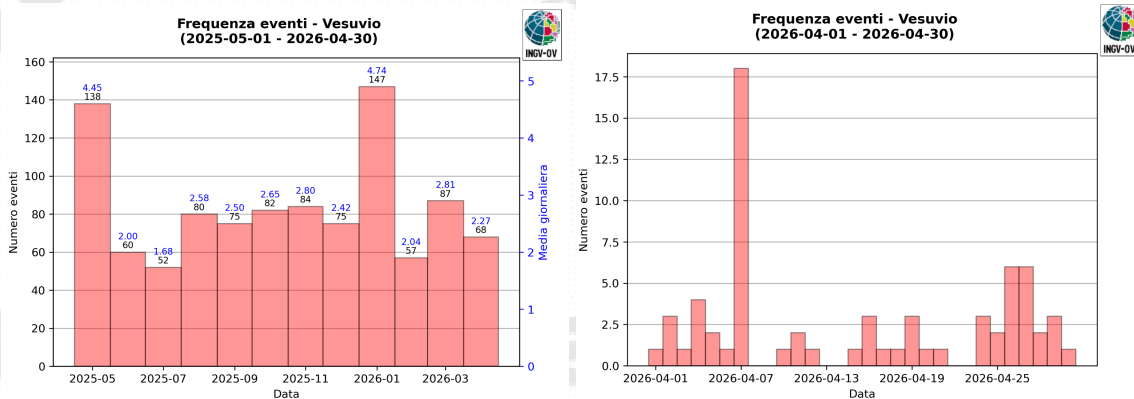
Figura 1.2 - A sinistra il numero di eventi registrati al Vesuvio nel corso degli ultimi 12 mesi (in totale 1005), mentre a destra quelli avvenuti nell'ultimo mese (in totale 68).
