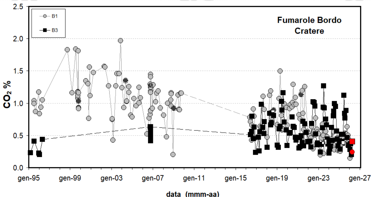
Figura 4.2 - Cronogramma della concentrazione di CO 2 delle fumarole di bordo cratere B1 (area anemometro) e B3 (settore SW). I campioni delle fumarole B1 e B3 del mese di aprile 2026 sono riportati con il simbolo rosso.
