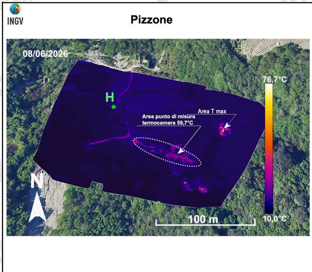
Figura 3.5 – Località Pizzone. Fotocomposizione di immagini termiche rilevate da drone nel mese di giugno 2026 (area rosa "Piz" in Figura 3.1). H* indica il sito di decollo e di atterraggio del drone. L'area racchiusa dalla linea tratteggiata bianca è quella dove vengono effettuate le misure termiche discrete (sito "Piz" di Figura 3.1).
