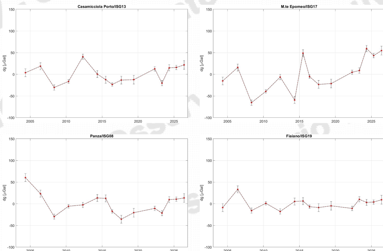
Figura 2.3.3. Serie temporali di alcune stazioni della rete gravimetrica di Ischia a partire dal 2004. Si notano le oscillazioni dei residui gravimetrici, in alcuni casi superiori alle decine di \mu\text{Gal} . Queste oscillazioni sono generalmente attribuibili alla dinamica del sistema idrotermale dell'isola e a fenomeni idrologici a carattere stagionale.
