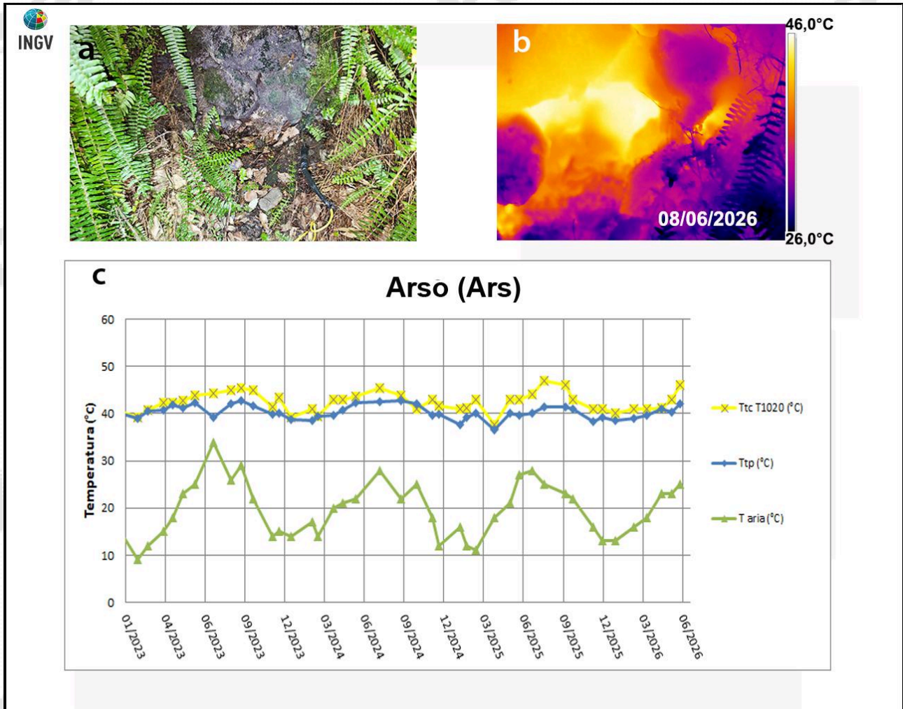
Figura 3.2 - Cratere dell'Arso a Ischia. Immagini nel visibile (a) e termica (b) riprese dal punto stazione Ars di Figura 3.1. Il grafico (c) riporta la serie temporale (gennaio 2023 – giugno 2026) dei valori massimi di temperatura con termocamera FLIR T1020 (TtcT1020) e con termocoppia (Ttp), confrontati con la temperatura dell'aria (Taria) misurata nel momento del rilievo termico.
