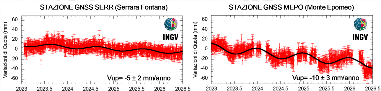
Figura 2.1.2 - Serie temporali delle variazioni giornaliere della componente verticale delle stazioni di SERR e MEPO (Ischia) da gennaio 2023 a giugno 2026.
