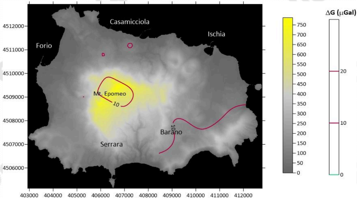
Figura 2.3.2. Residui gravimetrici ricavati dalla differenza tra i valori di \Delta G della campagna 2026 e della precedente del 2024. Non si evidenziano variazioni significative che sono al limite dell'errore statistico ( 10\mu\text{Gal} )
