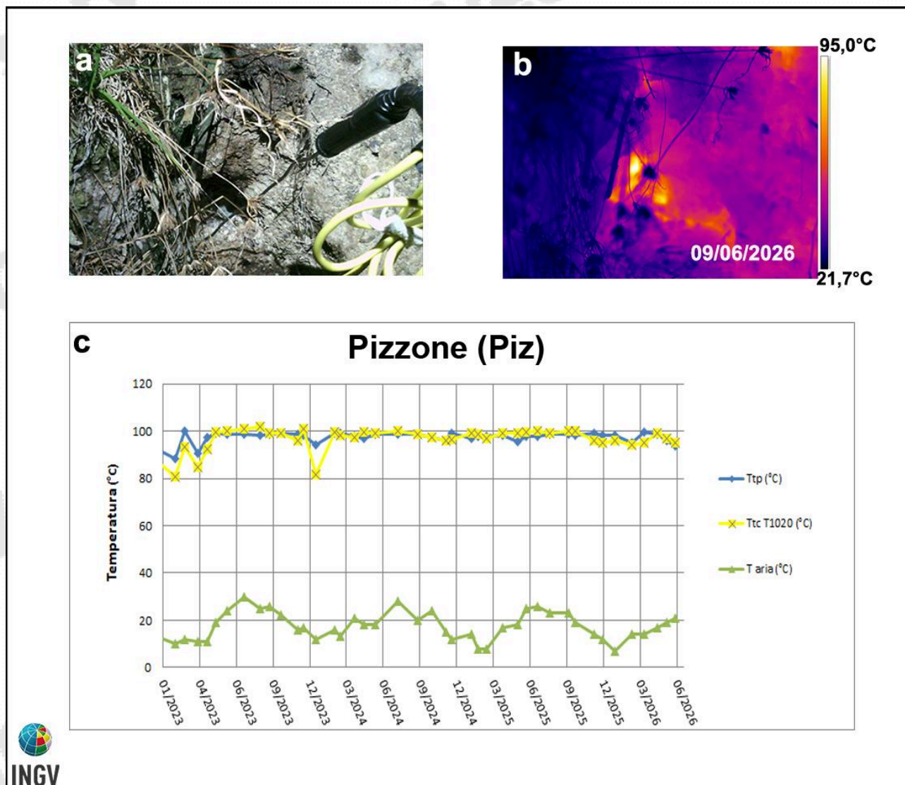
Figura 3.4 – Fumarola in località Pizzone a Ischia. Immagini nel visibile (a) e termica (b) riprese dal punto stazione Piz di Fig. 3.1. Il grafico (c) riporta la serie temporale (gennaio 2023 – giugno 2026) dei valori massimi di temperatura con termocamera FLIR T1020 (TtcT1020) e con termocoppia (Ttp), confrontati con la temperatura dell'aria (Taria) misurata nel momento del rilievo termico.
