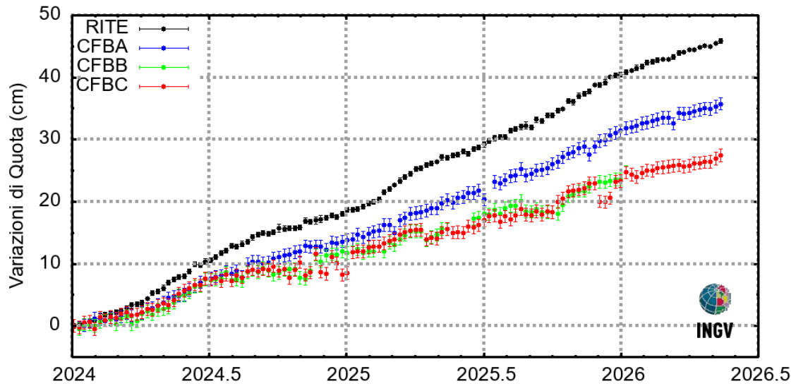
Figura 2.1.6 – Serie temporali delle variazioni settimanali in quota delle stazioni GNSS dell'infrastruttura marina MEDUSA nell'intervallo gennaio 2024 - maggio 2026, confrontate con quella della stazione RITE
