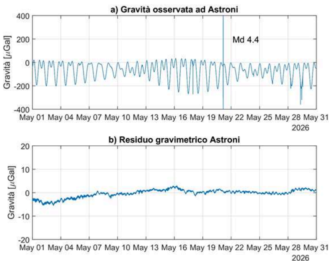
Figura 2.4.1 - a: serie temporale (risoluzione temporale 1 minuto) raw registrata dal gPhone. Si osserva il contributo dominante delle maree. b: serie residua di gravità.
