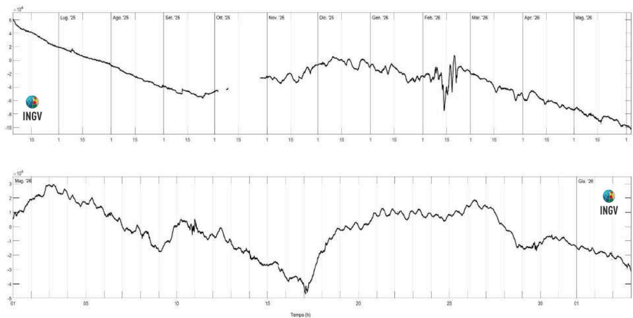
Figura 2.5.3 - In alto: Strain registrato nell'ultimo anno alla stazione di Monterusciello, dalle 00:00 UTC del 02/06/2025 alle 16:00 UTC del giorno 03/06/2026. In basso: Strain registrato nell'ultima settimana alla stazione di Monterusciello, dalle 00:00 del 1/05/2026 alle 16:00 del 03/06/2026.
