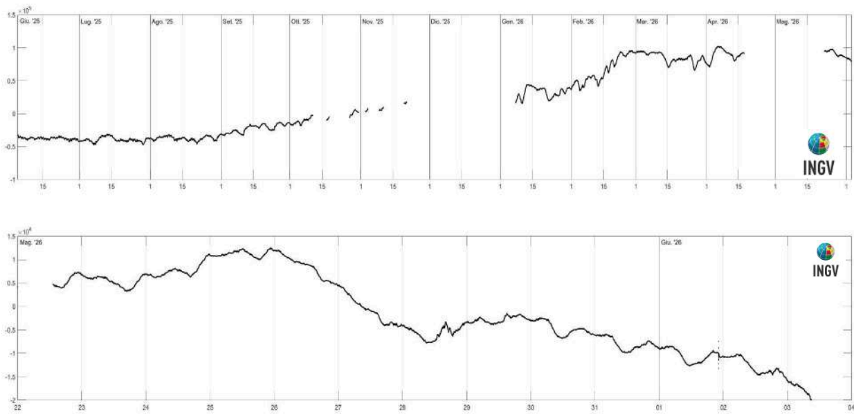
Figura 2.5.2 - Strain registrato dalla stazione dilatometrica di Quarto. In alto è mostrato lo strain registrato nell'ultimo anno, dalle 00:00 UTC del 2/06/2025 alle 12:00 UTC del 03/06/2026. In basso, i dati di strain disponibili nell'ultimo periodo, dalle 12:00 UTC del 22/05/2026 alle 12:00 UTC del 03/06/2026.
