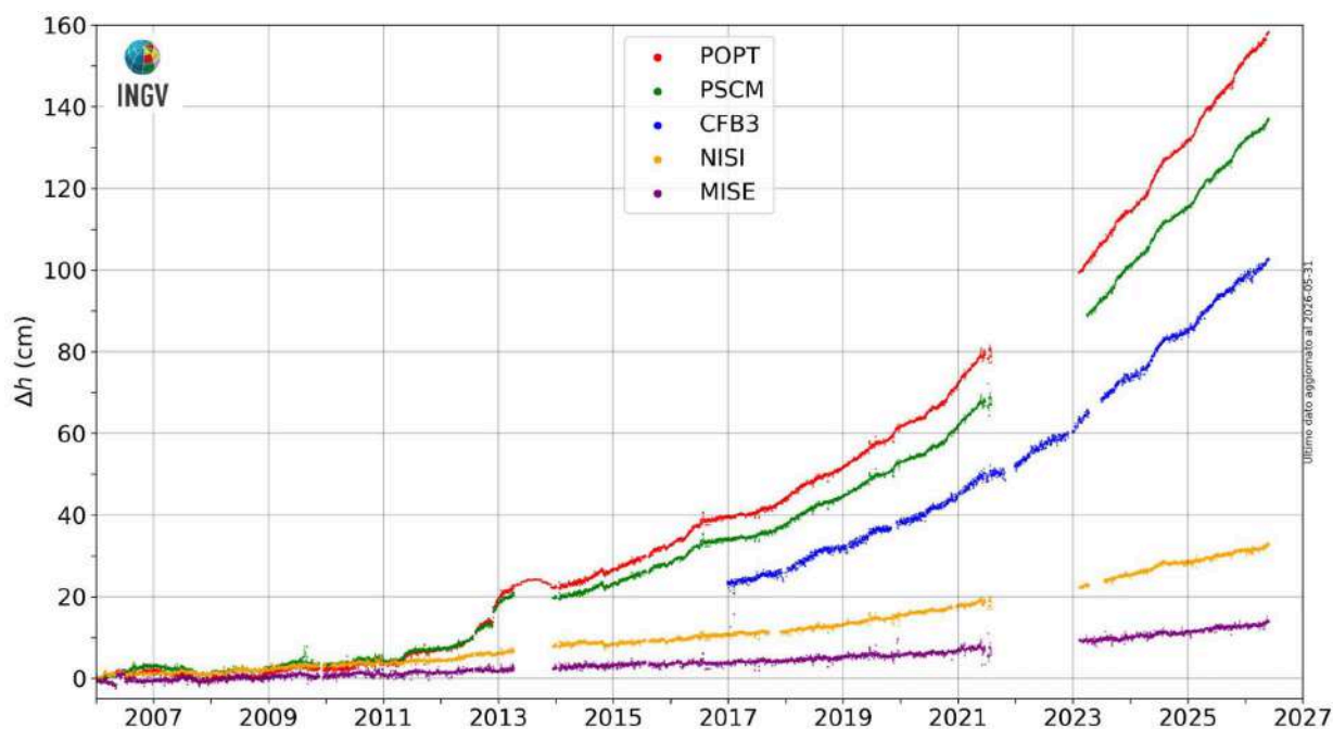
Figura 2.3.4 - Movimenti verticali del suolo nel periodo gennaio 2006 – maggio 2026, ottenuti dall'analisi dei dati acquisiti da tutte le stazioni mareografiche dell'area della caldera Flegrea. Le variazioni, riportate in cm, rappresentano le medie giornaliere e sono tutte riferite alla stazione mareografica di Napoli, molo San Vincenzo (NAMM).
