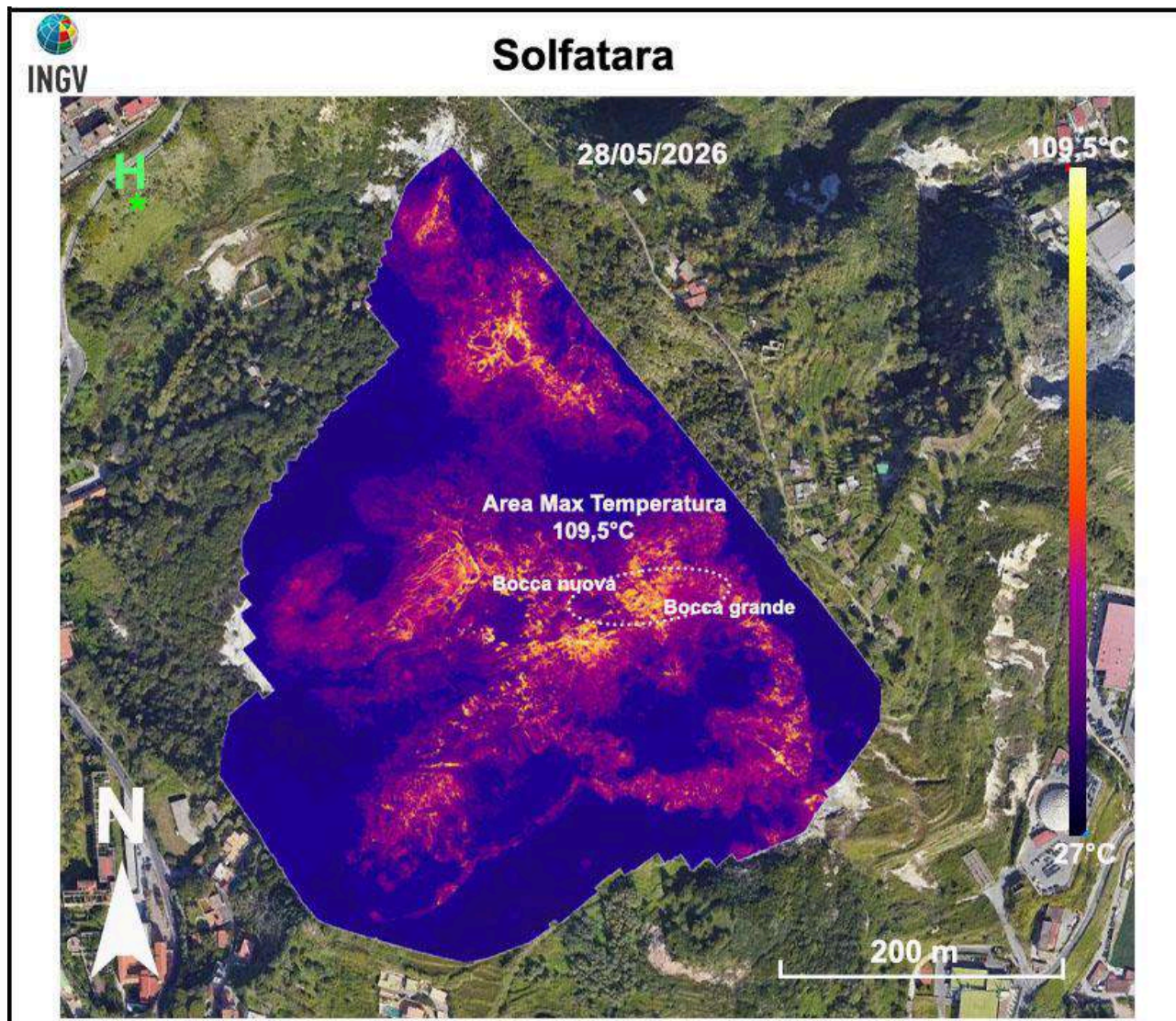
Figura 3.2.4 – Fotocomposizione di immagini termiche rilevate da drone nel mese di giugno 2025 su La Solfatara (Solf in figura 3.2.1.B). H* indica il sito di decollo e di atterraggio del drone corrispondente al punto S1 di Fig.3.2.1.B.
