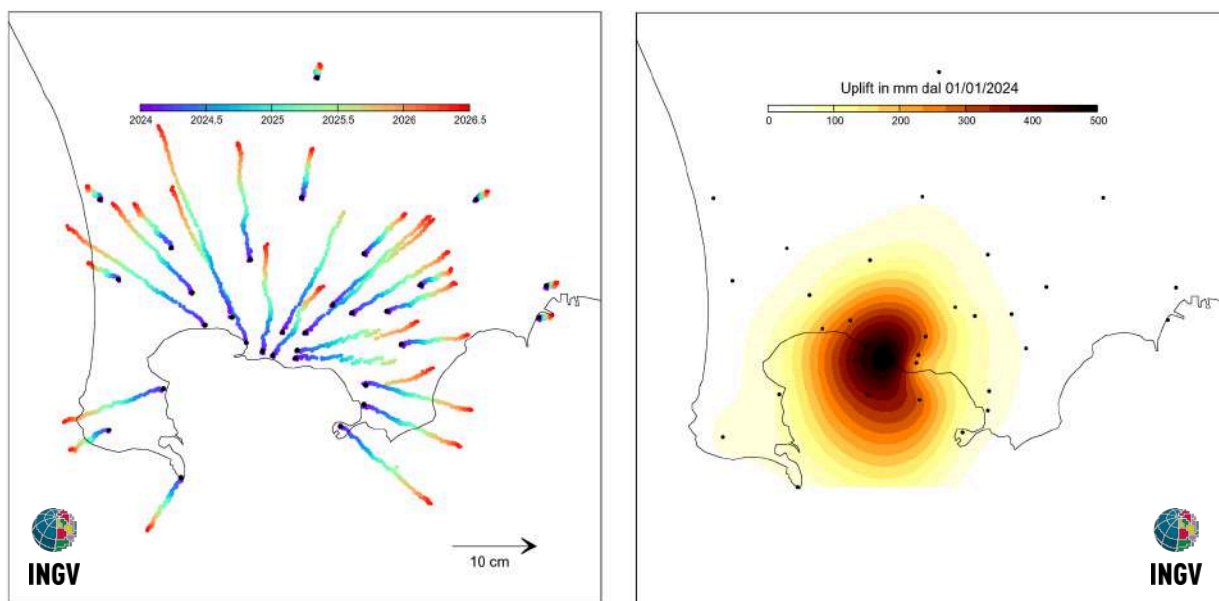
Figura 2.1.5 - Mappa degli spostamenti GNSS orizzontali (a) e verticali (b) registrati nell’area flegrea da gennaio 2024 a maggio 2026.
