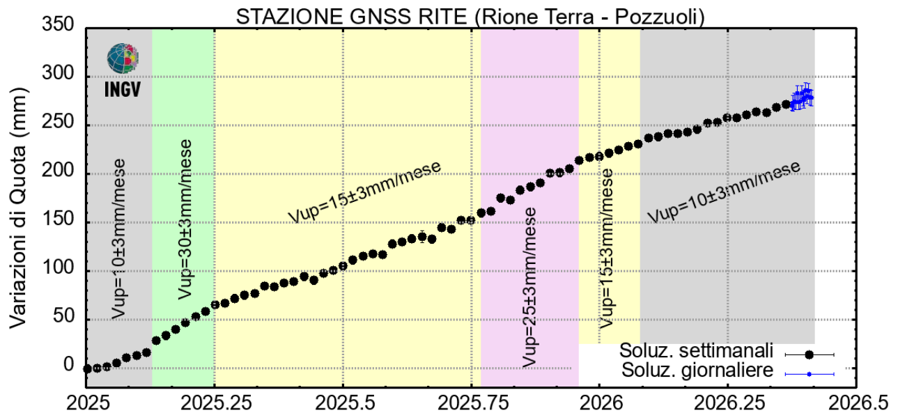
Figura 2.1.2 - Serie temporale delle variazioni in quota della stazione GNSS di RITE dal 01/01/2025 al 31/05/2026. Elaborazione dati in modalità differenziale singola baseline con software GNSS Spider.
