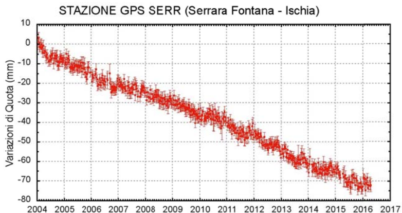
Figura 3.2.1 - Serie temporale delle variazioni settimanali in quota della stazione di SERR (Ischia) dal 2004 ad aprile 2016.
