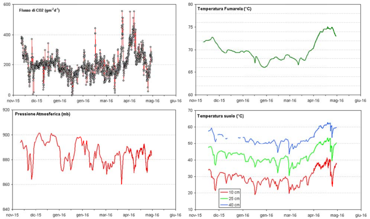
Figura 1.4.4 - Parametri misurati dalla stazione geochimica installata in area bordo cratere del Vesuvio (settore SW).
