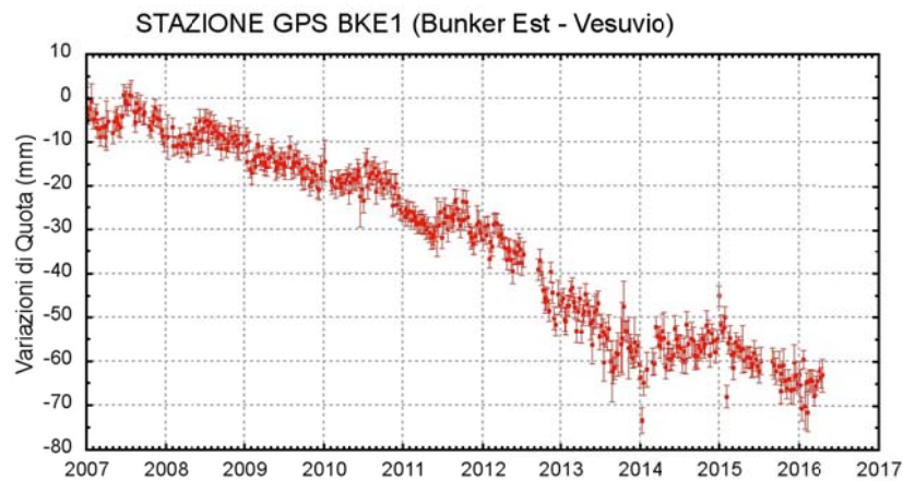
Figura 1.2.1 - Serie temporale delle variazioni settimanali in quota della stazione di BKE1 (Vesuvio) dal 2007 ad aprile 2016.
