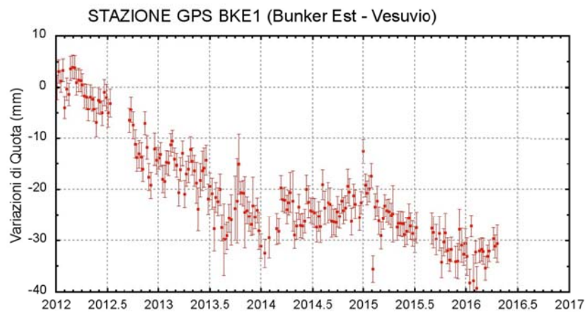
Figura 1.2.2 - Serie temporale delle variazioni settimanali in quota della stazione di BKE1 (Vesuvio) da gennaio 2012 ad aprile 2016.
