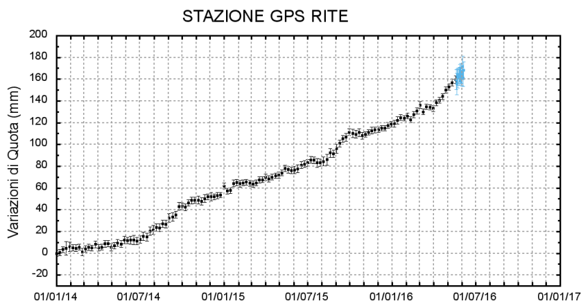
Figura 2.2.3 - Serie temporale delle variazioni in quota della stazione di RITE (Pozzuoli) dal 01 gennaio 2014 al 05 giugno 2016.
