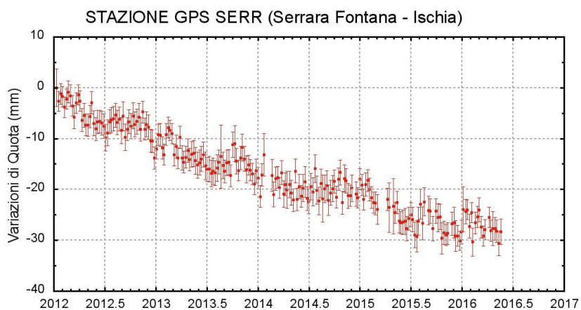
Figura 3.2.2 - Serie temporale delle variazioni settimanali in quota della stazione di SERR (Ischia) da gennaio 2012 a maggio 2016.
