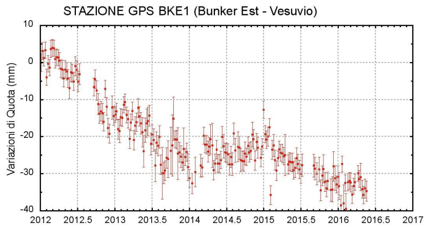
Figura 1.2.2 - Serie temporale delle variazioni settimanali in quota della stazione di BKE1 (Vesuvio) da gennaio 2012 a maggio 2016.
