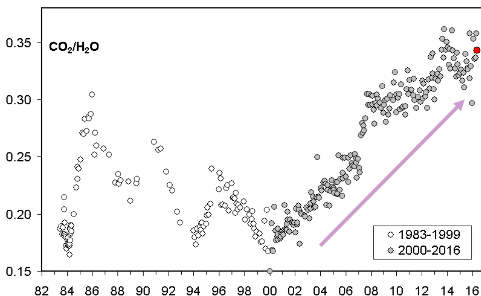
Figura 2.3.1 - Cronogramma del rapporto CO_2/H_2O per la fumarola BG. In grigio sono riportati dati a partire dal 2000, quando è iniziato un trend d'aumento del rapporto CO_2/H_2O , in generale, indicativo di una crescente frazione della componente magmatica nei fluidi fumarolici. Con il simbolo rosso è evidenziato il campione di maggio 2016.
