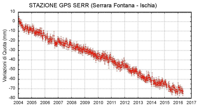
Figura 3.2.1 - Serie temporale delle variazioni settimanali in quota della stazione di SERR (Ischia) dal 2004 a maggio 2016.
