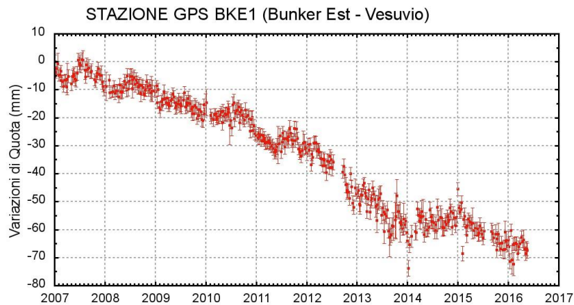
Figura 1.2.1 - Serie temporale delle variazioni settimanali in quota della stazione di BKE1 (Vesuvio) dal 2007 a maggio 2016
