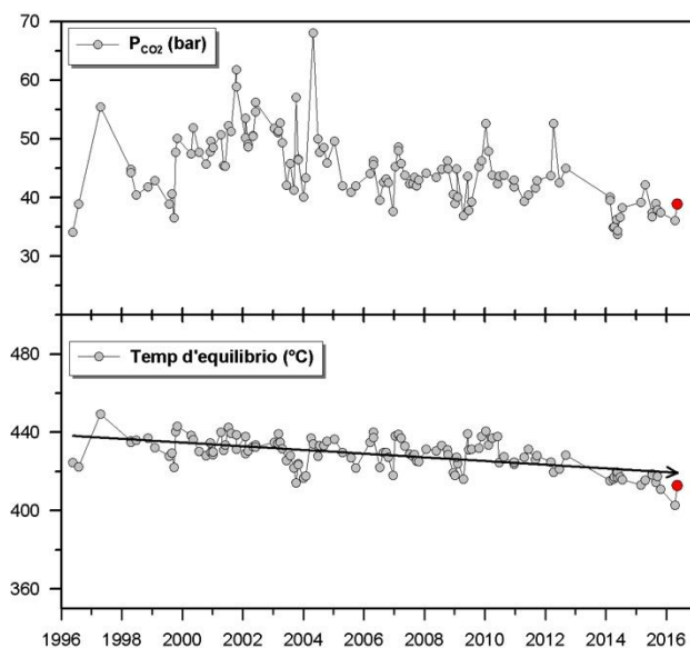
Figura 1.4.2 - Cronogramma dei valori d'equilibrio della temperatura e pressione parziale di CO_2 stimati per il sistema idrotermale del Vesuvio. Il campione di Maggio 2016 è riportato con il simbolo rosso.
