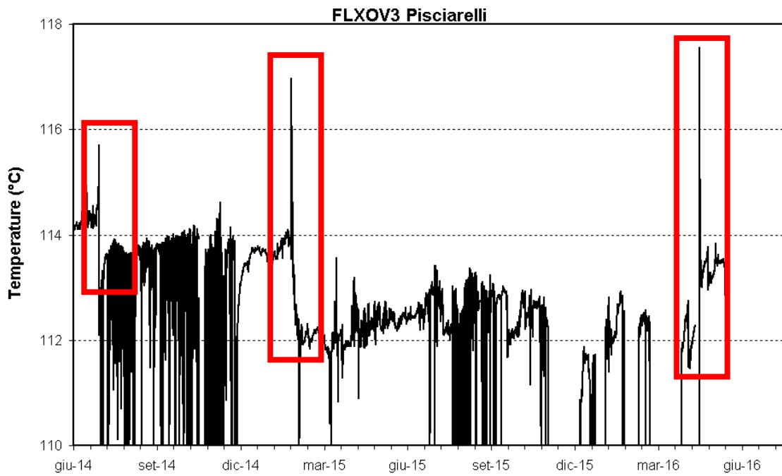
Figura 2.3.7 - Temperature registrate in continuo della fumarola di Pisciarelli.
