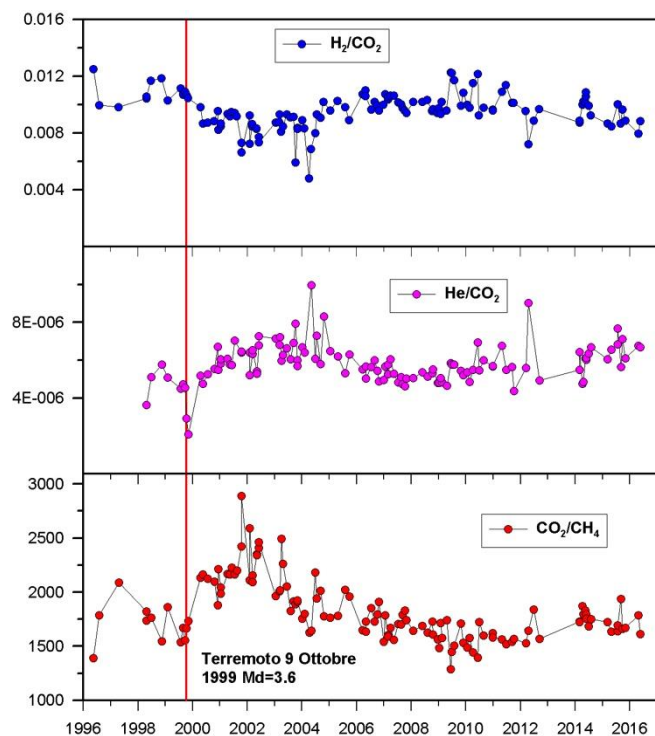
Figura 1.4.1 - Variazioni composizionali della fumarola FC2 nel periodo 1996-2016.
