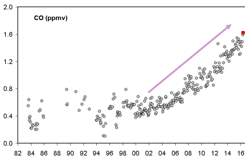
Figura 2.3.2 - Variazioni della concentrazione di monossido di carbonio (CO) misurato alla fumarola BG a partire dal 1983. Con il simbolo rosso è evidenziato il campione di maggio 2016. In generale alti contenuti di CO caratterizzano sistemi vulcanici ad elevata temperatura mentre fumarole alimentate da sistemi idrotermali mostrano concentrazioni più basse, in tali sistemi un aumento delle concentrazioni di CO può riflettere un incremento delle condizioni di pressione e temperatura.
