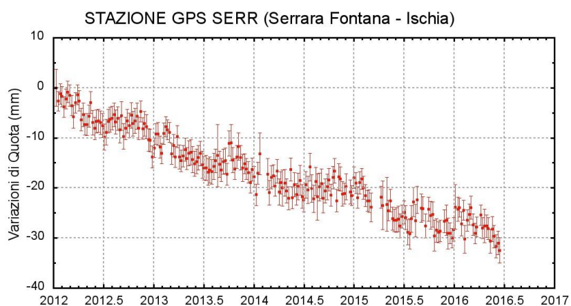
Figura 3.2.2 - Serie temporale delle variazioni settimanali in quota della stazione di SERR (Ischia) da gennaio 2012 a giugno 2016.
