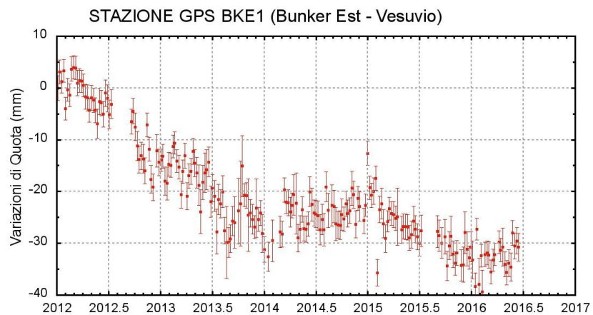
Figura 1.2.2 - Serie temporale delle variazioni settimanali in quota della stazione di BKE1 (Vesuvio) da gennaio 2012 a giugno 2016.
