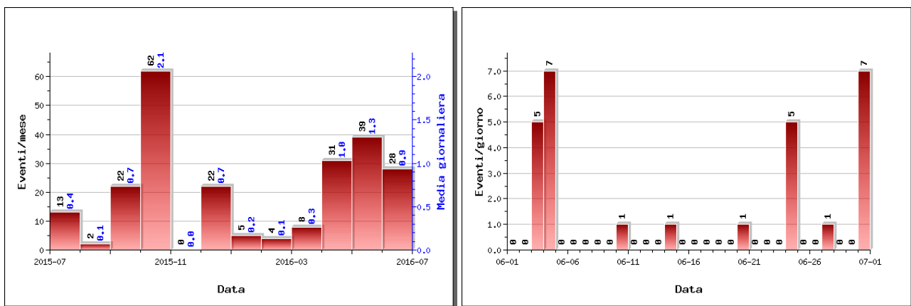
Figura 2.1.1 – A sinistra numero di eventi registrati ai Campi Flegrei nel corso degli ultimi 12 mesi (in totale 236), mentre a destra quelli avvenuti nell'ultimo mese (in totale 28).
