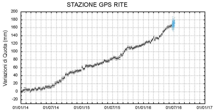
Figura 2.2.3 - Serie temporale delle variazioni in quota della stazione di RITE (Pozzuoli) dal 01 gennaio 2014 al 04 luglio 2016.
