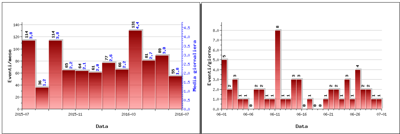
Figura 1.1.1 – A sinistra il numero di eventi registrati al Vesuvio nel corso degli ultimi 12 mesi (in totale 953), mentre a destra quelli avvenuti nell'ultimo mese (in totale 55).
