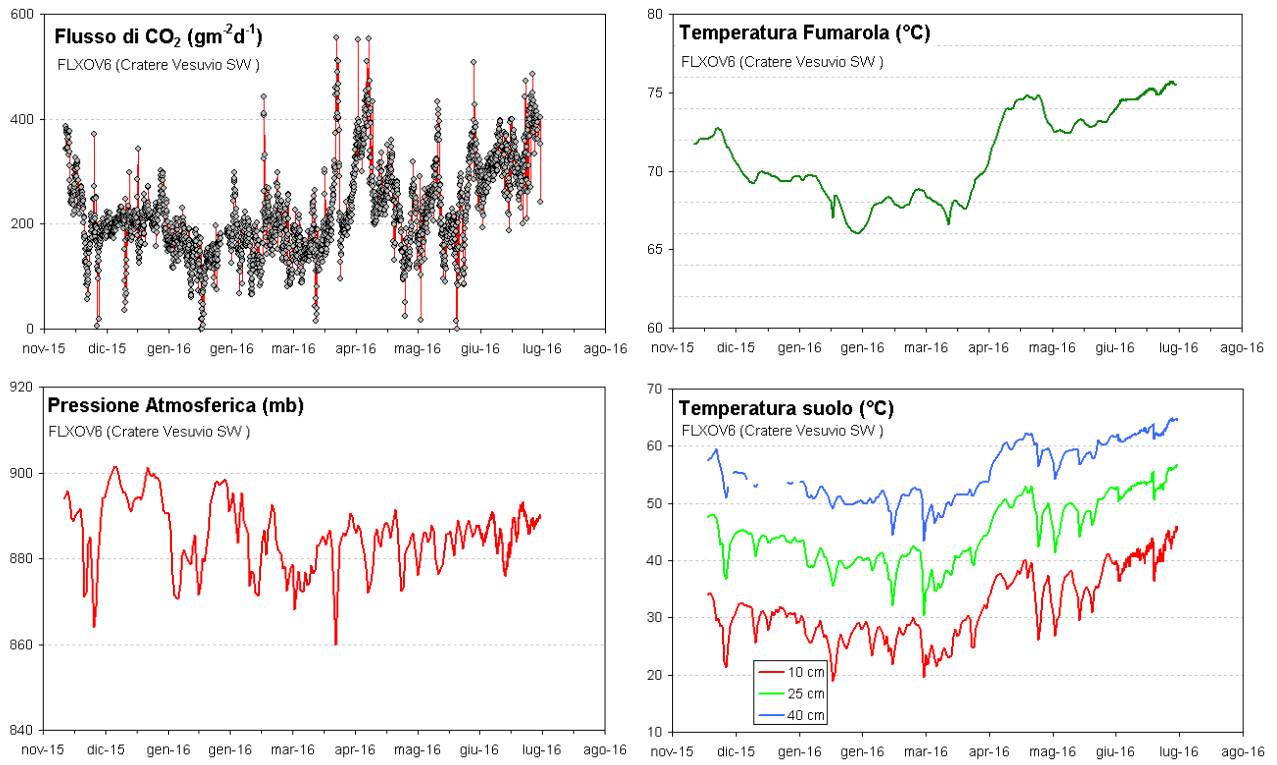
Figura 1.4.4 - Parametri misurati dalla stazione geochimica (FLXOV6) installata in area bordo cratere del Vesuvio (settore SW).
