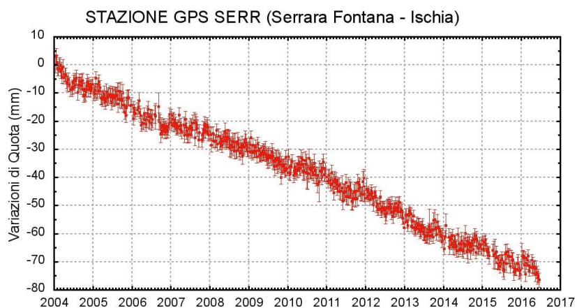
Figura 3.2.1 - Serie temporale delle variazioni settimanali in quota della stazione di SERR (Ischia) dal 2004 a giugno 2016.
