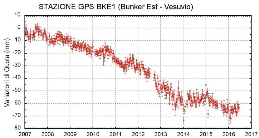
Figura 1.2.1 - Serie temporale delle variazioni settimanali in quota della stazione di BKE1 (Vesuvio) dal 2007 a giugno 2016.
