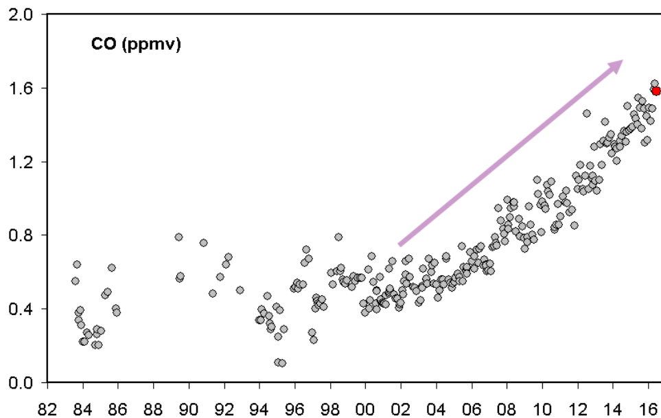
Figura 2.3.2 - Variazioni della concentrazione di monossido di carbonio (CO) misurato alla fumarola BG a partire dal 1983. Con il simbolo rosso è evidenziato il campione di Giugno 2016. In generale alti contenuti di CO caratterizzano sistemi vulcanici ad elevata temperatura mentre fumarole alimentate da sistemi idrotermali mostrano concentrazioni più basse, in tali sistemi un aumento delle concentrazioni di CO può riflettere un incremento delle condizioni di pressione e temperatura.
