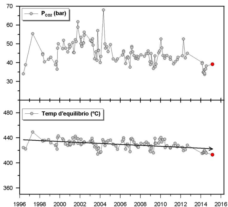
Figura 1.4.2 - Cronogramma dei valori d'equilibrio della temperatura e pressione parziale di CO 2 stimati per il sistema idrotermale del Vesuvio. Il campione di marzo 2015 è riportato con il simbolo rosso.
