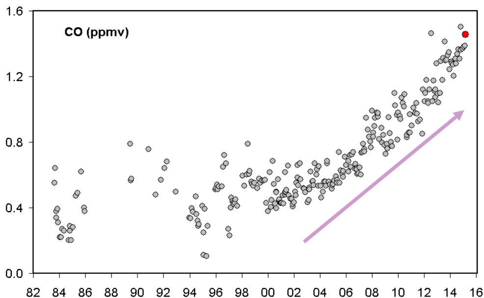
Figura 2.3.2 - Variazioni della concentrazione di monossido di carbonio (CO) misurato alla fumarola BG a partire dal 1983. In rosso è evidenziato il campione relativo al mese di Marzo 2015. In generale alti contenuti di CO caratterizzano sistemi vulcanici ad elevata temperatura mentre fumarole alimentate da sistemi idrotermali mostrano concentrazioni più basse, in tali sistemi un aumento delle concentrazioni di CO può riflettere un incremento delle condizioni di pressione e temperatura.
