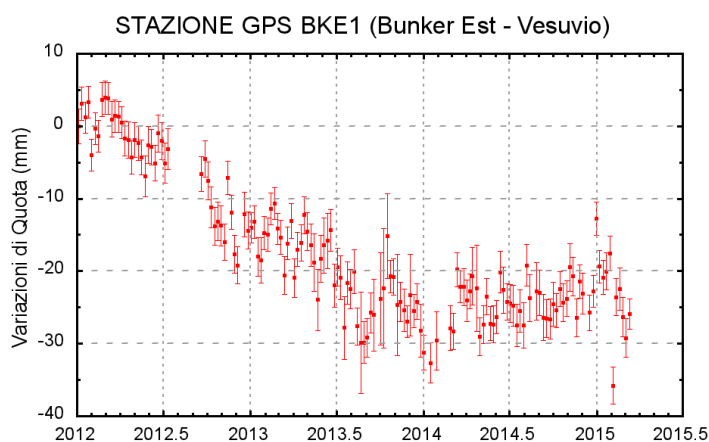
Figura 1.2.2 - Serie temporale delle variazioni settimanali in quota della stazione di BKE1 (Vesuvio) da gennaio 2012 a marzo 2015
