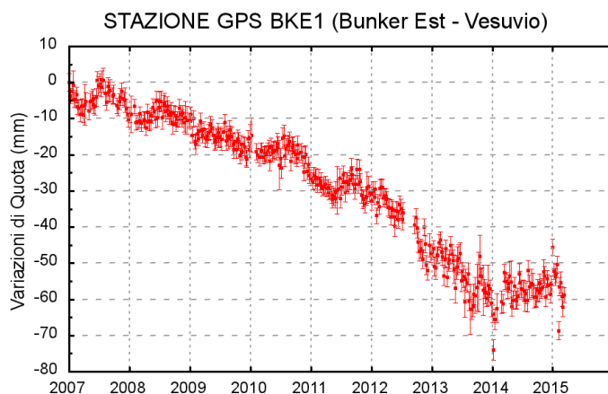
Figura 1.2.1 - Serie temporale delle variazioni settimanali in quota della stazione di BKE1 (Vesuvio) dal 2007 a marzo 2015
