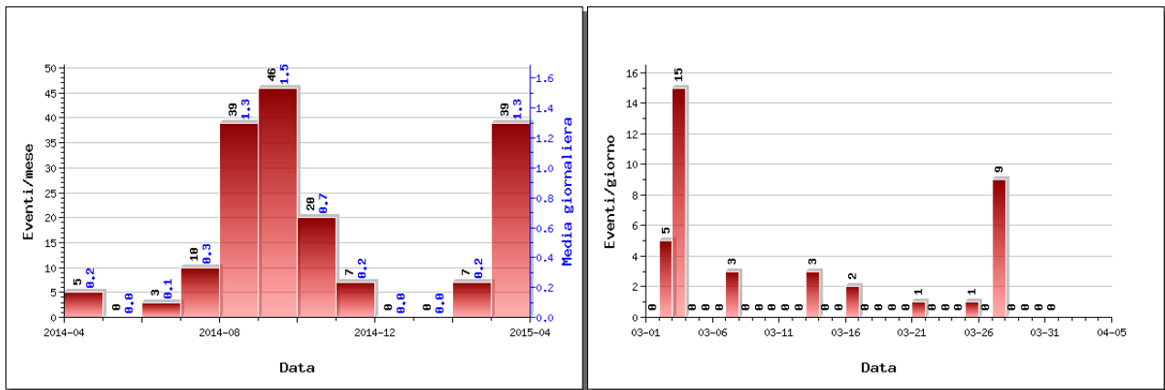
Figura 2.1.1 – A sinistra numero di eventi registrati ai Campi Flegrei nel corso degli ultimi 12 mesi (in totale 176), mentre a destra quelli avvenuti nell'ultimo mese (in totale 39).
