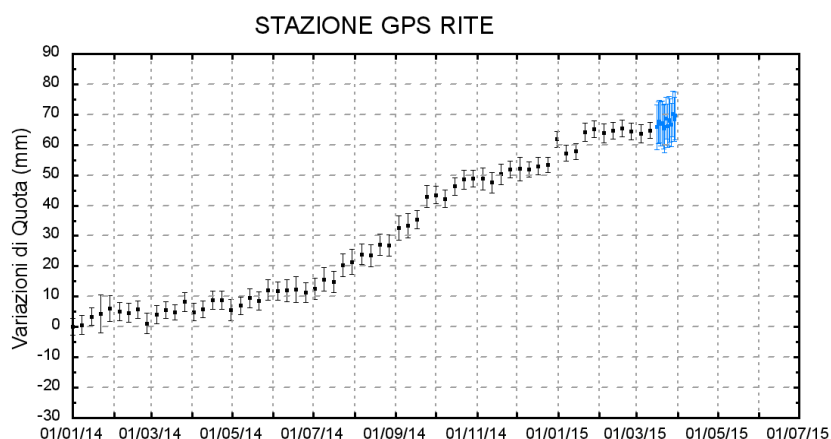
Figura 2.2.2 - Serie temporale delle variazioni in quota della stazione di RITE (Pozzuoli) dal 01 gennaio 2014 al 30 marzo 2015.
