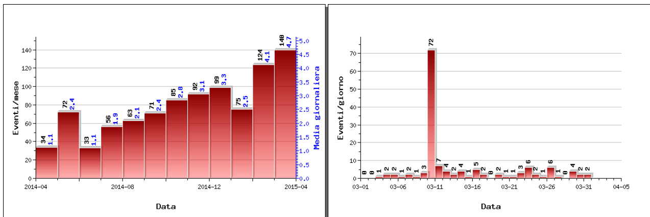
Figura 1.1.1 – A sinistra il numero di eventi registrati al Vesuvio nel corso degli ultimi 12 mesi (in totale 944), mentre a destra quelli avvenuti nell'ultimo mese (in totale 140).
