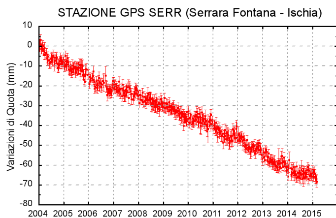
Figura 3.2.1 - Serie temporale delle variazioni settimanali in quota della stazione di SERR (Ischia) dal 2004 a marzo 2015
