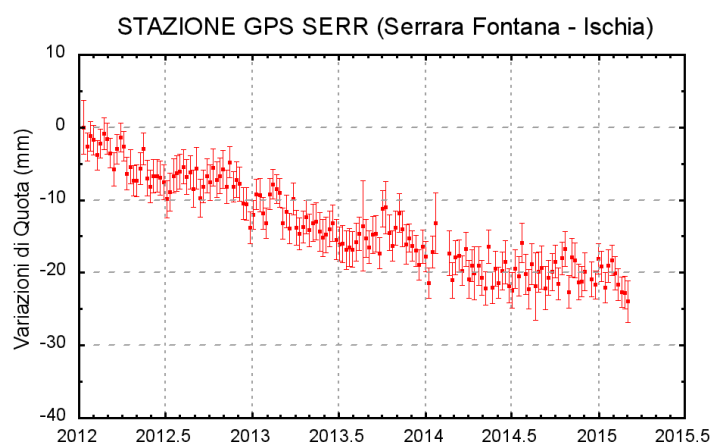
Figura 3.2.2 - Serie temporale delle variazioni settimanali in quota della stazione di SERR (Ischia) da gennaio 2012 a marzo 2015
