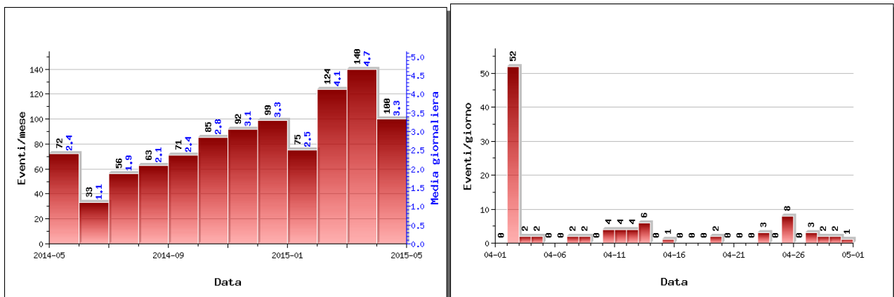
Figura 1.1.1 – A sinistra il numero di eventi registrati al Vesuvio nel corso degli ultimi 12 mesi (in totale 1010), mentre a destra quelli avvenuti nell'ultimo mese (in totale 100).
