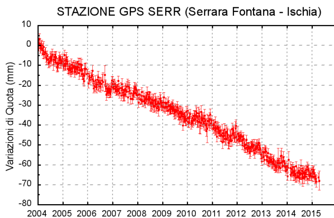
Figura 3.2.1 - Serie temporale delle variazioni settimanali in quota della stazione di SERR (Ischia) dal 2004 a aprile 2015.
