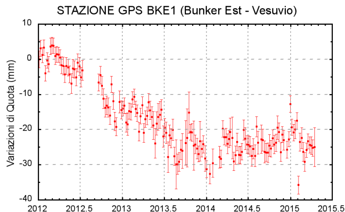
Figura 1.2.2 - Serie temporale delle variazioni settimanali in quota della stazione di BKE1 (Vesuvio) da gennaio 2012 a aprile 2015.
