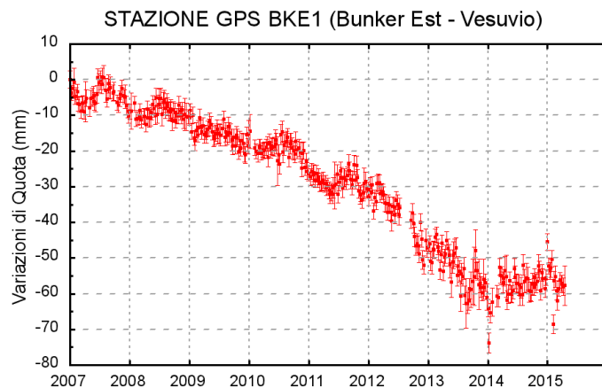
Figura 1.2.1 - Serie temporale delle variazioni settimanali in quota della stazione di BKE1 (Vesuvio) dal 2007 a aprile 2015.
