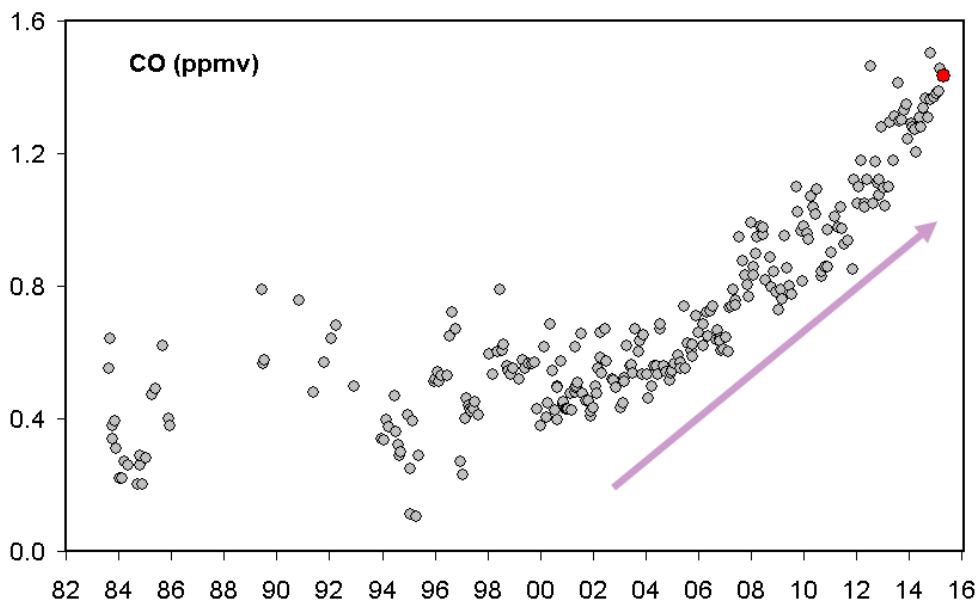
Figura 2.3.2 - Variazioni della concentrazione di monossido di carbonio (CO) misurato alla fumarola BG a partire dal 1983. In rosso è evidenziato il campione relativo al mese di Aprile 2015. In generale alti contenuti di CO caratterizzano sistemi vulcanici ad elevata temperatura mentre fumarole alimentate da sistemi idrotermali mostrano concentrazioni più basse, in tali sistemi un aumento delle concentrazioni di CO può riflettere un incremento delle condizioni di pressione e temperatura.
