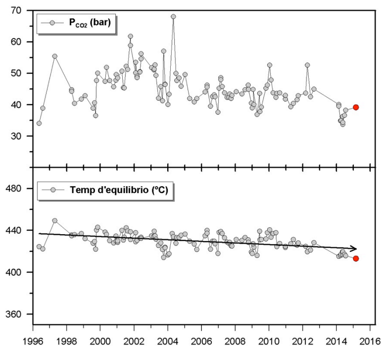
Figura 1.3.2 - Cronogramma dei valori d'equilibrio della temperatura e pressione parziale di CO 2 stimati per il sistema idrotermale del Vesuvio. Il campione di marzo 2015 è riportato con il simbolo rosso.
