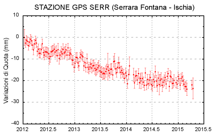
Figura 3.2.2 - Serie temporale delle variazioni settimanali in quota della stazione di SERR (Ischia) da gennaio 2012 a aprile 2015.
