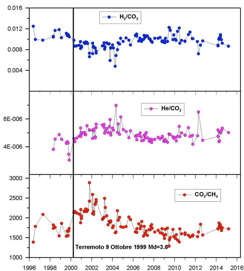
Figura 1.3.1 - Variazioni composizionali della fumarola FC2 nel periodo 1996-2015.
