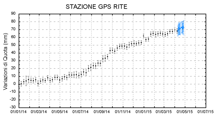
Figura 2.2.2 - Serie temporale delle variazioni in quota della stazione di RITE (Pozzuoli) dal 01 gennaio 2014 al 28 aprile 2015
