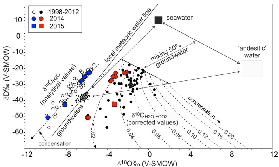
Figura 1.3.3 - Diagramma della composizione isotopica dell'ossigeno e dell'idrogeno dei vapori emessi dalle fumarole di fondo cratere del Vesuvio. I dati analitici (simboli blu e bianchi) possono essere interpretati considerando l'equilibrio isotopico dell'ossigeno tra il CO 2 e il vapore e gli effetti di condensazione in accordo con il modello proposto in Caliro et al. (2011), al quale si rimanda per maggiori dettagli e approfondimenti. Tale modello prevede un'origine del vapore fumarolico dovuta al mixing di tre componenti: acqua magmatica di tipo andesitico, acqua di mare e acque meteoriche locali. Le linee tratteggiate indicano le variazioni composizionali del sistema H 2 O+CO 2 legate a processi di condensazione del vapore per un fluido originato da differenti miscele delle tre componenti, la cui frazione molare di CO 2 è indicata su ogni linea. La composizione dei campioni calcolata per il sistema H 2 O+CO 2 (simboli
