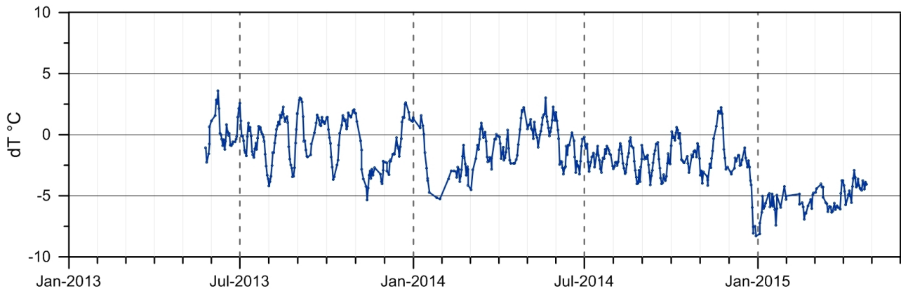
Figura 1.3.1 - Stazione Vesuvio. Medie settimanali dei residui (dT°; Vilardo et al., 2015) della serie temporale dei valori di temperatura massima rilevati nell'immagine IR.
