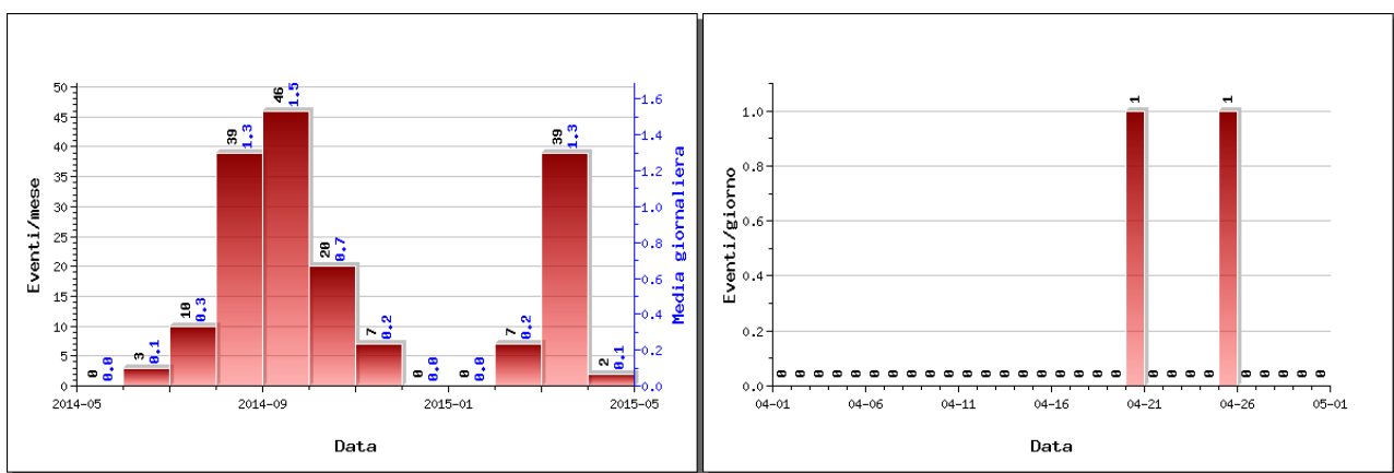
Figura 2.1.1 – A sinistra numero di eventi registrati ai Campi Flegrei nel corso degli ultimi 12 mesi (in totale 173), mentre a destra quelli avvenuti nell'ultimo mese (in totale 2).
