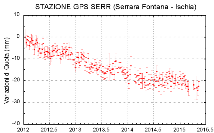
Figura 3.2.2 - Serie temporale delle variazioni settimanali in quota della stazione di SERR (Ischia) da gennaio 2012 a maggio 2015
