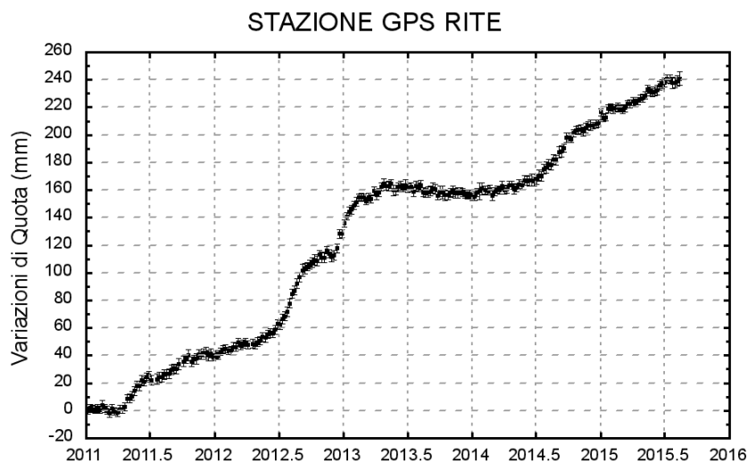
Figura 2.2.2 - Serie temporale delle variazioni settimanali in quota della stazione di RITE (Pozzuoli) dal 2011 ad agosto 2015.
