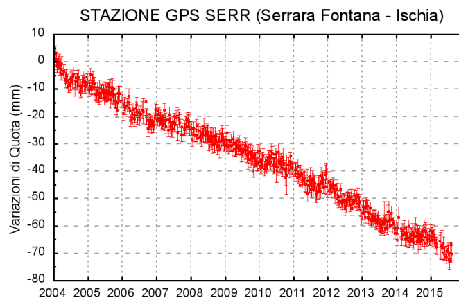
Figura 3.2.1: Serie temporale delle variazioni settimanali in quota della stazione di SERR (Ischia) dal 2004 ad agosto 2015.
