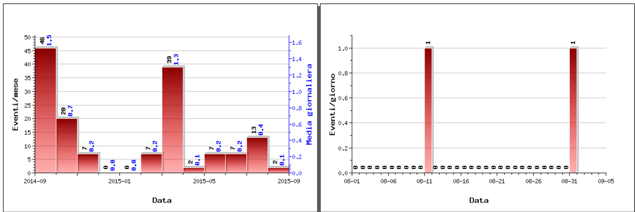
Figura 2.1.1 – A sinistra numero di eventi registrati ai Campi Flegrei nel corso degli ultimi 12 mesi (in totale 150), mentre a destra quelli avvenuti nell'ultimo mese (in totale 2).
