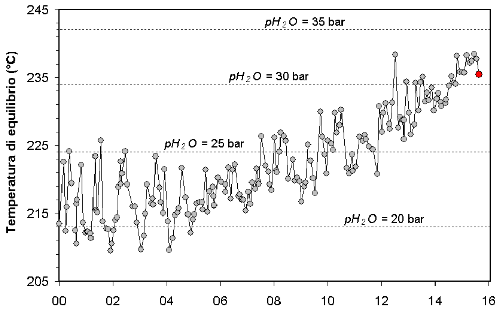
Fig. 2.3.3 – Cronogramma delle temperature di equilibrio per il sistema CO-CO 2 , stimate assumendo condizioni redox fissate dalla relazione di D'Amore and Panichi (1980). Tali temperature, rappresentative della parte più superficiale del sistema idrotermale (Caliro et al., 2007), mostrano un trend d'aumento a partire dai primi anni del 2000. In rosso è evidenziato il campione relativo al mese di Agosto 2015.
