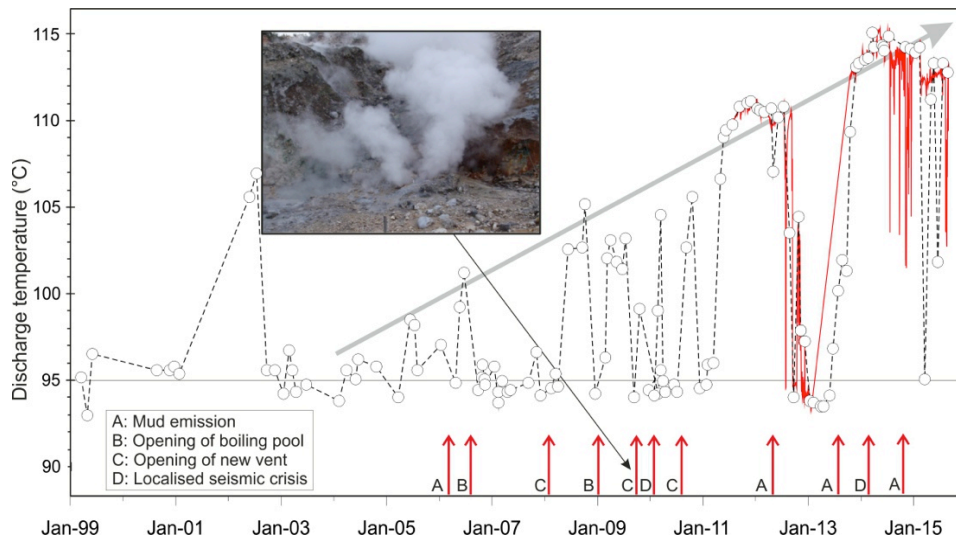
Fig. 2.3.6 - Cronogramma delle temperature ( ^{\circ}\text{C} ) della fumarola di Pisciarelli e dei maggiori eventi occorsi legati all'aumento dell'attività idrotermale (i cerchi si riferiscono a misure discrete riferite al punto di prelievo dei gas, la linea rossa si riferisce alle medie giornaliere delle misure in continuo). La temperatura di 95^{\circ}\text{C} rappresenta la temperatura di ebollizione per i fluidi fumarolici di Pisciarelli. Nella foto è riportata la nuova vigorosa fumarola sorta il 20 dicembre 2009.
