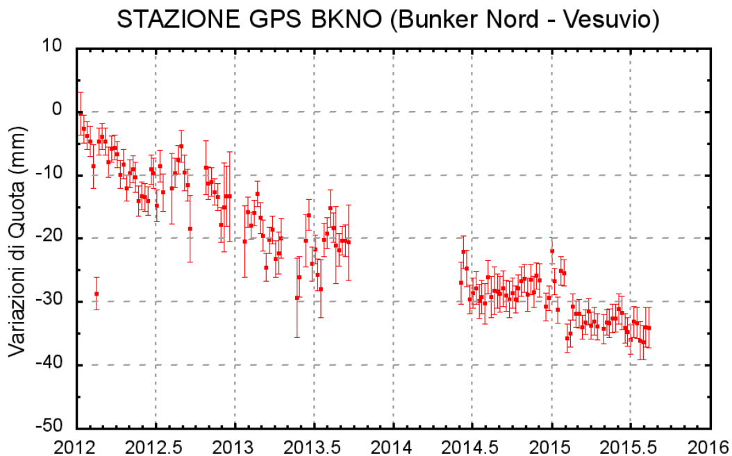
Figura 1.2.1 - Serie temporale delle variazioni settimanali in quota della stazione di BKNO (Vesuvio) da gennaio 2012 ad agosto 2015.
