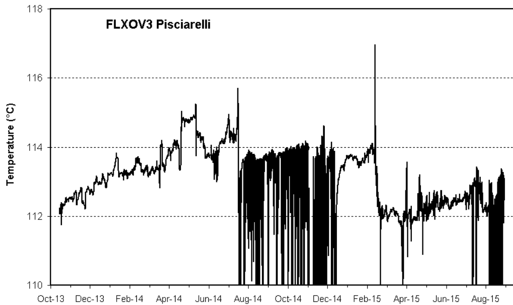
Fig. 2.3.7 - Temperature registrate in continuo della fumarola di Pisciarelli.
