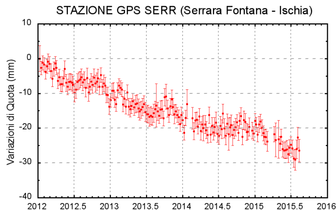
Figura 3.2.2: Serie temporale delle variazioni settimanali in quota della stazione di SERR (Ischia) da gennaio 2012 ad agosto 2015.
