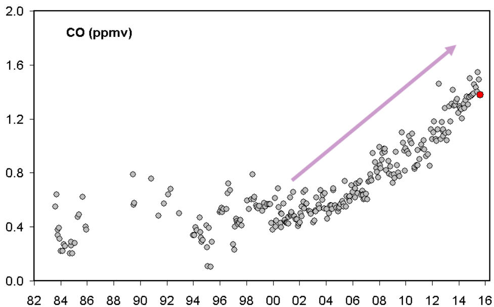
Fig. 2.3.2 - Variazioni della concentrazione di monossido di carbonio (CO) misurato alla fumarola BG a partire dal 1983. In rosso è evidenziato il campione relativo al mese di Agosto 2015. In generale alti contenuti di CO caratterizzano sistemi vulcanici ad elevata temperatura mentre fumarole alimentate da sistemi idrotermali mostrano concentrazioni più basse, in tali sistemi un aumento delle concentrazioni di CO può riflettere un incremento delle condizioni di pressione e temperatura.
