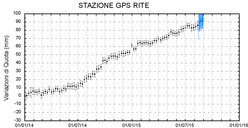
Figura 2.2.3 - Serie temporale delle variazioni in quota della stazione di RITE (Pozzuoli) dal 01 gennaio 2014 al 31 agosto 2015.
