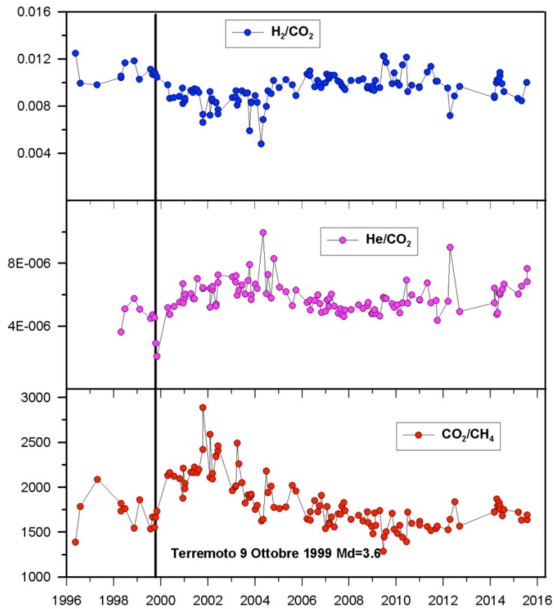
Figura 1.4.1 - Variazioni composizionali della fumarola FC2 nel periodo 1996-2015.
