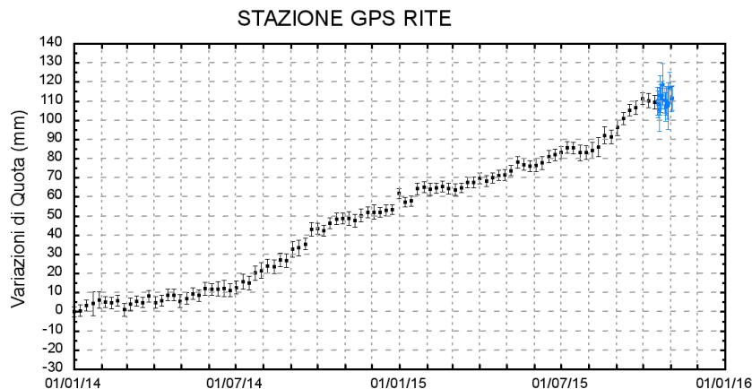
Figura 2.2.3 - Serie temporale delle variazioni in quota della stazione di RITE (Pozzuoli) dal 01 gennaio 2014 al 03 novembre 2015.
