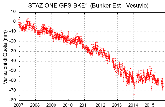
Figura 1.2.1 - Serie temporale delle variazioni settimanali in quota della stazione di BKE1 (Vesuvio) dal 2007 ad ottobre 2015.
