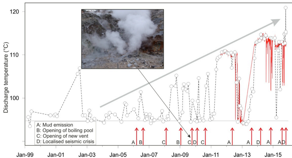
Fig. 2.3.6 - Cronogramma delle temperature ( ^{\circ}\text{C} ) della fumarola di Pisciarelli e dei maggiori eventi occorsi legati all'aumento dell'attività idrotermale (i cerchi si riferiscono a misure discrete riferite al punto di prelievo dei gas, la linea rossa si riferisce alle medie giornaliere delle misure in continuo). La temperatura di \sim 95^{\circ}\text{C} rappresenta la temperatura di ebollizione per i fluidi fumarolici di Pisciarelli. Nella foto è riportata la nuova vigorosa fumarola sorta il 20 dicembre 2009.
