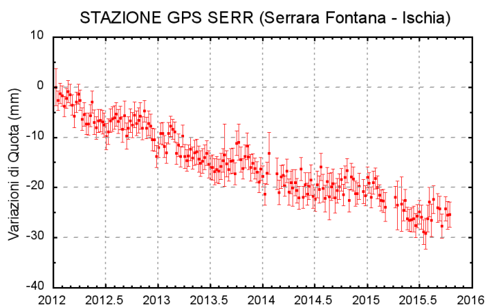
Figura 3.2.2 - Serie temporale delle variazioni settimanali in quota della stazione di SERR (Ischia) da gennaio 2012 ad ottobre 2015.
