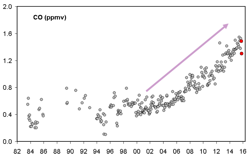
Fig. 2.3.2 - Variazioni della concentrazione di monossido di carbonio (CO) misurato alla fumarola BG a partire dal 1983. In rosso sono evidenziati i campioni di Ottobre 2015. In generale alti contenuti di CO caratterizzano sistemi vulcanici ad elevata temperatura mentre fumarole alimentate da sistemi idrotermali mostrano concentrazioni più basse, in tali sistemi un aumento delle concentrazioni di CO può riflettere un incremento delle condizioni di pressione e temperatura.
