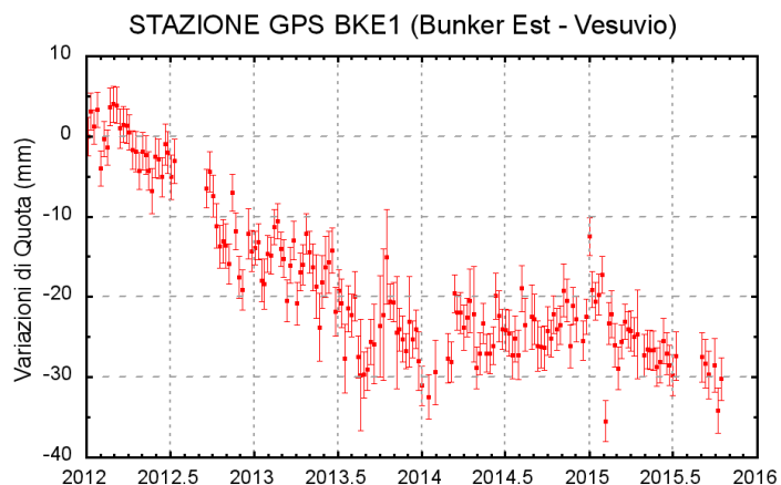
Figura 1.2.2 - Serie temporale delle variazioni settimanali in quota della stazione di BKE1 (Vesuvio) da gennaio 2012 ad ottobre 2015.
