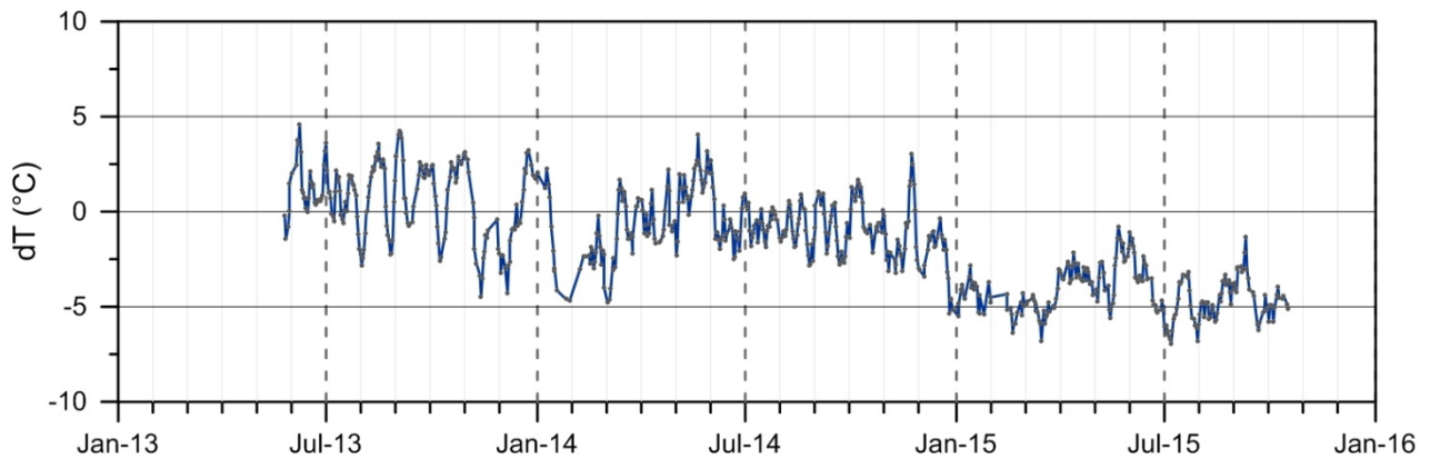
Figura 1.3.1 - Stazione Vesuvio. Medie settimanali dei residui ( dT^{\circ} ; Vilaro et al., 2015) della serie temporale dei valori di temperatura massima rilevati nell'immagine IR.
