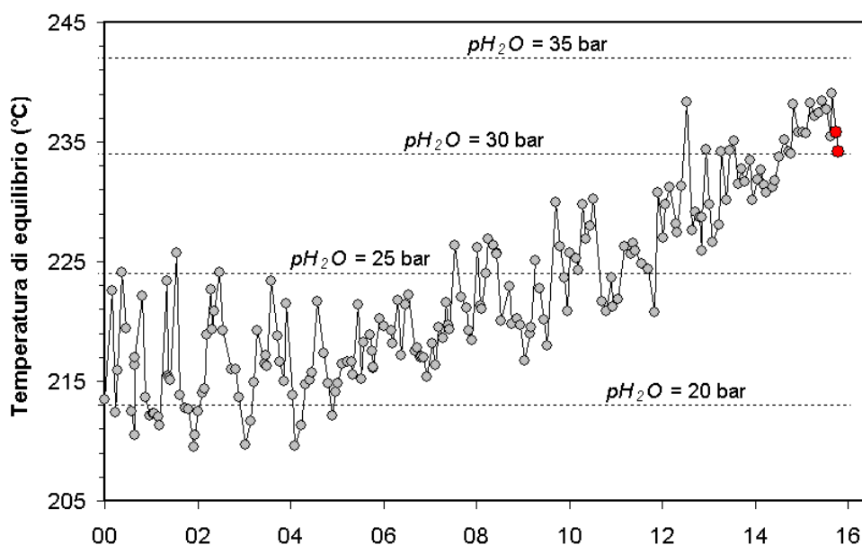
Fig. 2.3.3 – Cronogramma delle temperature di equilibrio per il sistema CO-CO_2 , stimate assumendo condizioni redox fissate dalla relazione di D'Amore and Panichi (1980). Tali temperature, rappresentative della parte più superficiale del sistema idrotermale (Caliro et al., 2007), mostrano un trend d'aumento a partire dai primi anni del 2000. In rosso sono evidenziati i campioni di Ottobre 2015.
