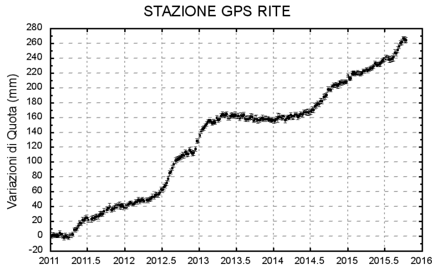
Figura 2.2.2 - Serie temporale delle variazioni settimanali in quota della stazione di RITE (Pozzuoli) dal 2011 ad ottobre 2015.
