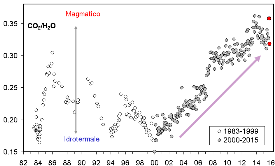
Fig. 2.3.1 - Cronogramma del rapporto CO_2/H_2O per la fumarola BG. In grigio sono riportati i dati a partire dal 2000, quando è iniziato un trend d'aumento del rapporto CO_2/H_2O , in generale, indicativo di una crescente frazione della componente magmatica nei fluidi fumarolici. In rosso sono evidenziati i campioni di Ottobre 2015.
