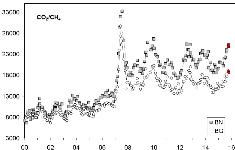
Fig. 2.3.4 – Variazioni del rapporto CO_2/CH_4 per le fumarole BG e BN a partire dal 2000. I picchi nel rapporto, registrati in superficie con circa un anno di ritardo, evidenziano episodi di degassamento magmatico occorsi ai Campi Flegrei (Chiodini et al., 2012). In rosso sono evidenziati i valori relativi ai campioni di Ottobre 2015.
