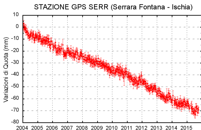
Figura 3.2.1 - Serie temporale delle variazioni settimanali in quota della stazione di SERR (Ischia) dal 2004 ad ottobre 2015.
