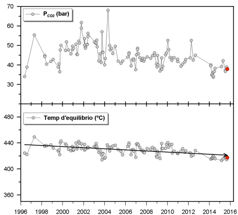
Figura 1.4.2 - Cronogramma dei valori d'equilibrio della temperatura e pressione parziale di CO_2 stimati per il sistema idrotermale del Vesuvio. Il campione di Ottobre 2015 è riportato con il simbolo rosso.
