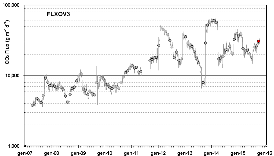
Fig. 2.3.8 - Medie giornaliere (linea) e medie mensili (cerchi) dei flussi di CO_2 misurati a Pisciarelli (FLXOV3). E' da evidenziare il continuo trend d'aumento nel tempo del flusso CO_2 . La media dei flussi relativa al mese di Ottobre è riportata con il simbolo rosso.
