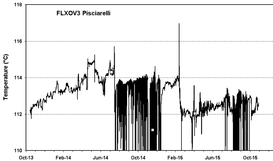
Fig. 2.3.7 - Temperature registrate in continuo della fumarola di Pisciarelli. Le temperature sono lievemente più basse delle temperature massime misurate poiché attualmente il sensore di temperatura, a causa del continuo allargamento della bocca di emissione, non è più posizionato nel punto di massimo flusso.
