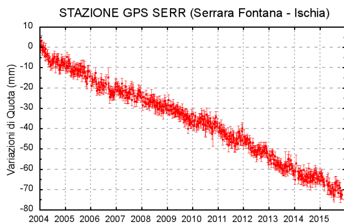
Figura 3.2.1 - Serie temporale delle variazioni settimanali in quota della stazione di SERR (Ischia) dal 2004 a novembre 2015.
