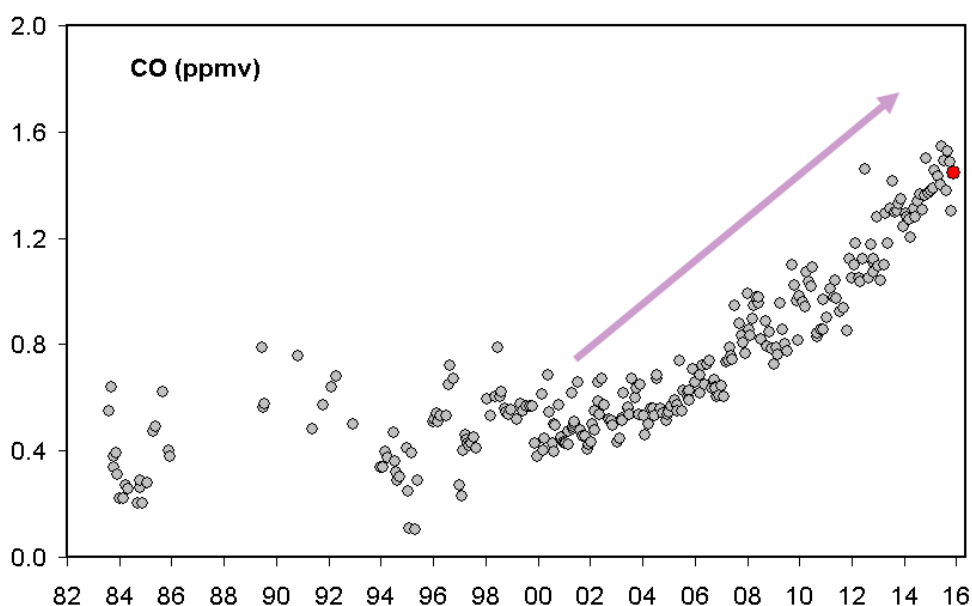
Figura 2.3.2 - Variazioni della concentrazione di monossido di carbonio (CO) misurato alla fumarola BG a partire dal 1983. Con il simbolo rosso è evidenziato il campione di Novembre 2015. In generale alti contenuti di CO caratterizzano sistemi vulcanici ad elevata temperatura mentre fumarole alimentate da sistemi idrotermali mostrano concentrazioni più basse, in tali sistemi un aumento delle concentrazioni di CO può riflettere un incremento delle condizioni di pressione e temperatura.
