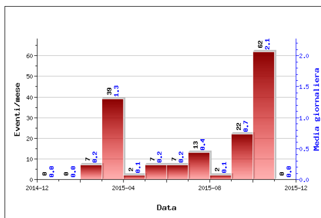
Figura 2.1.1 - Numero di eventi registrati ai Campi Flegrei nel corso degli ultimi 12 mesi (in totale 161).
