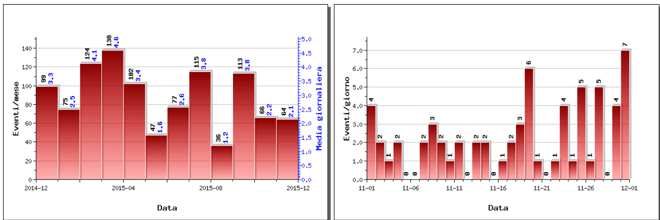
Figura 1.1.1 – A sinistra il numero di eventi registrati al Vesuvio nel corso degli ultimi 12 mesi (in totale 1056), mentre a destra quelli avvenuti nell'ultimo mese (in totale 64).
