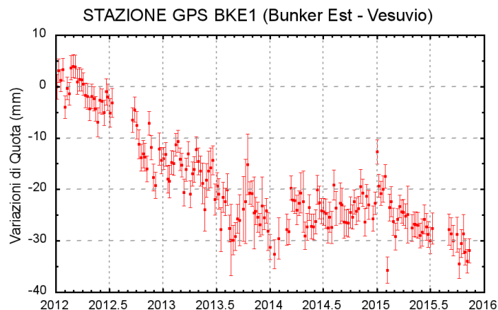
Figura 1.2.2 - Serie temporale delle variazioni settimanali in quota della stazione di BKE1 (Vesuvio) da gennaio 2012 a novembre 2015.
