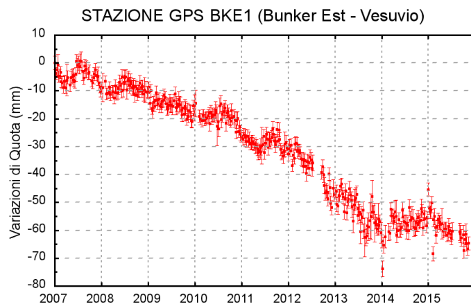
Figura 1.2.1 - Serie temporale delle variazioni settimanali in quota della stazione di BKE1 (Vesuvio) dal 2007 a novembre 2015.
