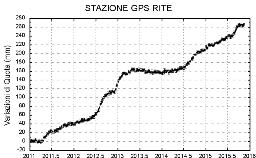
Figura 2.2.2 - Serie temporale delle variazioni settimanali in quota della stazione di RITE (Pozzuoli) dal 2011 a novembre 2015.
