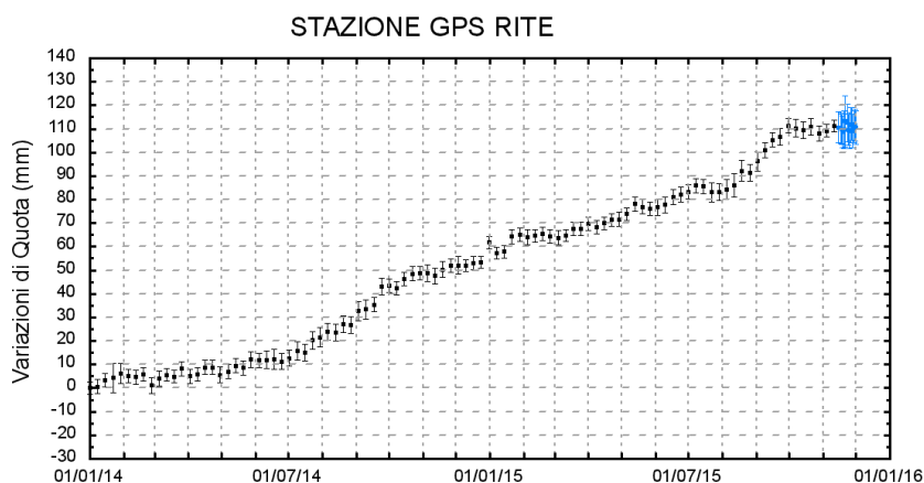
Figura 2.2.3 - Serie temporale delle variazioni in quota della stazione di RITE (Pozzuoli) dal 01 gennaio 2014 al 01 dicembre 2015.
