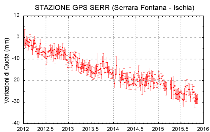
Figura 3.2.2 - Serie temporale delle variazioni settimanali in quota della stazione di SERR (Ischia) da gennaio 2012 a novembre 2015.
