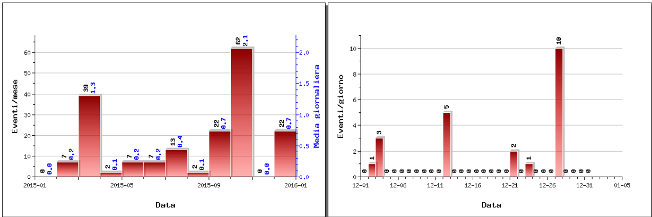
Figura 2.1.1 – A sinistra numero di eventi registrati ai Campi Flegrei nel corso degli ultimi 12 mesi (in totale 183), mentre a destra quelli avvenuti nell'ultimo mese (in totale 22).
