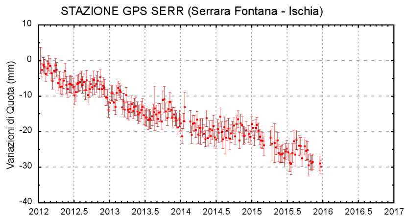
Figura 3.2.2 - Serie temporale delle variazioni settimanali in quota della stazione di SERR (Ischia) da gennaio 2012 a dicembre 2015.
