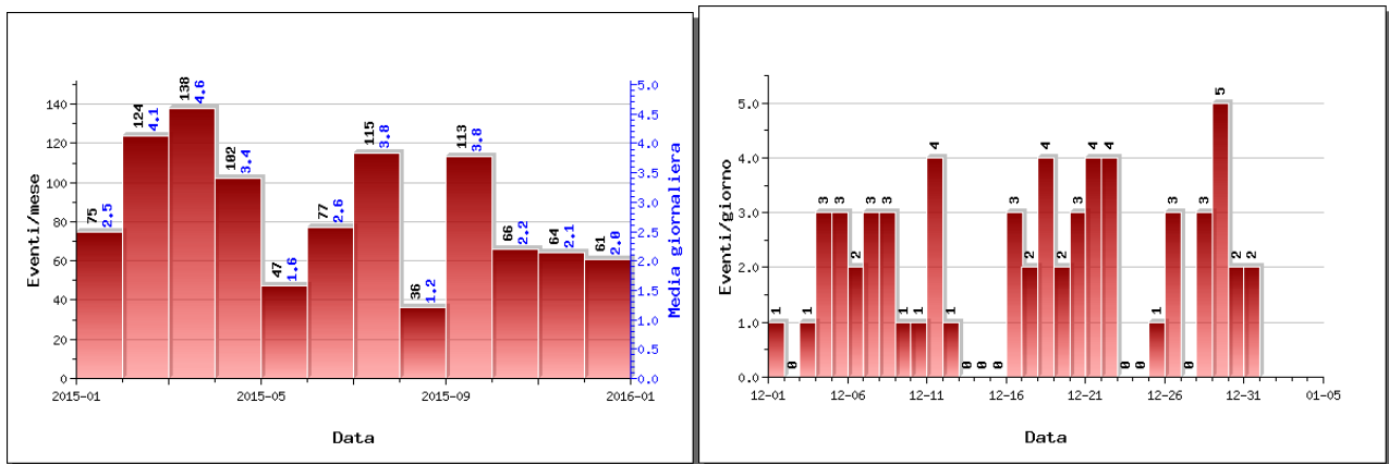
Figura 1.1.1 – A sinistra il numero di eventi registrati al Vesuvio nel corso degli ultimi 12 mesi (in totale 1018), mentre a destra quelli avvenuti nell'ultimo mese (in totale 61).
