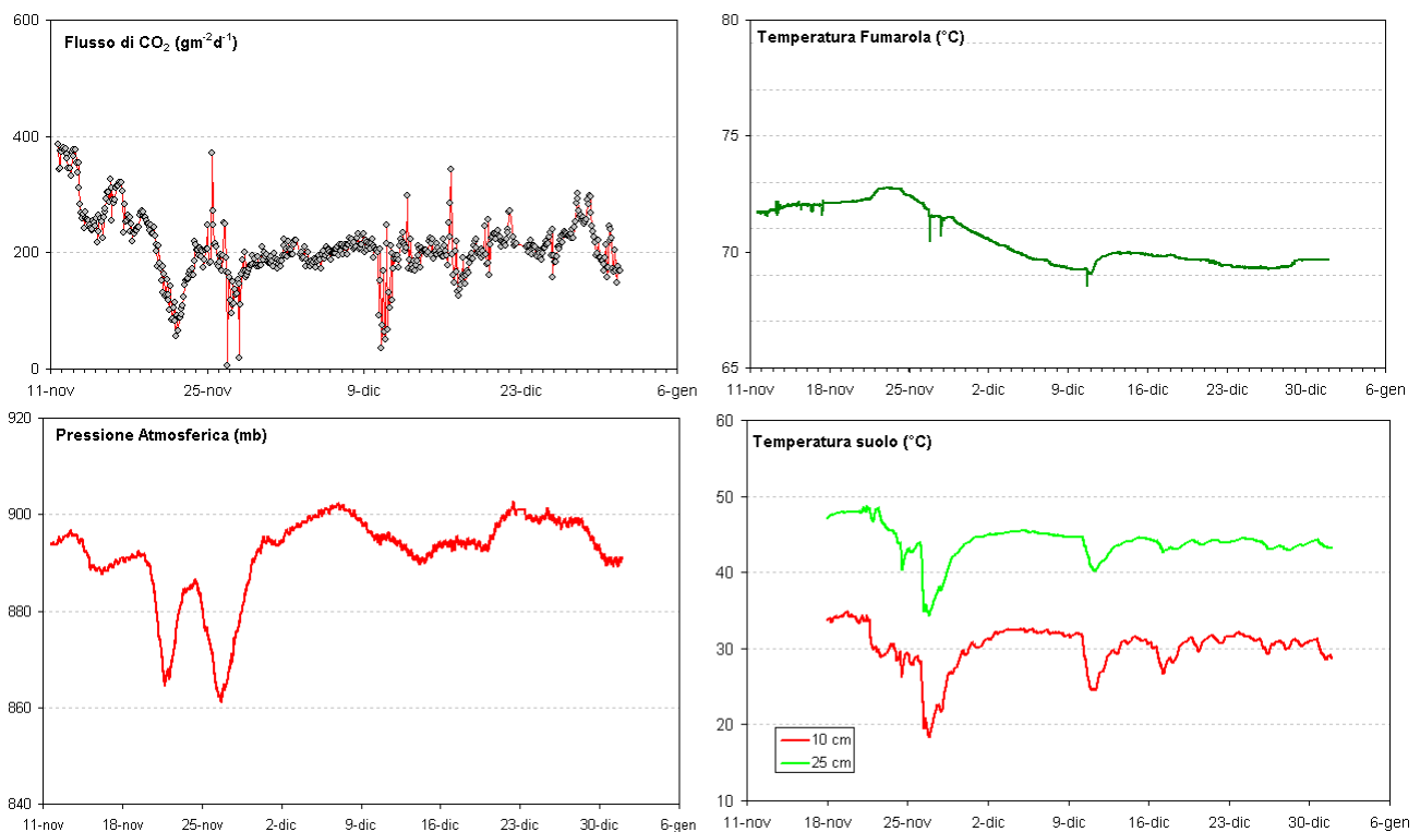
Figura 1.4.4 - Parametri misurati dalla stazione geochimica installata in area bordo cratere del Vesuvio (settoe SW).
