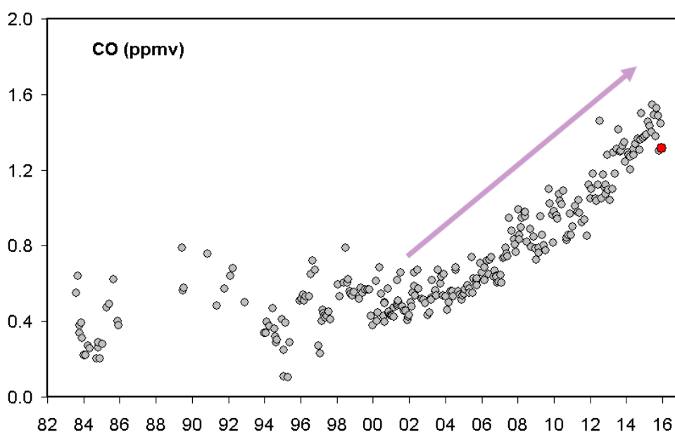
Figura 2.3.2 - Variazioni della concentrazione di monossido di carbonio (CO) misurato alla fumarola BG a partire dal 1983. Con il simbolo rosso è evidenziato il campione di Dicembre 2015. In generale alti contenuti di CO caratterizzano sistemi vulcanici ad elevata temperatura mentre fumarole alimentate da sistemi idrotermali mostrano concentrazioni più basse, in tali sistemi un aumento delle concentrazioni di CO può riflettere un incremento delle condizioni di pressione e temperatura.
