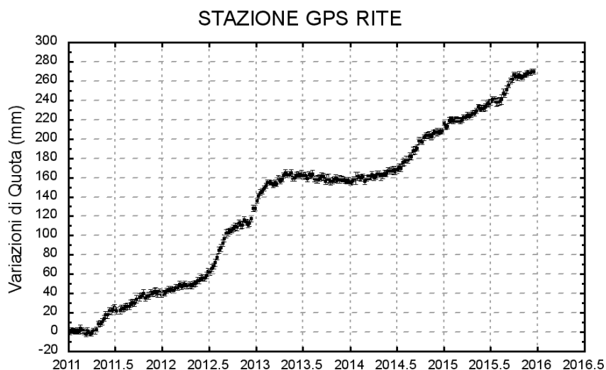
Figura 2.2.2 - Serie temporale delle variazioni settimanali in quota della stazione di RITE (Pozzuoli) dal 2011 a dicembre 2015.
