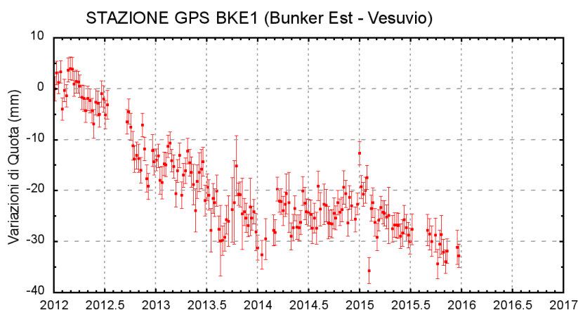
Figura 1.2.2 - Serie temporale delle variazioni settimanali in quota della stazione di BKE1 (Vesuvio) da gennaio 2012 a dicembre 2015.
