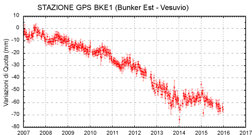
Figura 1.2.1 - Serie temporale delle variazioni settimanali in quota della stazione di BKE1 (Vesuvio) dal 2007 a dicembre 2015.
