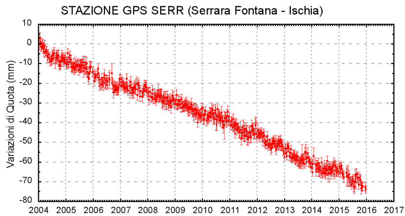
Figura 3.2.1 - Serie temporale delle variazioni settimanali in quota della stazione di SERR (Ischia) dal 2004 a dicembre 2015.
