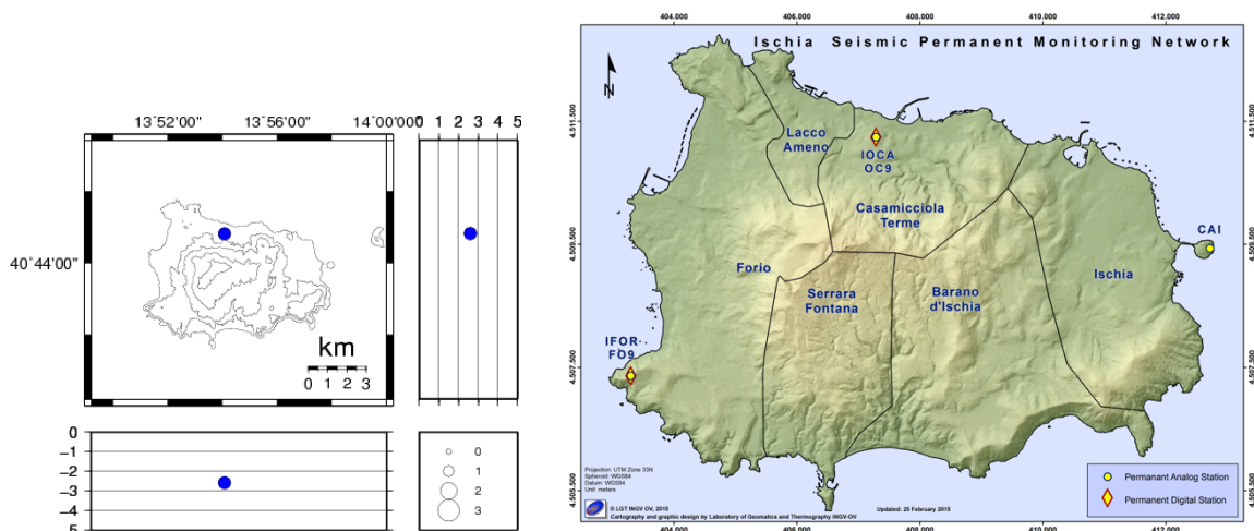
Figura 3.1.2 – Localizzazioni ipocentrali ad Ischia nel corso degli ultimi 12 mesi. La dimensione dei simboli è proporzionale alla magnitudo, come indicato nel riquadro in basso. A destra è mostrata la mappa con la rete sismica di Ischia.
