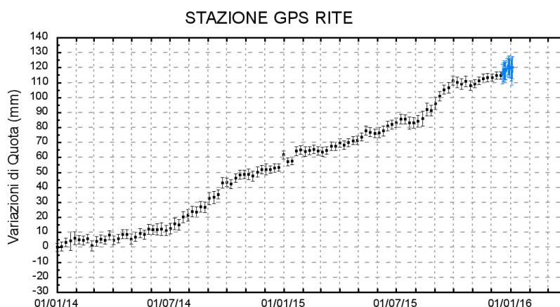
Figura 2.2.3 - Serie temporale delle variazioni in quota della stazione di RITE (Pozzuoli) dal 01 gennaio 2014 al 04 gennaio 2016.
