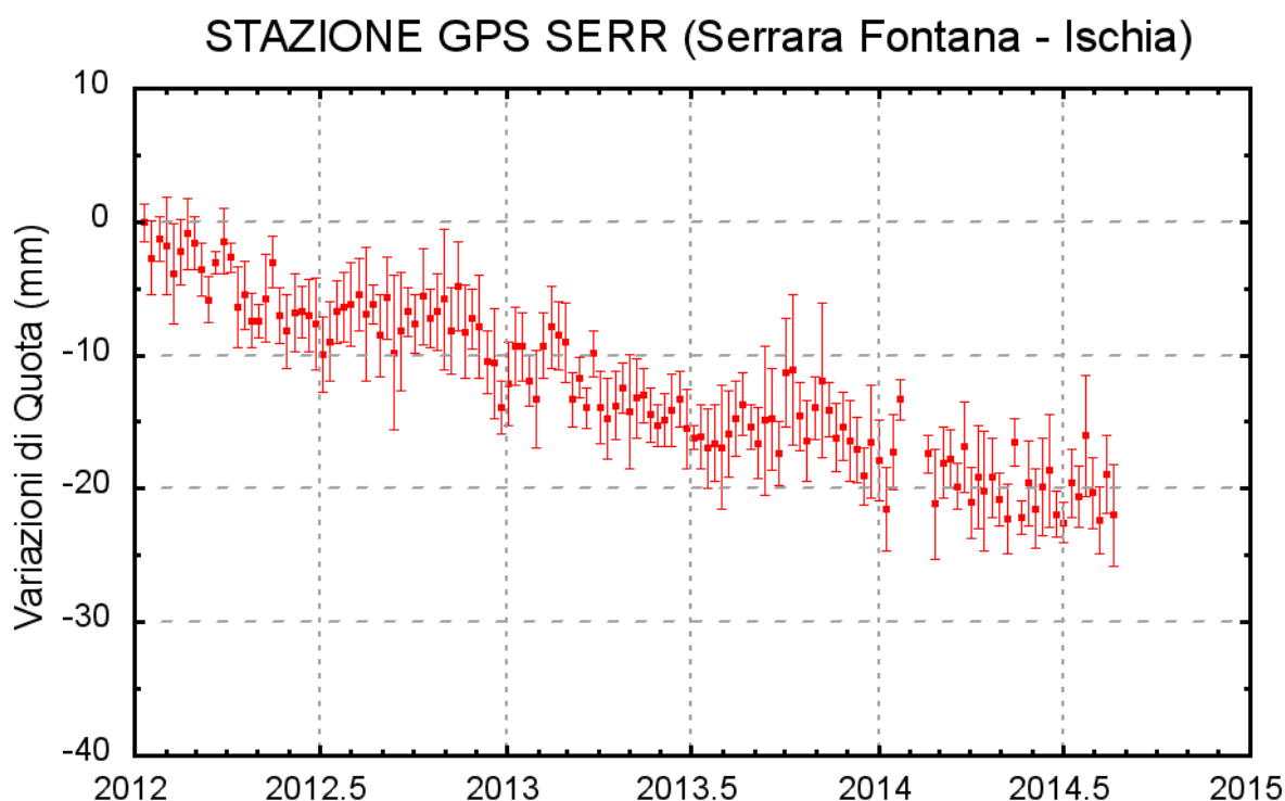
Figura 3.2.2 - Serie temporale delle variazioni settimanali in quota della stazione di SERR (Ischia) dal 01 gennaio 2012 al 31 agosto 2014
