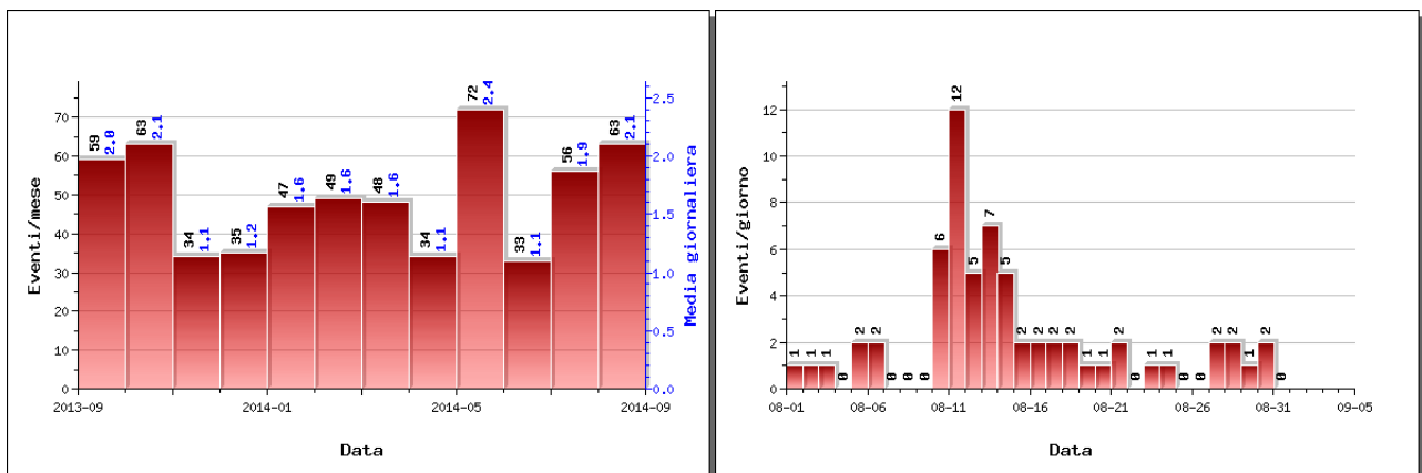
Figura 1.1.1 – A sinistra il numero di eventi registrati al Vesuvio nel corso degli ultimi 12 mesi (in totale 593), mentre a destra quelli avvenuti nell'ultimo mese (in totale 63).
