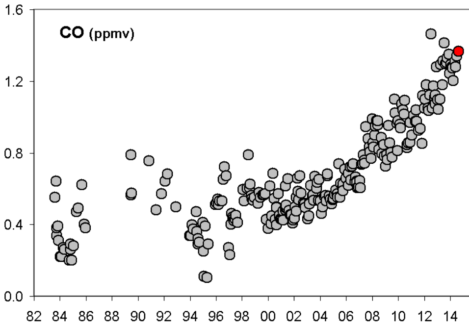
Fig. 2.3.3 – Variazioni della concentrazione di monossido di carbonio (CO) misurato alla fumarola BG a partire dal 1983. In rosso è evidenziato il campione relativo al mese di Agosto 2014. In generale alti contenuti di CO caratterizzano sistemi vulcanici ad elevata temperatura mentre fumarole alimentate da sistemi idrotermali mostrano concentrazioni più basse, in tali sistemi un aumento delle concentrazioni di CO può riflettere un incremento delle condizioni di pressione e temperatura.
