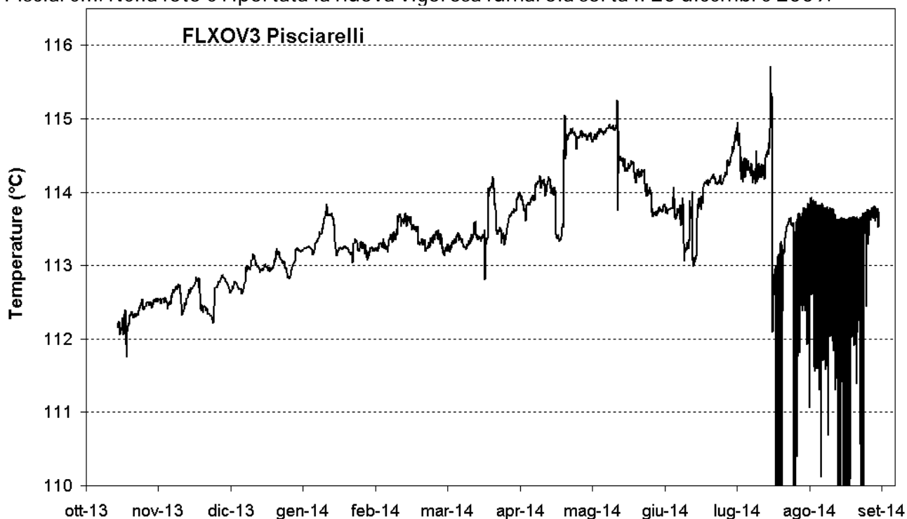
Figura 2.3.7 - Dettaglio delle temperature registrate in continuo della fumarola di Pisciarelli. È da evidenziare il continuo trend d'aumento della temperatura che a Luglio ha superato i 115.7 °C.
