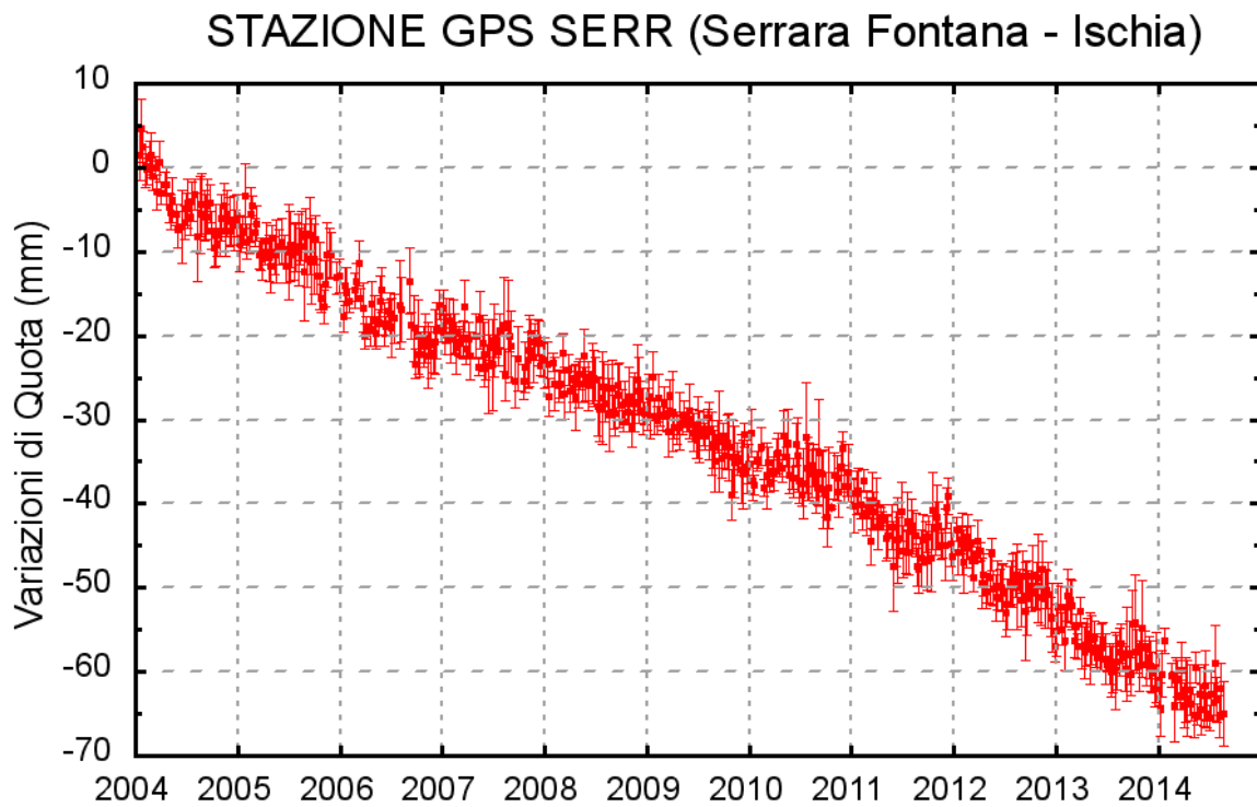
Figura 3.2.1 - Serie temporale delle variazioni settimanali in quota della stazione di SERR (Ischia) dal 2004 al 31 agosto 2014
