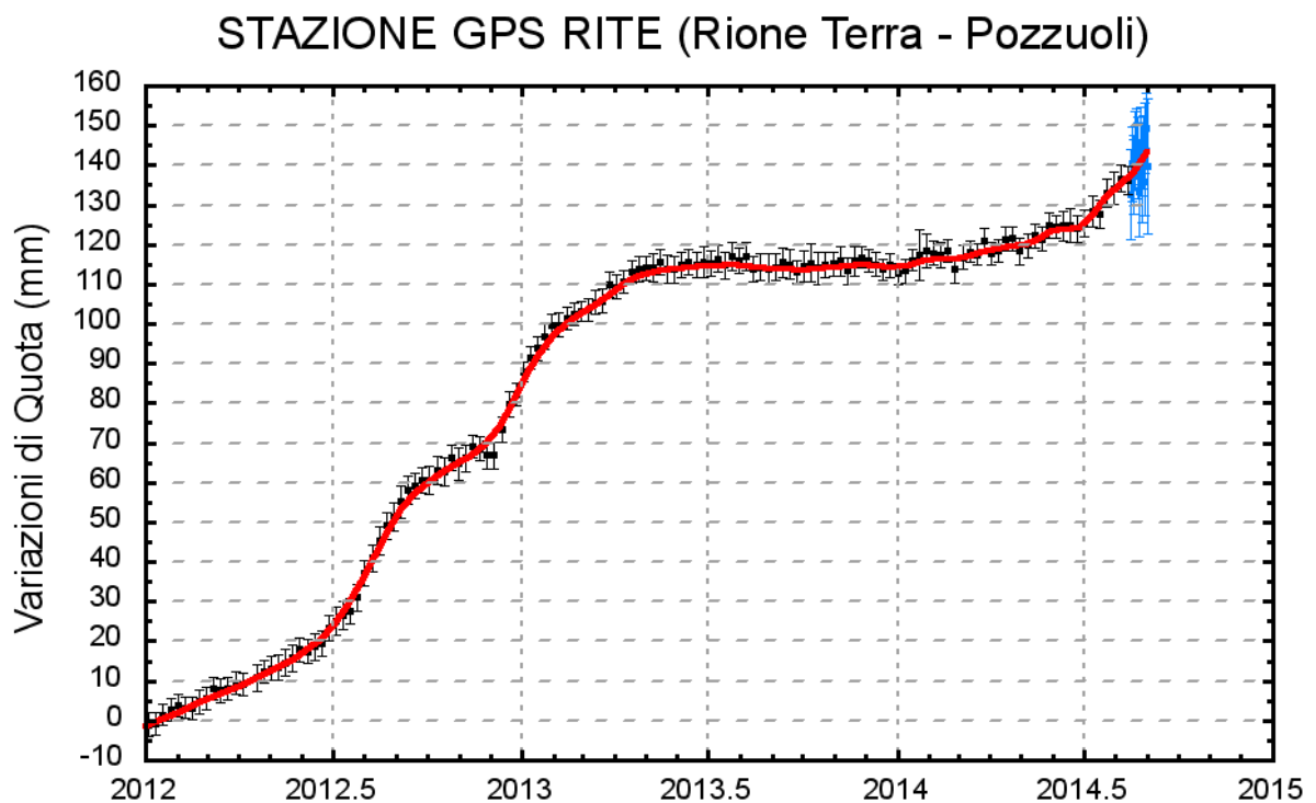
Figura 2.2.2 - Serie temporale delle variazioni in quota della stazione di RITE (Pozzuoli) dal 01 gennaio 2012 al 01 settembre 2014
