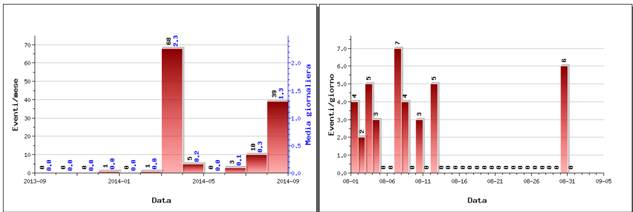
Figura 2.1.1 – A sinistra il numero di eventi registrati ai Campi Flegrei nel corso degli ultimi 12 mesi (in totale 127), mentre a destra quelli avvenuti nell'ultimo mese (in totale 39).
