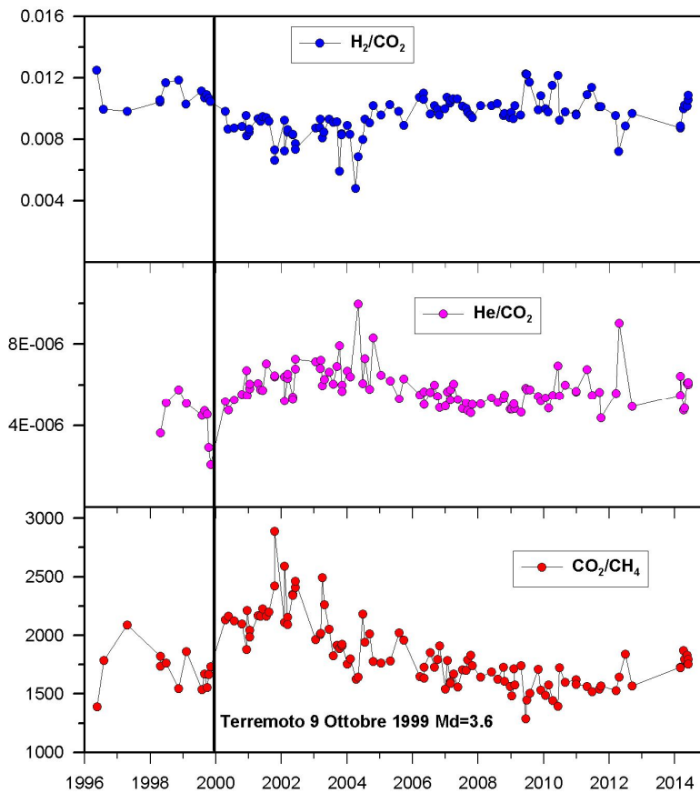
Figura 1.3.1 - Variazioni composizionali della fumarola FC2 nel periodo 1996-2014.
