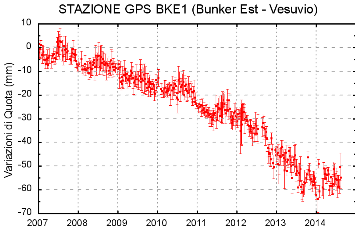
Figura 1.2.1 - Serie temporale delle variazioni settimanali in quota della stazione di BKE1 (Vesuvio) dal 2007 al 31 agosto 2014
