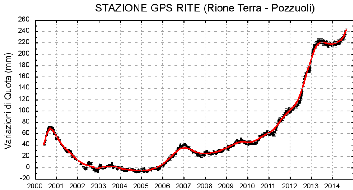
Figura 2.2.1 - Serie temporale delle variazioni settimanali in quota della stazione di RITE (Pozzuoli) dal 2000 al 31 agosto 2014
