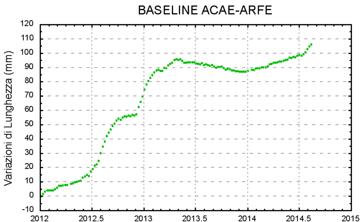
Figura 2.2.3 - Serie temporale delle variazioni in lunghezza della baseline ACAE (Accademia Aeronautica) – ARFE (Arcofelice) dal 01 gennaio 2012 al 23 agosto 2014.
