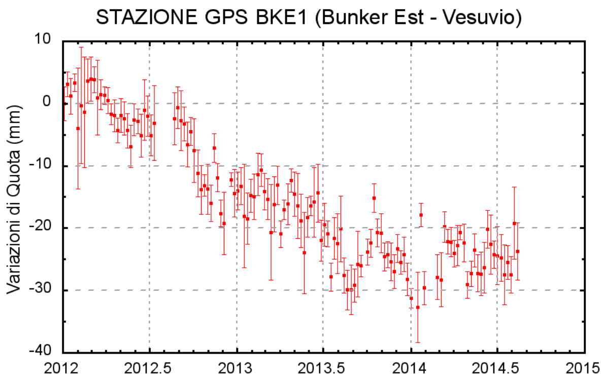
Figura 1.2.2 - Serie temporale delle variazioni settimanali in quota della stazione di BKE1 (Vesuvio) dal 01 gennaio 2012 al 31 agosto 2014
