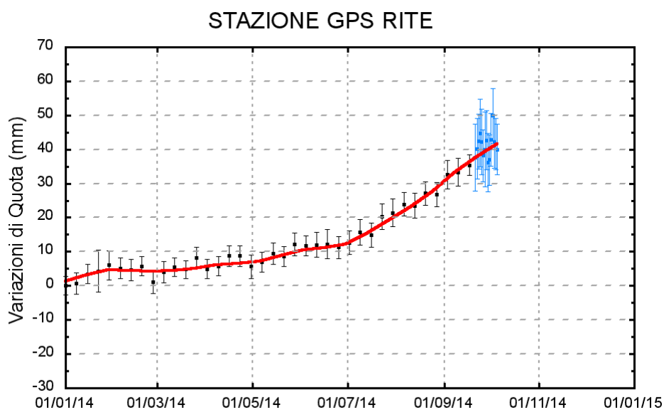
Figura 2.2.2 - Serie temporale delle variazioni in quota della stazione di RITE (Pozzuoli) dal 01 gennaio 2012 al 05 ottobre 2014 (vedi bollettino settimanale)
