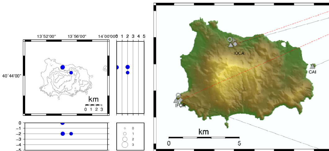
Figura 3.1.2 – Localizzazione ipocentrale degli eventi localizzati ad Ischia nel corso degli ultimi 12 mesi. La dimensione del simbolo è proporzionale alla magnitudo, come indicato nel riquadro in basso. A destra è mostrata la mappa con la rete sismica di Ischia.
