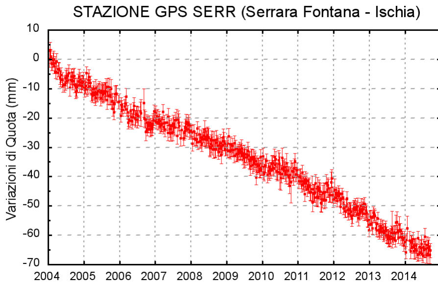
Figura 3.2.1 - Serie temporale delle variazioni settimanali in quota della stazione di SERR (Ischia) dal 2004 a settembre 2014
