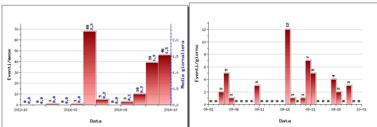
Figura 2.1.1 – A sinistra il numero di eventi registrati ai Campi Flegrei nel corso degli ultimi 12 mesi (in totale 173), mentre a destra quelli avvenuti nell'ultimo mese (in totale 46).
