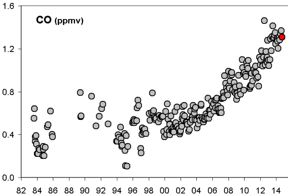
Figura 2.3.3 – Variazioni della concentrazione di monossido di carbonio (CO) misurato alla fumarola BG a partire dal 1983. In rosso è evidenziato il campione relativo al mese di Settembre 2014. In generale alti contenuti di CO caratterizzano sistemi vulcanici ad elevata temperatura mentre fumarole alimentate da sistemi idrotermali mostrano concentrazioni più basse, in tali sistemi un aumento delle concentrazioni di CO può riflettere un incremento delle condizioni di pressione e temperatura.
