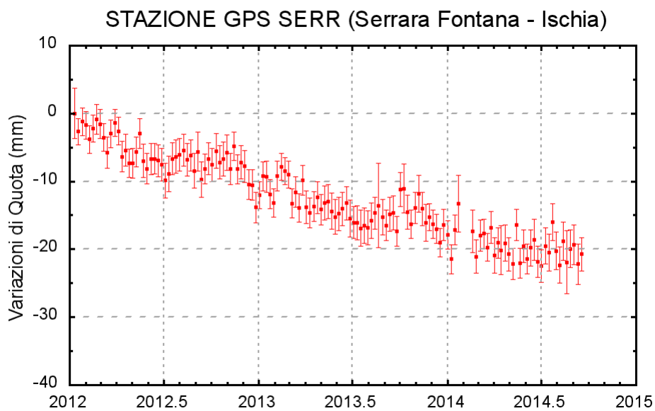
Figura 3.2.2 - Serie temporale delle variazioni settimanali in quota della stazione di SERR (Ischia) da gennaio 2012 a settembre 2014
