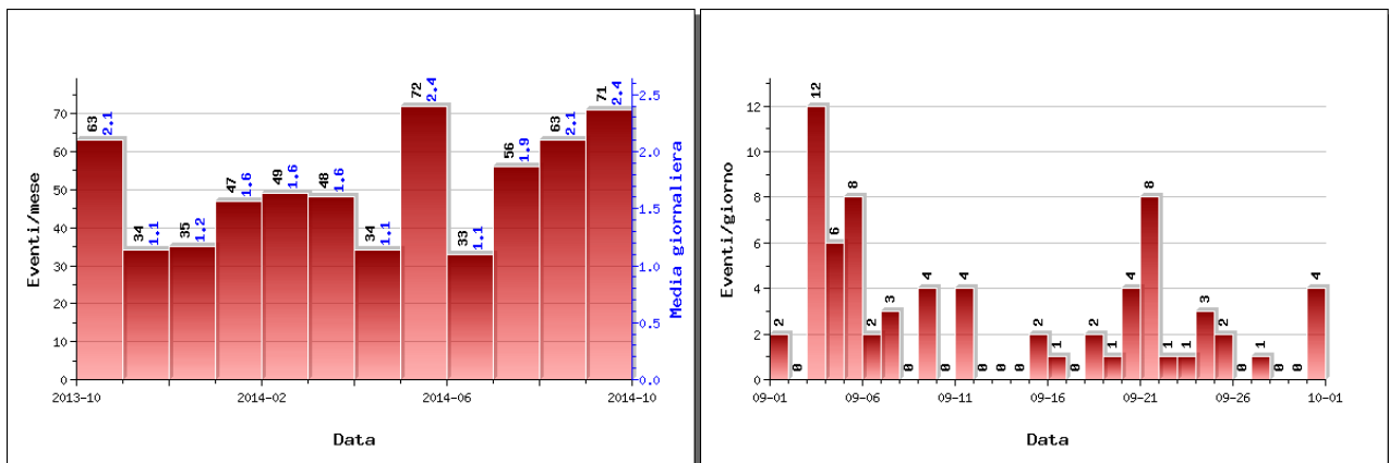
Figura 1.1.1 – A sinistra il numero di eventi registrati al Vesuvio nel corso degli ultimi 12 mesi (in totale 605), mentre a destra quelli avvenuti nell'ultimo mese (in totale 71).
