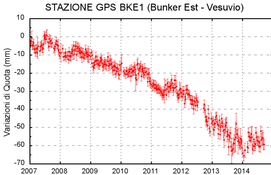
Figura 1.2.1 - Serie temporale delle variazioni settimanali in quota della stazione di BKE1 (Vesuvio) dal 2007 a settembre 2014
