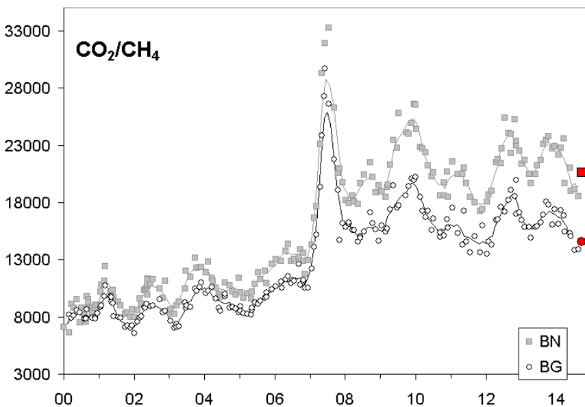
Figure 2.3.4 – Variazioni del rapporto CO 2 /CH 4 per le fumarole BG e BN a partire dal 2000. I picchi nel rapporto, registrati in superficie con circa un anno di ritardo, evidenziano episodi di degassamento magmatico occorsi ai Campi Flegrei (Chiodini et al., 2012). In rosso sono evidenziati i valori relativi ai campioni di Settembre 2014.
