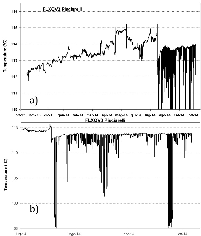
Figura 2.3.7 - Temperature registrate in continuo della fumarola di Pisciarelli. a) È da evidenziare il continuo trend d'aumento della temperatura che a Luglio ha superato i 115.7 °C. b) Dettaglio delle temperature da Luglio, le oscillazioni della temperatura, ed in particolare quelle fino alla temperatura di ebollizione (~95 °C), possono indicare i momenti di emissione dalla fumarola di una fase liquida.
