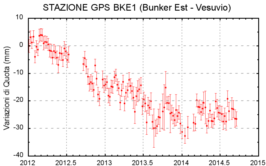
Figura 1.2.2 - Serie temporale delle variazioni settimanali in quota della stazione di BKE1 (Vesuvio) da gennaio 2012 a settembre 2014
