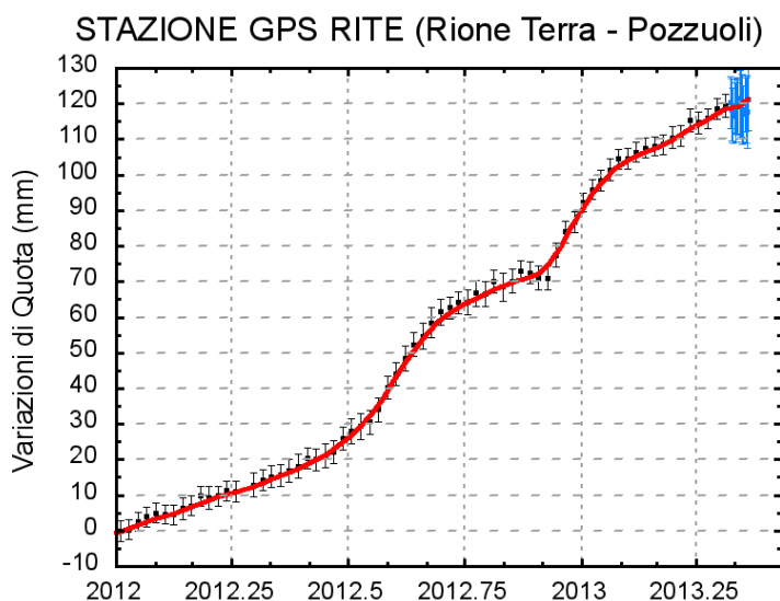
Fig. 2.2.2: Serie temporale delle variazioni in quota della stazione di RITE (Pozzuoli) dal 01 gennaio 2012 al 12 maggio 2013 (vedi bollettino settimanale)
