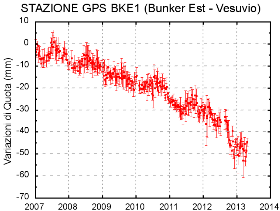
Fig. 1.2.1: Serie temporale delle variazioni settimanali in quota della stazione di BKE1 (Vesuvio) dal 2007 al 30 aprile 2013
