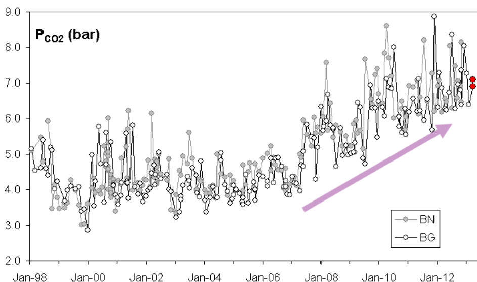
Fig 2.3.1 -Cronogramma della pressione di CO 2 d'equilibrio stimata nel sistema H 2 O-CO 2 -H 2 -CO per le fumarole BG e BN. In rosso sono evidenziati i dati relativi agli ultimi campioni analizzati (marzo 2013).
