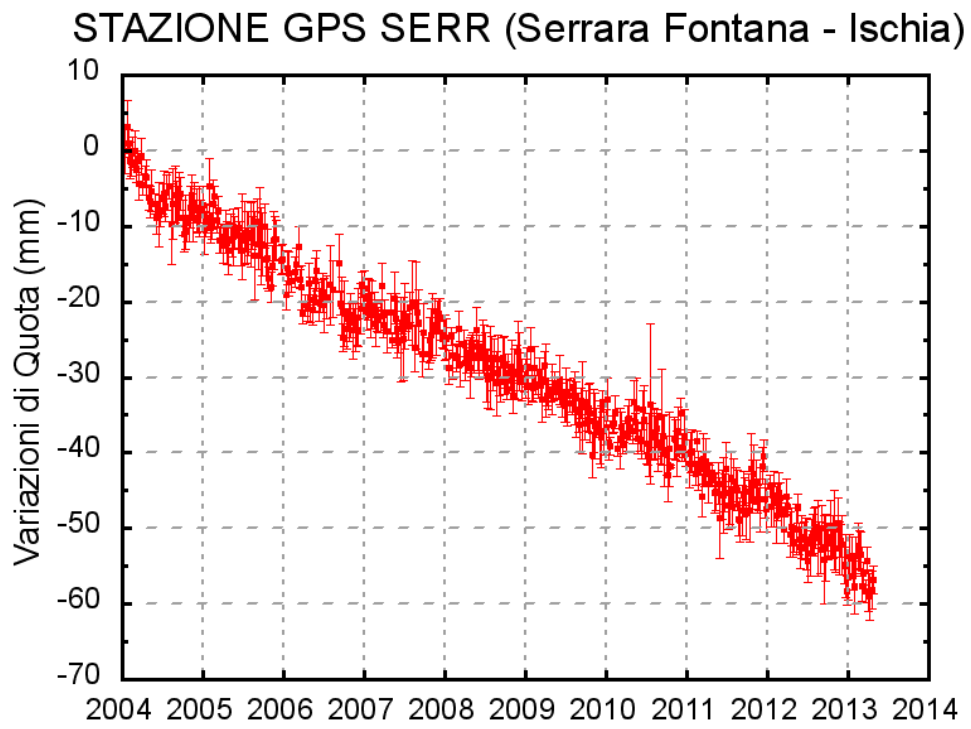
Fig. 3.2.1: Serie temporale delle variazioni settimanali in quota della stazione di SERR (Ischia) dal 2004 al 30 aprile 2013
