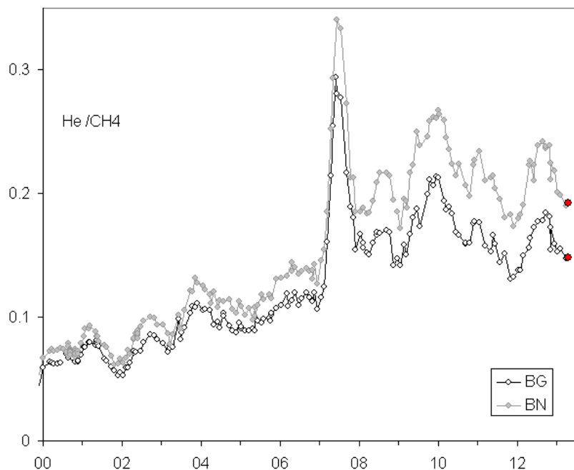
Fig. 2.3.3 – Variazioni del rapporto \text{He}/\text{CH}_4 per le fumarole BG e BN a partire dal 2000. I picchi nel rapporto, registrati in superficie con circa un anno di ritardo, evidenziano episodi di degassamento magmatico occorsi ai Campi Flegrei (Chiodini et al., 2012). In rosso sono evidenziati i valori relativi all'ultimo campione analizzato (Aprile 2013).
