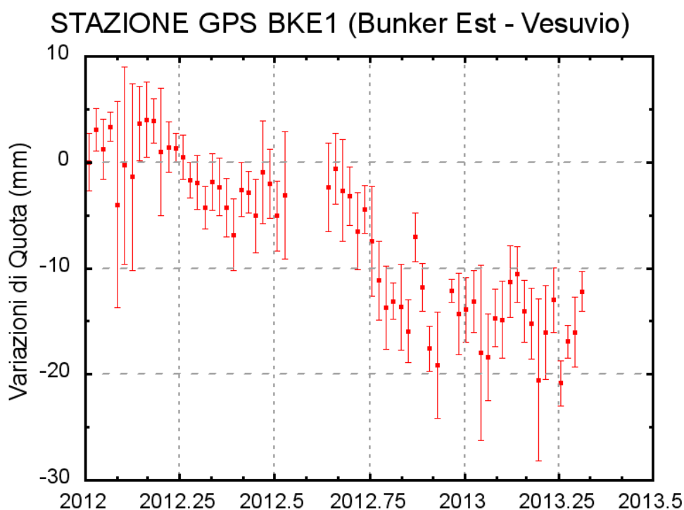
Fig. 1.2.2: Serie temporale delle variazioni settimanali in quota della stazione di BKE1 (Vesuvio) dal 01 gennaio 2012 al 30 aprile 2013
