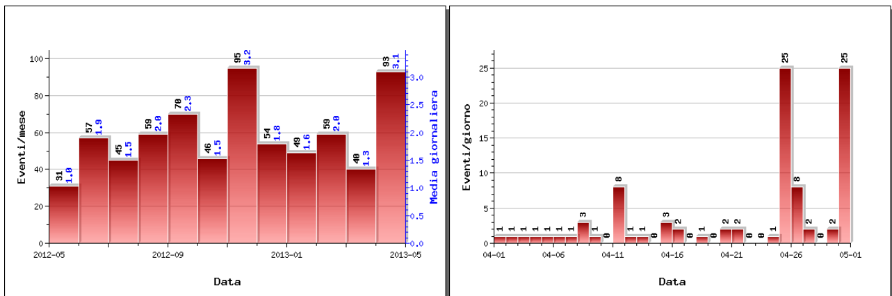
Figura 1.1.1 – A sinistra il numero di eventi registrati al Vesuvio nel corso degli ultimi 12 mesi (in totale 698), mentre a destra quelli avvenuti nell'ultimo mese (in totale 93).
