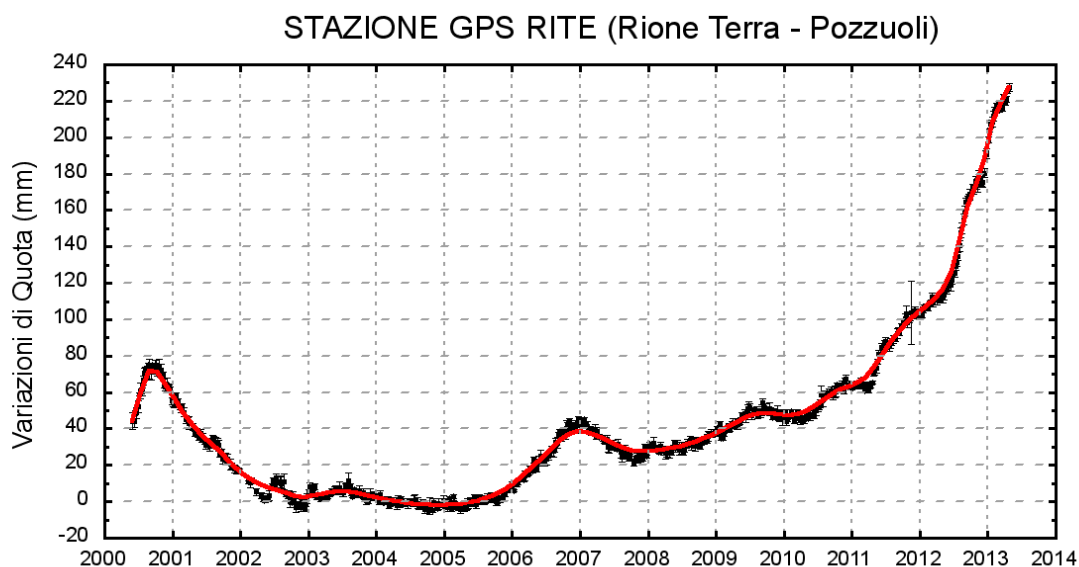
Fig. 2.2.1: Serie temporale delle variazioni settimanali in quota della stazione di RITE (Pozzuoli) dal 2000 al 30 aprile 2013
