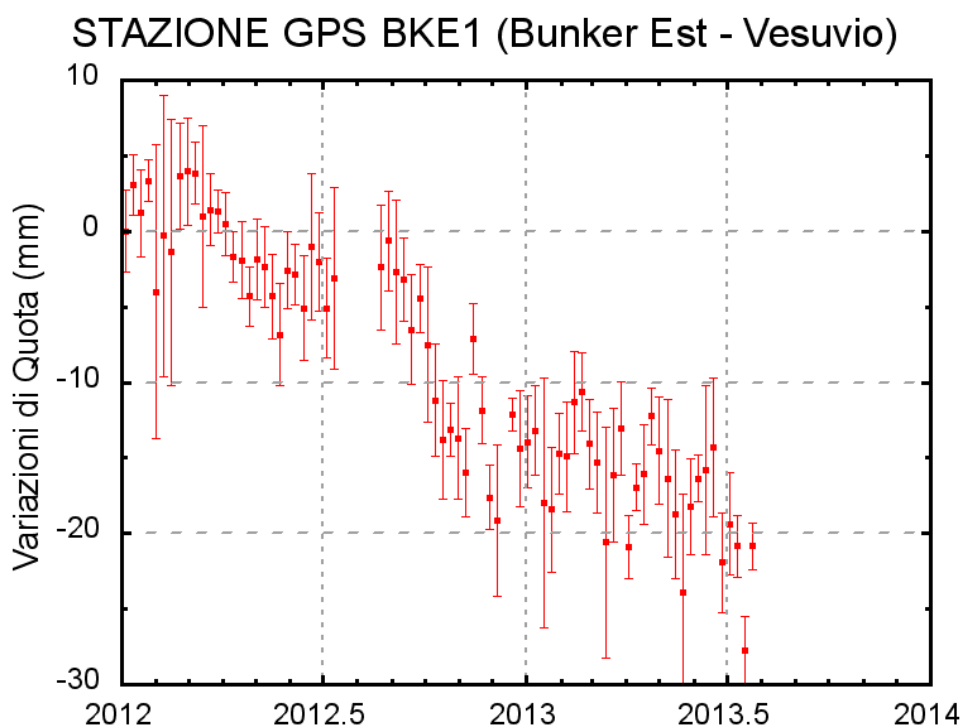
Fig. 1.2.2: Serie temporale delle variazioni settimanali in quota della stazione di BKE1 (Vesuvio) dal 01 gennaio 2012 al 31 luglio 2013
