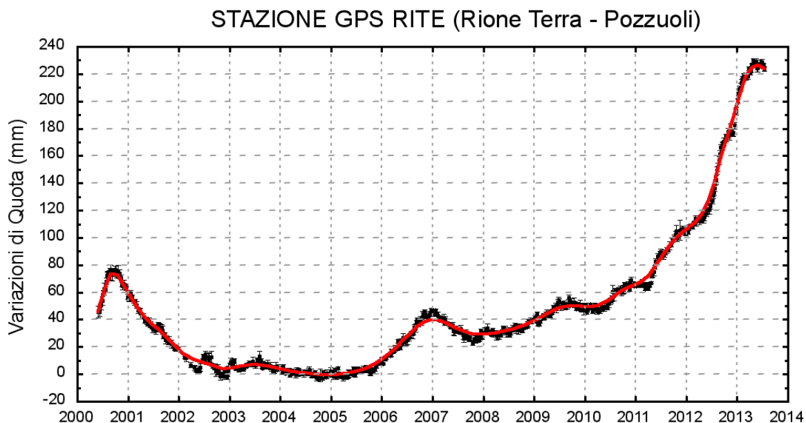
Fig. 2.2.1: Serie temporale delle variazioni settimanali in quota della stazione di RITE (Pozzuoli) dal 2000 al 31 luglio 2013
