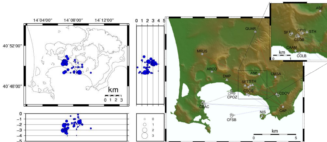
Figura 2.1.2 – Localizzazioni ipocentrali ai Campi Flegrei nel corso degli ultimi 12 mesi (92 eventi). La dimensione dei simboli è proporzionale alla magnitudo, come indicato nel riquadro in basso. A destra è mostrata la mappa con la rete sismica dei Campi Flegrei.
