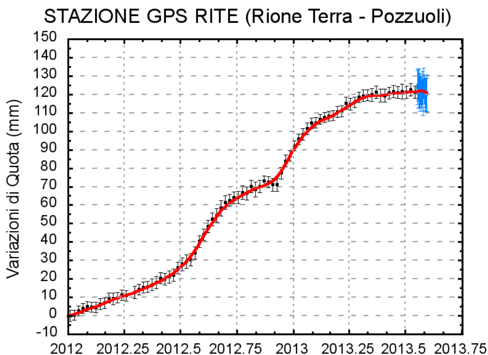
Fig. 2.2.2: Serie temporale delle variazioni in quota della stazione di RITE (Pozzuoli) dal 01 gennaio 2012 al 05 agosto 2013 (vedi bollettino settimanale)
