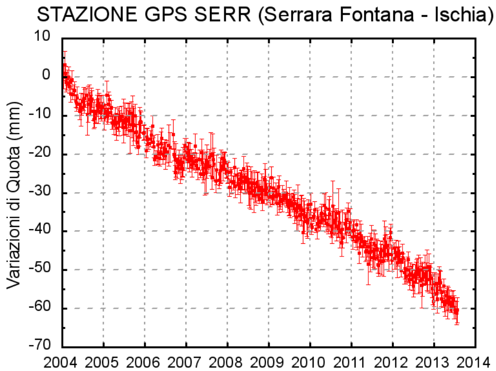
Fig. 3.2.1: Serie temporale delle variazioni settimanali in quota della stazione di SERR (Ischia) dal 2004 al 31 luglio 2013
