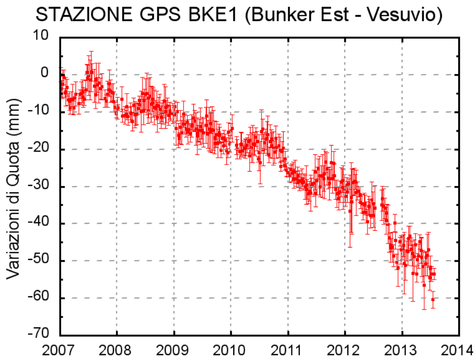
Fig. 1.2.1: Serie temporale delle variazioni settimanali in quota della stazione di BKE1 (Vesuvio) dal 2007 al 31 luglio 2013
