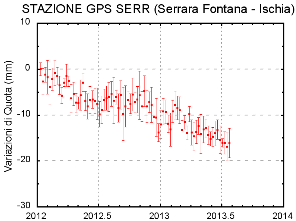
Fig. 3.2.2: Serie temporale delle variazioni settimanali in quota della stazione di SERR (Ischia) dal 01 gennaio 2012 al 31 luglio 2013
