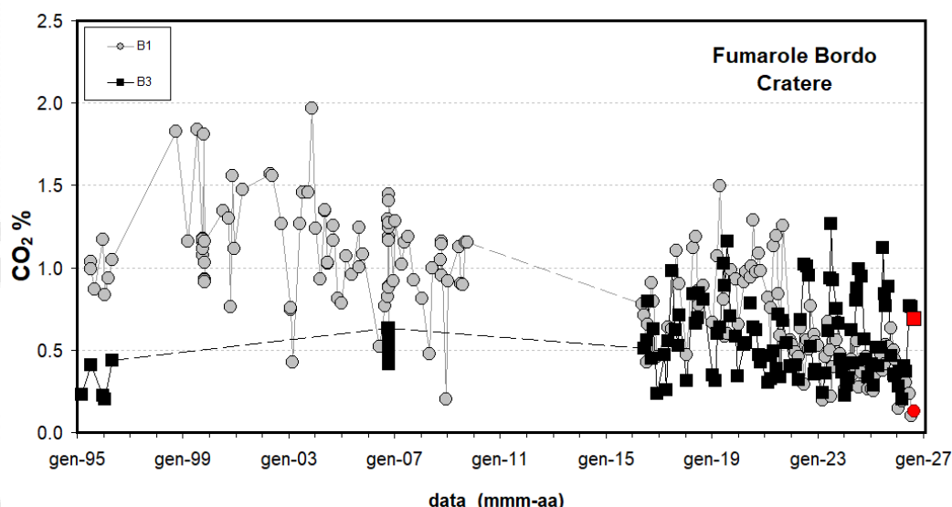
Figura 4.2 - Cronogramma della concentrazione di \text{CO}_2 delle fumarole di bordo cratere B1 (area anemometro) e B3 (sette SW). I campioni delle fumarole B1 e B3 del mese di agosto 2026 sono riportati con il simbolo rosso.
