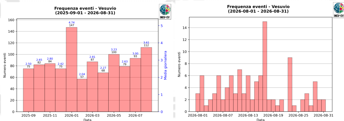
Figura 1.2 - A sinistra il numero di eventi registrati al Vesuvio nel corso degli ultimi 12 mesi (in totale 1059), a destra quelli avvenuti nell'ultimo mese (in totale 112).
