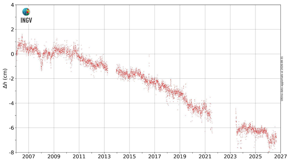
Figura 2.3.3 - Movimenti verticali del suolo, nel periodo gennaio 2006 – agosto 2026, ottenuti dall'analisi dei dati acquisiti dalla stazione mareografica di Torre del Greco, molo Redentore (TRDG). Le variazioni, riportate in cm, rappresentano le medie giornaliere e sono riferite alla stazione mareografica di Napoli molo San Vincenzo (NAMM).
