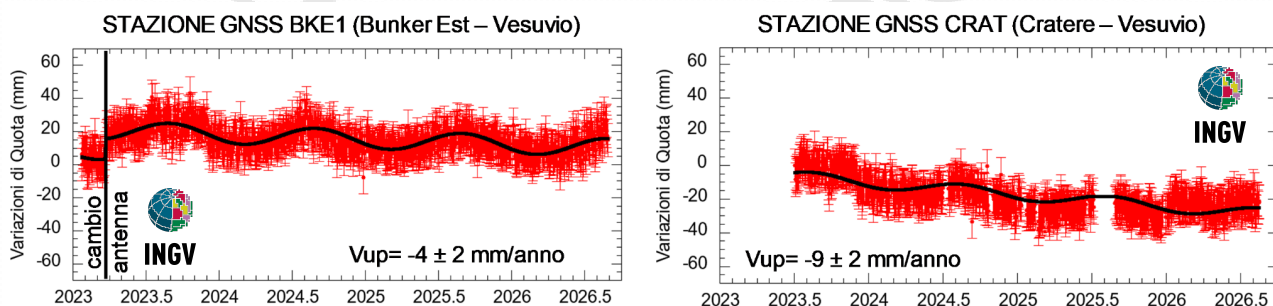
Figura 2.1.2 - Serie temporali delle variazioni giornaliere della componente verticale delle stazioni BKE1 e CRAT (Vesuvio) da gennaio 2023 ad agosto 2026.
