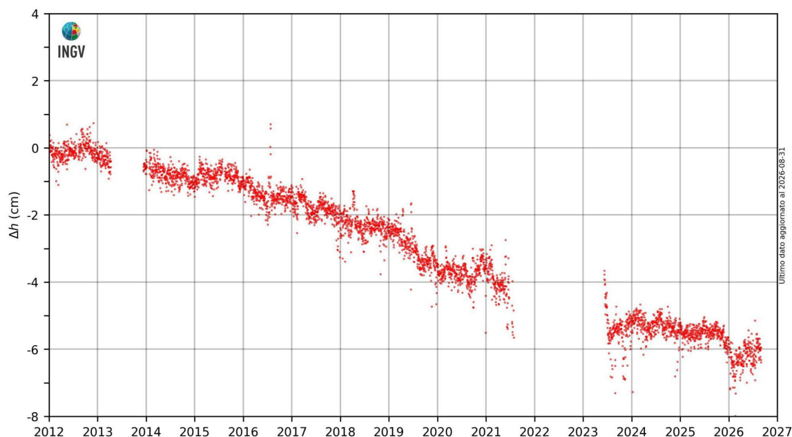
Figura 2.3.2 – Movimenti verticali del suolo, nel periodo gennaio 2012 – agosto 2026, ottenuti dall'analisi dei dati acquisiti dalla stazione mareografica di Torre del Greco, molo Redentore (TRDG). Le variazioni, riportate in cm, rappresentano le medie giornaliere e sono riferite alla stazione mareografica di Napoli, molo San Vincenzo (NAMM).
