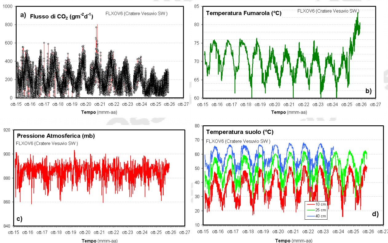
Figura 4.3 - Parametri misurati dalla stazione geochimica (FLXOV6) installata in area bordo cratere del Vesuvio (sette SW). I valori, eccetto il flusso di \text{CO}_2 dal suolo, sono riportati come medie giornaliere.
