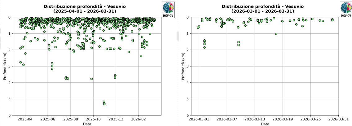
Figura 1.5 - Profondità ipocentrali degli eventi registrati al Vesuvio nel corso degli ultimi 12 mesi (a sinistra) e dell'ultimo mese (a destra).
