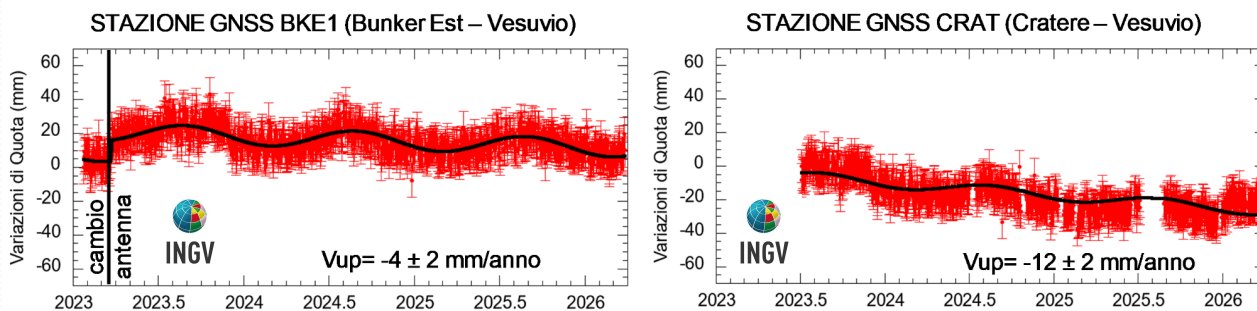
Figura 2.1.2 - Serie temporali delle variazioni giornaliere della componente verticale delle stazioni BKE1 e CRAT (Vesuvio) da gennaio 2023 a marzo 2026.
