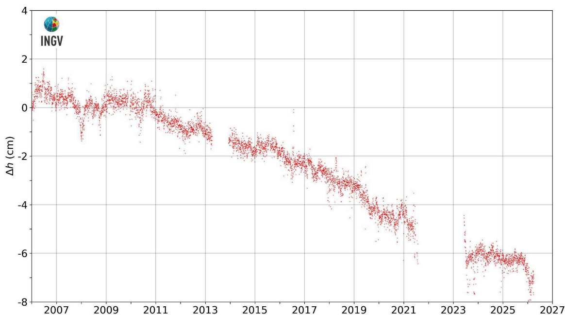
Figura 2.3.3 - Movimenti verticali del suolo, nel periodo gennaio 2006 – marzo 2026, ottenuti dall'analisi dei dati acquisiti dalla stazione mareografica di Torre del Greco, molo Redentore (TRDG). Le variazioni, riportate in cm, rappresentano le medie giornaliere e sono riferite alla stazione mareografica di Napoli molo San Vincenzo (NAMM).
