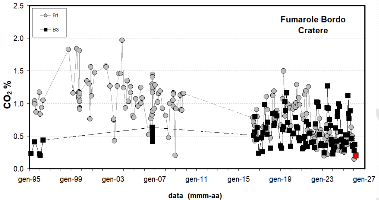
Figura 4.2 - Cronogramma della concentrazione di CO 2 delle fumarole di bordo cratere B1 (area anemometro) e B3 (settore SW). I campioni delle fumarole B1 e B3 del mese di febbraio 2026 sono riportati con il simbolo rosso.
