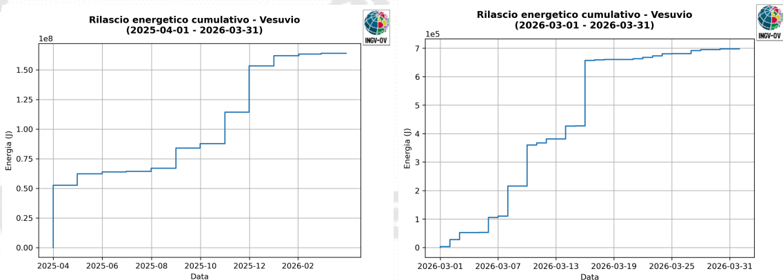
Figura 1.7 - Rilascio cumulativo di energia sismica al Vesuvio nel corso degli ultimi 12 mesi (a sinistra) e dell'ultimo mese (a destra).
