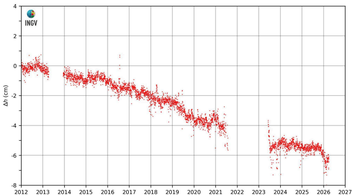
Figura 2.3.2 – Movimenti verticali del suolo, nel periodo gennaio 2012 – marzo 2026, ottenuti dall'analisi dei dati acquisiti dalla stazione mareografica di Torre del Greco, molo Redentore (TRDG). Le variazioni, riportate in cm, rappresentano le medie giornaliere e sono riferite alla stazione mareografica di Napoli, molo San Vincenzo (NAMM).
