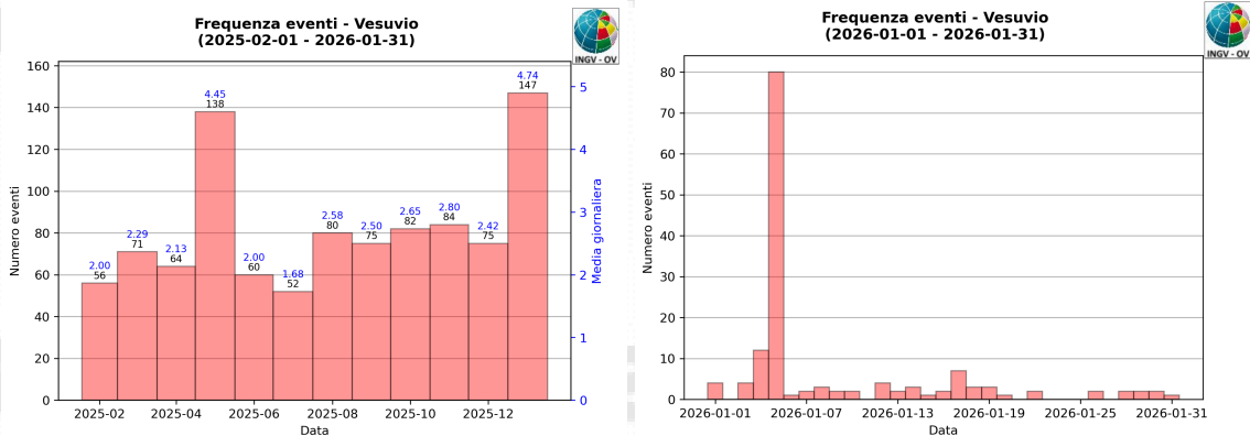
Figura 1.2 - A sinistra il numero di eventi registrati al Vesuvio nel corso degli ultimi 12 mesi (in totale 984), mentre a destra quelli avvenuti nell'ultimo mese (in totale 147).
