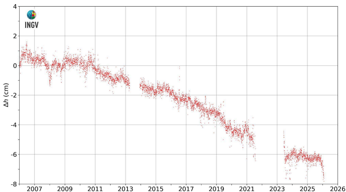
Figura 2.3.3 - Movimenti verticali del suolo, nel periodo gennaio 2006 – gennaio 2026, ottenuti dall'analisi dei dati acquisiti dalla stazione mareografica di Torre del Greco, molo Redentore (TRDG). Le variazioni, riportate in cm, rappresentano le medie giornaliere e sono riferite alla stazione mareografica di Napoli molo San Vincenzo (NAMM).
