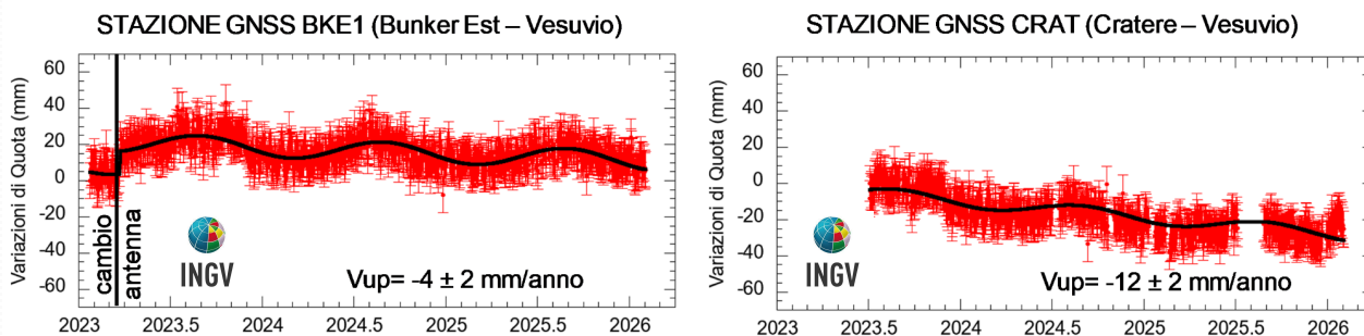
Figura 2.1.2 - Serie temporali delle variazioni giornaliere della componente verticale delle stazioni BKE1 e CRAT (Vesuvio) da gennaio 2023 a gennaio 2026.
