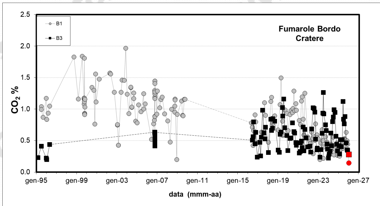
Figura 4.2 - Cronogramma della concentrazione di CO 2 delle fumarole di bordo cratere B1 (area anemometro) e B3 (settore SW). I campioni delle fumarole B1 e B3 del mese di gennaio 2026 sono riportati con il simbolo rosso.
