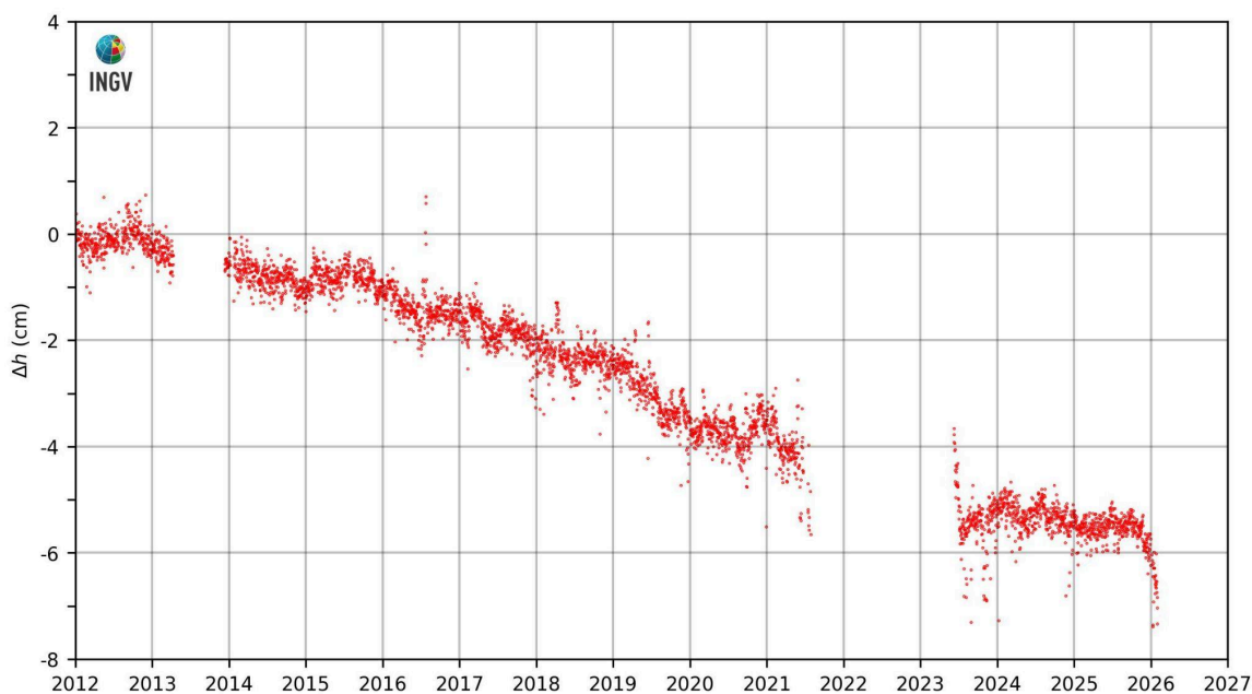
Figura 2.3.2 – Movimenti verticali del suolo, nel periodo gennaio 2012 – gennaio 2026, ottenuti dall'analisi dei dati acquisiti dalla stazione mareografica di Torre del Greco, molo Redentore (TRDG). Le variazioni, riportate in cm, rappresentano le medie giornaliere e sono riferite alla stazione mareografica di Napoli, molo San Vincenzo (NAMM).
