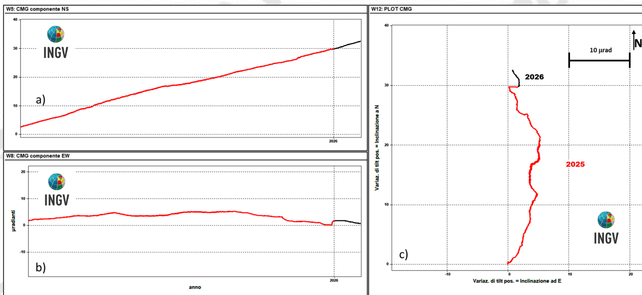
Figura 2.2.2 – Serie temporali e plot (ultimi 12 mesi) del tilt della stazione CMG della rete del Vesuvio.
