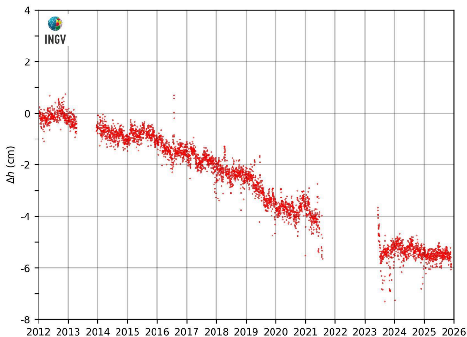
Figura 2.3.2 – Movimenti verticali del suolo, nel periodo gennaio 2012 – novembre 2025, ottenuti dall’analisi dei dati acquisiti dalla stazione mareografica di Torre del Greco, molo Redentore (TRDG). Le variazioni, riportate in cm, rappresentano le medie giornaliere e sono riferite alla stazione mareografica di Napoli, molo San Vincenzo (NAMM).
