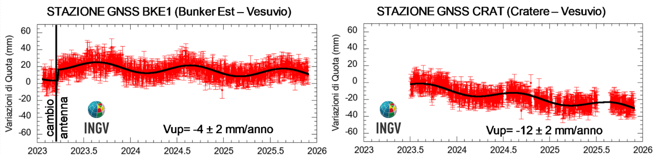
Figura 2.1.2 - Serie temporali delle variazioni giornaliere della componente verticale delle stazioni BKE1 e CRAT (Vesuvio) da gennaio 2023 a novembre 2025.
