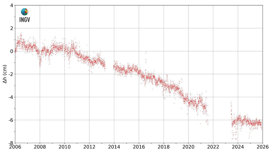
Figura 2.3.3 - Movimenti verticali del suolo, nel periodo gennaio 2006 – novembre 2025, ottenuti dall’analisi dei dati acquisiti dalla stazione mareografica di Torre del Greco, molo Redentore (TRDG). Le variazioni, riportate in cm, rappresentano le medie giornaliere e sono riferite alla stazione mareografica di Napoli molo San Vincenzo (NAMM).
