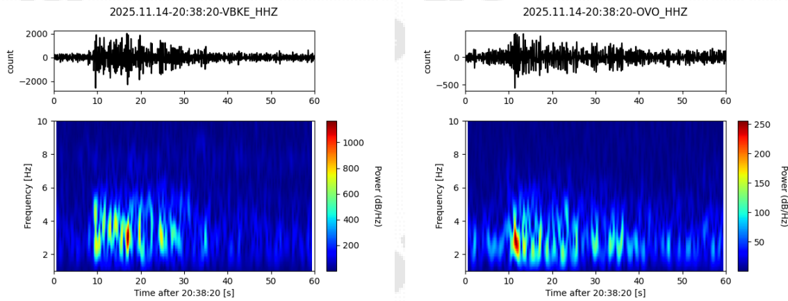
Figura 1.3 – Spettrogramma dell'evento registrato il 14/11/2025 alle 20:38 UTC alla stazione VBKE (a sinistra) e OVO (a destra)
