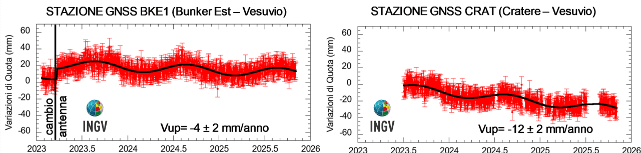
Figura 2.1.2 - Serie temporali delle variazioni giornaliere della componente verticale delle stazioni BKE1 e CRAT (Vesuvio) da gennaio 2023 a ottobre 2025.
