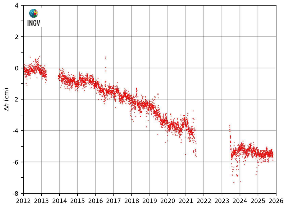
Figura 2.3.2 – Movimenti verticali del suolo, nel periodo gennaio 2012 – ottobre 2025, ottenuti dall'analisi dei dati acquisiti dalla stazione mareografica di Torre del Greco, molo Redentore (TRDG). Le variazioni, riportate in cm, rappresentano le medie giornaliere e sono riferite alla stazione mareografica di Napoli, molo San Vincenzo (NAMM).
