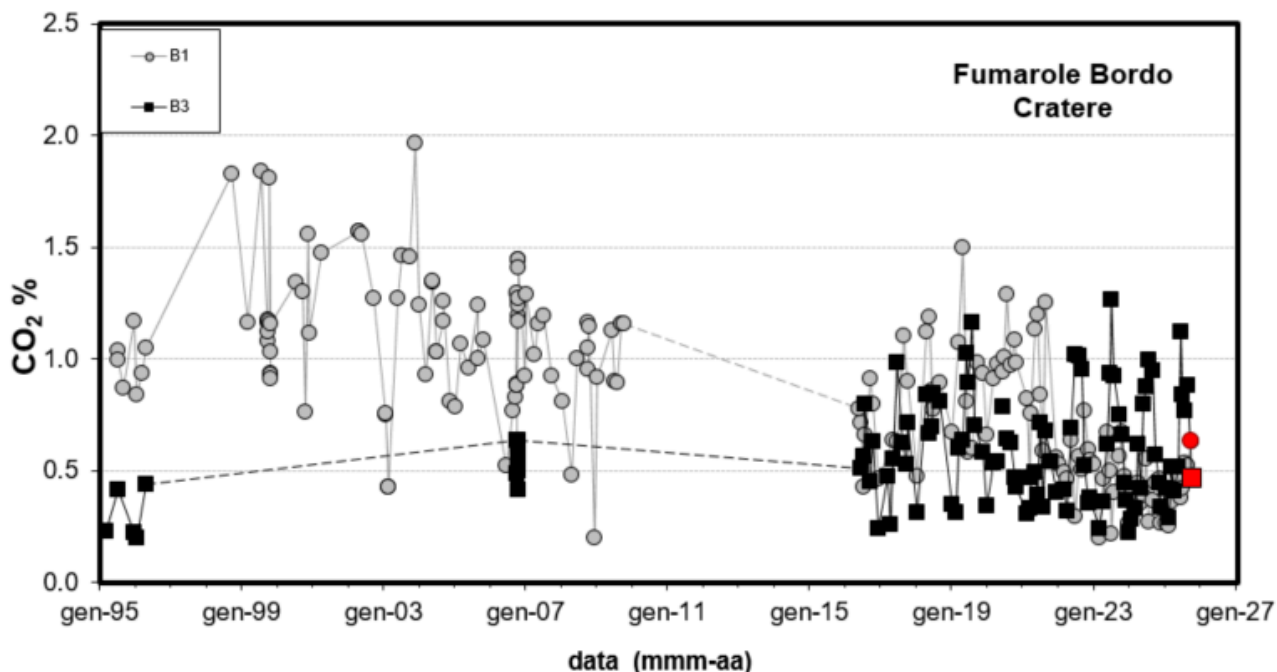
Figura 4.2 - Cronogramma della concentrazione di CO 2 delle fumarole di bordo cratere B1 (area anemometro) e B3 (settore SW). I campioni delle fumarole B1 e B3 del mese di ottobre 2025 sono riportati con il simbolo rosso.
