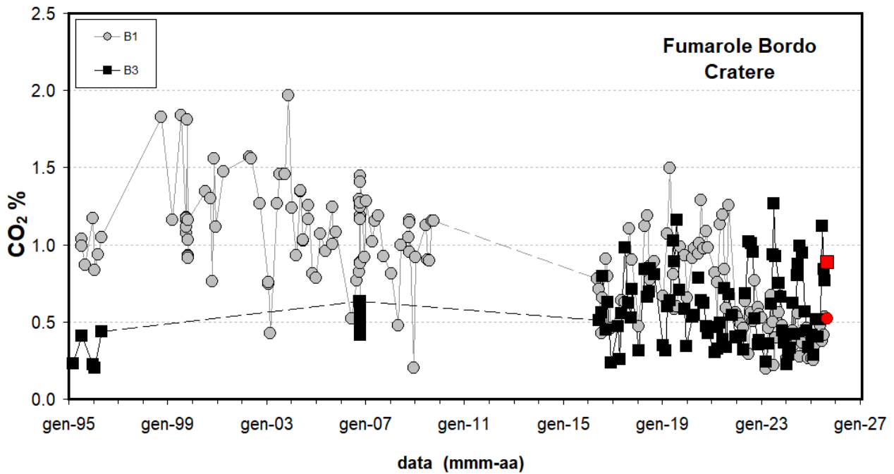
Figura 4.2 - Cronogramma della concentrazione di CO 2 delle fumarole di bordo cratere B1 (area anemometro) e B3 (settore SW). I campioni delle fumarole B1 e B3 del mese di settembre 2025 sono riportati con il simbolo rosso.
