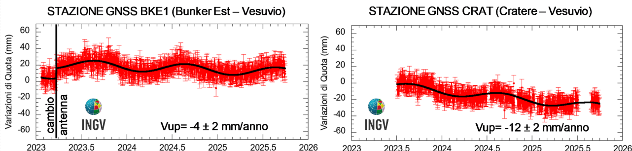
Figura 2.1.2 - Serie temporali delle variazioni giornaliere della componente verticale delle stazioni BKE1 e CRAT (Vesuvio) da gennaio 2023 a settembre 2025.
