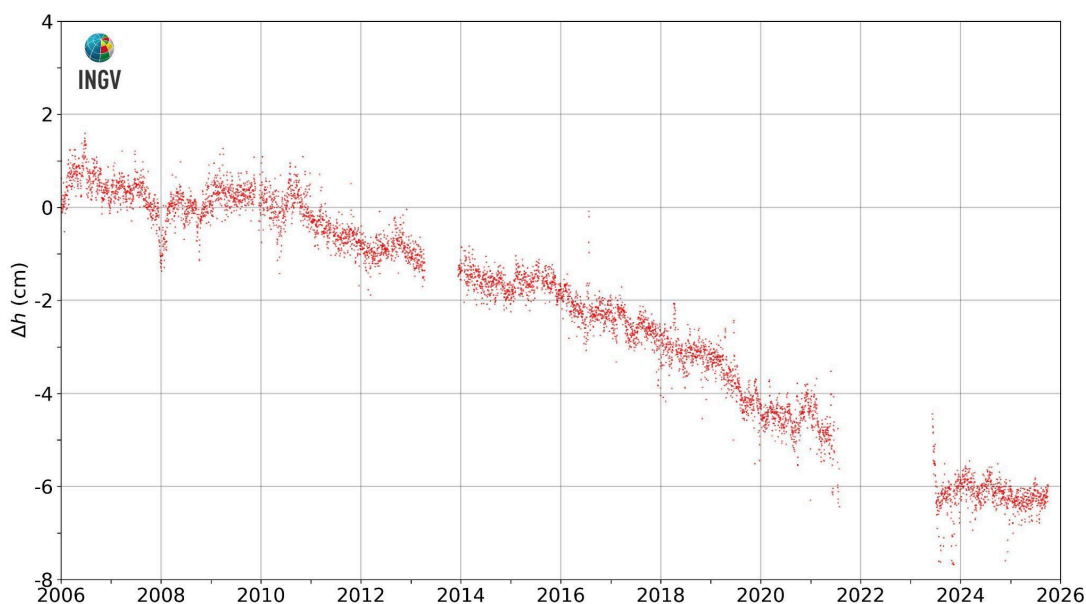
Figura 2.3.3 - Movimenti verticali del suolo, nel periodo gennaio 2006 – settembre 2025, ottenuti dall’analisi dei dati acquisiti dalla stazione mareografica di Torre del Greco, molo Redentore (TRDG). Le variazioni, riportate in cm, rappresentano le medie giornaliere e sono riferite alla stazione mareografica di Napoli molo San Vincenzo (NAMM).
