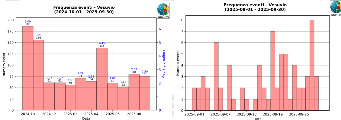
Figura 1.2 - A sinistra il numero di eventi registrati al Vesuvio nel corso degli ultimi 12 mesi (in totale 1060), mentre a destra quelli avvenuti nell'ultimo mese (in totale 75).
