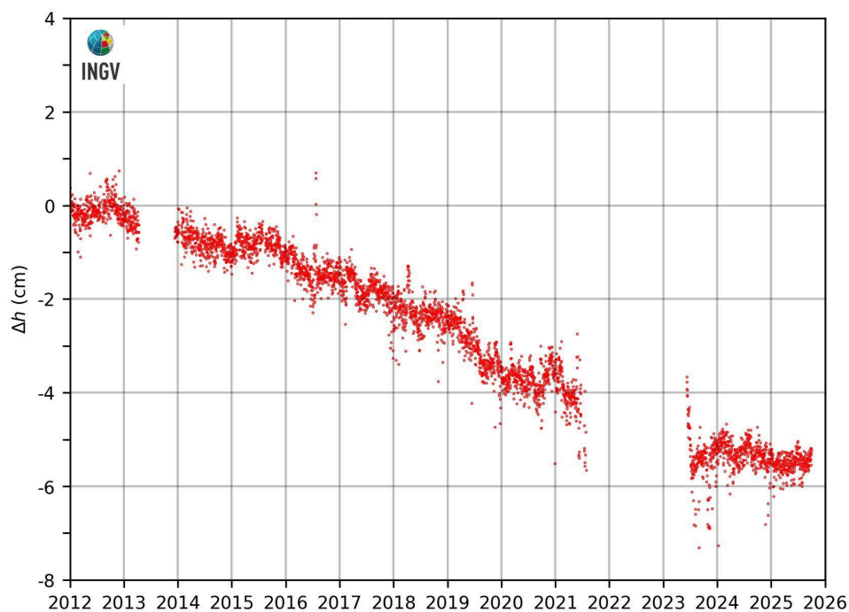
Figura 2.3.2 – Movimenti verticali del suolo, nel periodo gennaio 2012 – settembre 2025, ottenuti dall’analisi dei dati acquisiti dalla stazione mareografica di Torre del Greco, molo Redentore (TRDG). Le variazioni, riportate in cm, rappresentano le medie giornaliere e sono riferite alla stazione mareografica di Napoli, molo San Vincenzo (NAMM).
