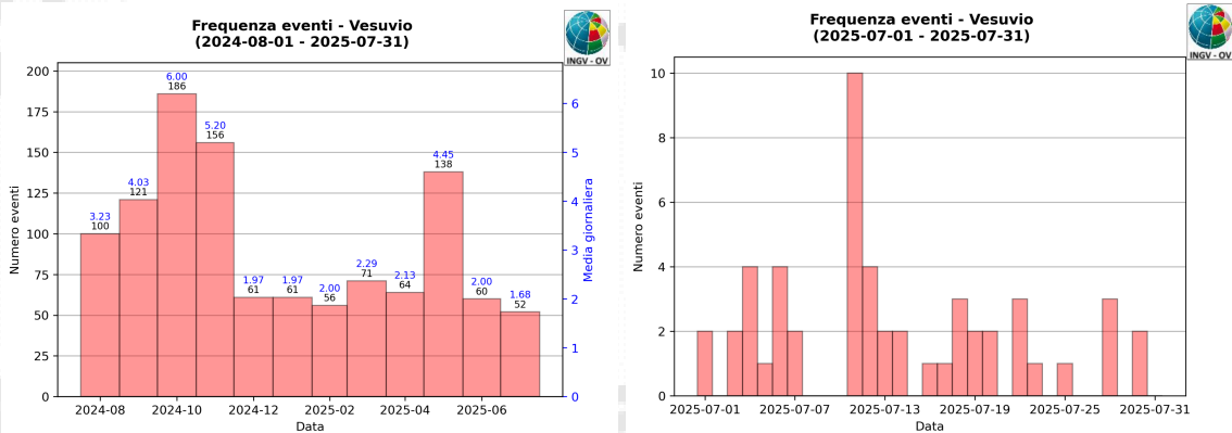
Figura 1.2 - A sinistra il numero di eventi registrati al Vesuvio nel corso degli ultimi 12 mesi (in totale 1126), mentre a destra quelli avvenuti nell'ultimo mese (in totale 52).
