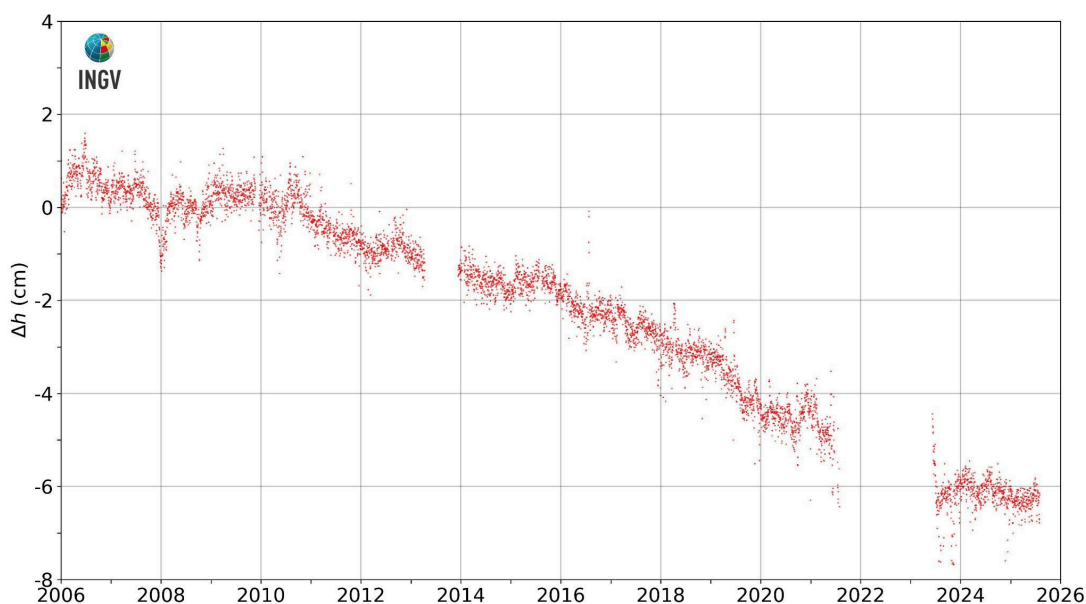
Figura 2.3.3 - Movimenti verticali del suolo, nel periodo gennaio 2006 – luglio 2025, ottenuti dall'analisi dei dati acquisiti dalla stazione mareografica di Torre del Greco, molo Redentore (TRDG). Le variazioni, riportate in cm, rappresentano le medie giornaliere e sono riferite alla stazione mareografica di Napoli molo San Vincenzo (NAMM).
