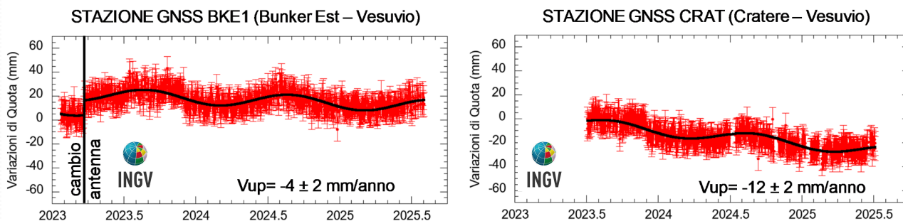
Figura 2.1.2 - Serie temporali delle variazioni giornaliere della componente verticale delle stazioni BKE1 e CRAT (Vesuvio) da gennaio 2023 a luglio 2025.
