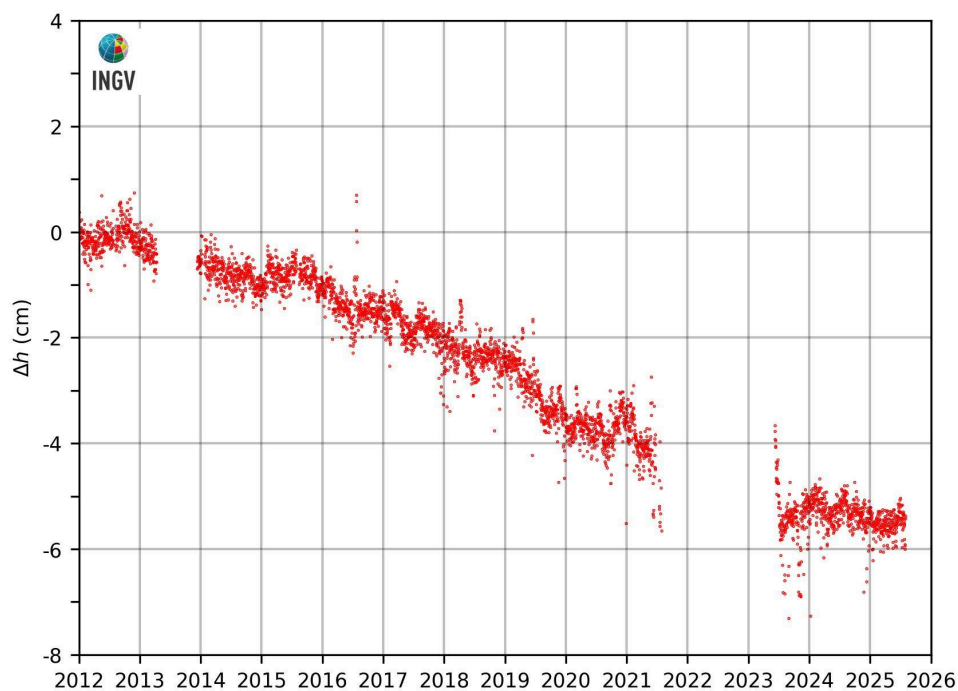
Figura 2.3.2 – Movimenti verticali del suolo, nel periodo gennaio 2012 – luglio 2025, ottenuti dall'analisi dei dati acquisiti dalla stazione mareografica di Torre del Greco, molo Redentore (TRDG). Le variazioni, riportate in cm, rappresentano le medie giornaliere e sono riferite alla stazione mareografica di Napoli, molo San Vincenzo (NAMM).
