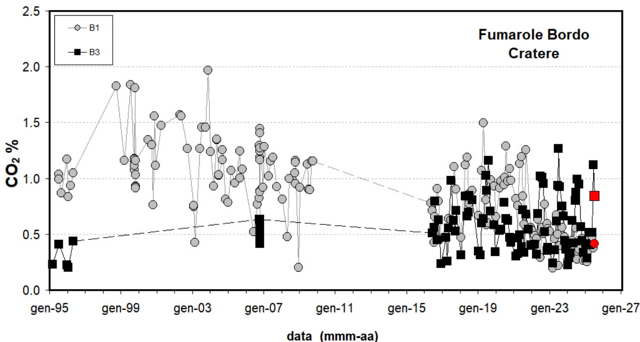
Figura 4.2 - Cronogramma della concentrazione di CO 2 delle fumarole di bordo cratere B1 (area anemometro) e B3 (settore SW). I campioni delle fumarole B1 e B3 del mese di luglio 2025 sono riportati con il simbolo rosso.
