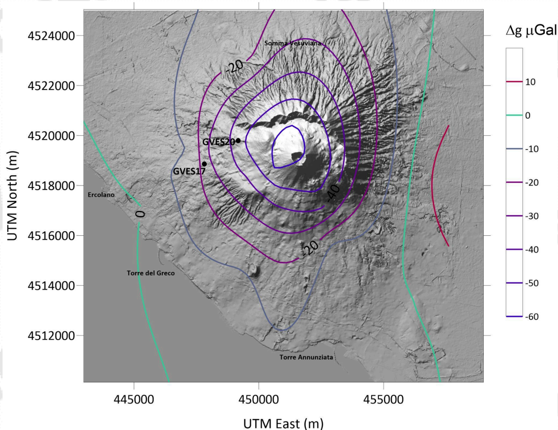
Figura 2.4.2 -Variazioni di gravità \Delta g , con riferimento al vertice di Napoli S. Marcellino, ottenute tra la campagna di aprile-maggio 2025 e aprile 2024. L'equidistanza delle isolinee è di 10\mu\text{Gal} , gli errori stimati sulla rete sono pari a \pm 10\mu\text{Gal} , per la campagna del 2024, e \pm 8\mu\text{Gal} , per la campagna 2025. E' indicata la posizione dei due caposaldi per i quali si riportano le serie temporali in figura 2.4.3
