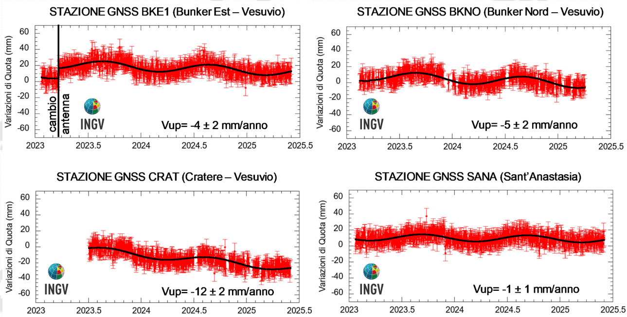
Figura 2.1.2 - Serie temporali delle variazioni giornaliere della componente verticale delle stazioni BKE1, BKNO, CRAT e SANA (Vesuvio) da gennaio 2023 a maggio 2025.
