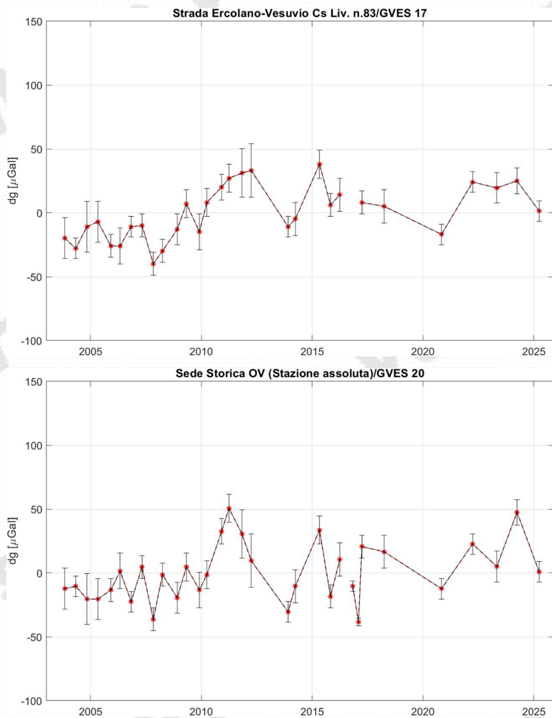
Figura 2.4.3 - Serie temporali dal 2004, aggiornate all'ultima campagna del 2025, osservate a 2 caposaldi (GVES17 e GVES20) della rete gravimetrica del Vesuvio.
