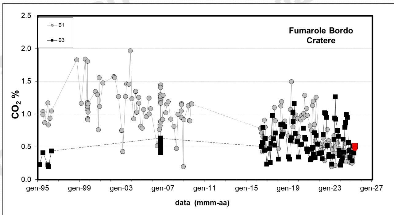
Figura 4.2 - Cronogramma della concentrazione di CO 2 delle fumarole di bordo cratere B1 (area anemometro) e B3 (settore SW). I campioni delle fumarole B1 e B3 del mese di maggio 2025 sono riportati con il simbolo rosso.
