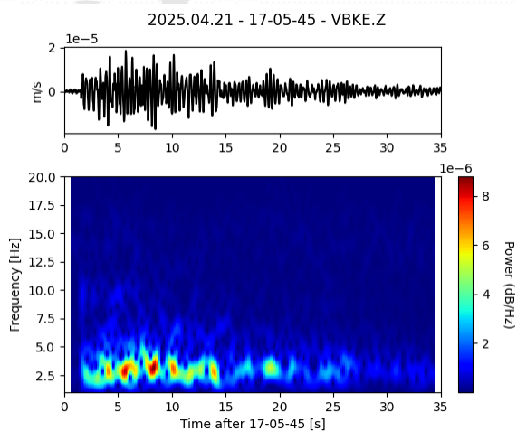
Figura 1.7 – Spettrogramma dell'evento registrato il 21/04/2025 alle 17:05 UTC alla stazione Bunker Est (VBKE).
