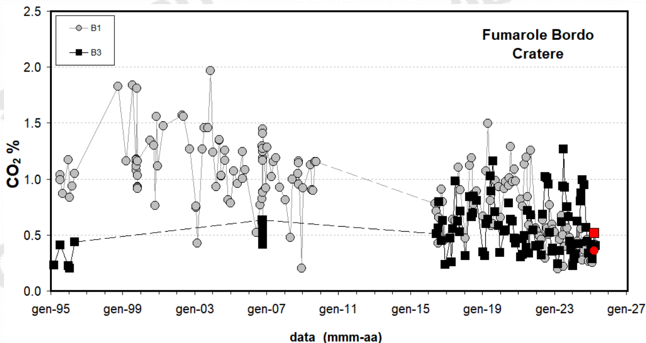
Figura 4.2 - Cronogramma della concentrazione di CO 2 delle fumarole di bordo cratere B1 (area anemometro) e B3 (settor SW). I campioni delle fumarole B1 e B3 del mese di aprile 2025 sono riportati con il simbolo rosso.
