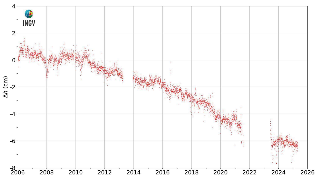
Figura 2.3.3 - Movimenti verticali del suolo, nel periodo gennaio 2006 – aprile 2025, ottenuti dall'analisi dei dati acquisiti dalla stazione mareografica di Torre del Greco, molo Redentore (TRDG). Le variazioni, riportate in cm, rappresentano le medie giornaliere e sono riferite alla stazione mareografica di Napoli molo San Vincenzo (NAMM).
