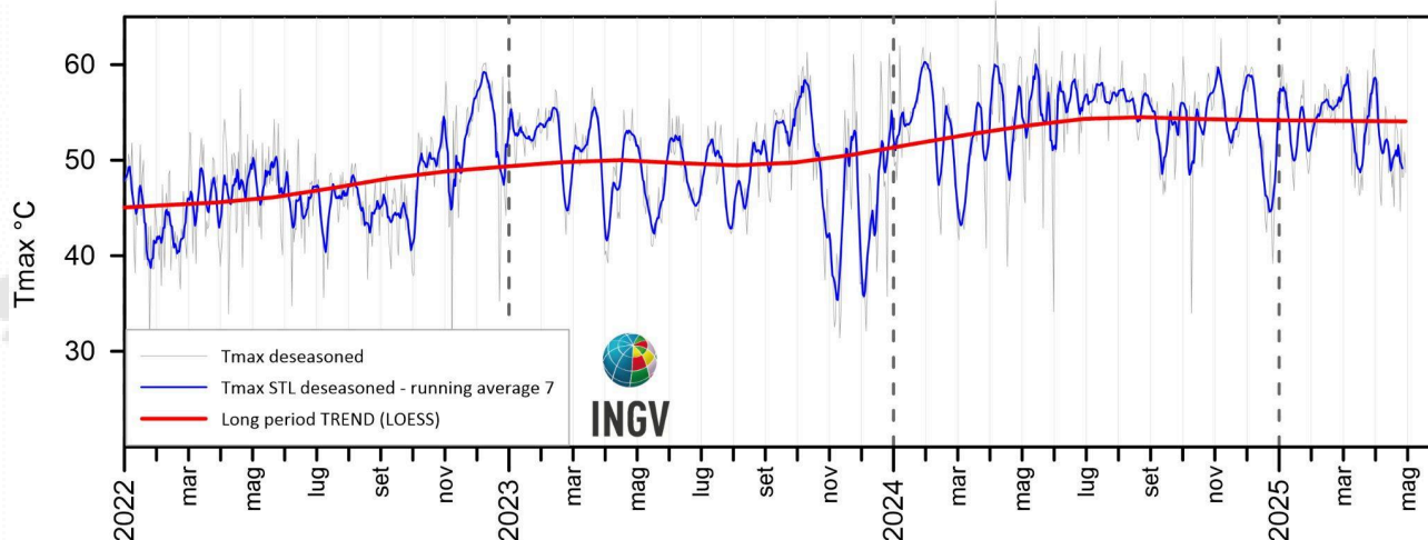
Figura 3.1.2 - Stazione Vesuvio VES1. Serie temporali dei valori di temperatura massima giornaliera rilevata nelle immagini IR, destagionalizzate mediante applicazione dell'algoritmo BR (medie settimanali termocamera 640x480). Il trend a lungo termine è ottenuto applicando un fitting LOESS di 2° alle temperature massime destagionalizzate.
