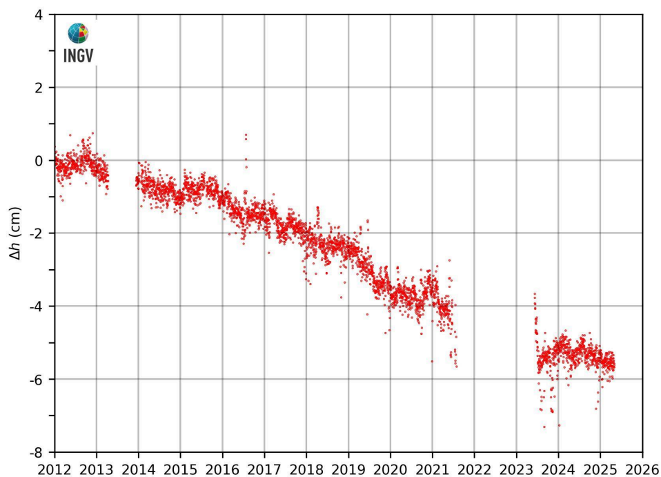
Figura 2.3.2 – Movimenti verticali del suolo, nel periodo gennaio 2012 – aprile 2025, ottenuti dall'analisi dei dati acquisiti dalla stazione mareografica di Torre del Greco, molo Redentore (TRDG). Le variazioni, riportate in cm, rappresentano le medie giornaliere e sono riferite alla stazione mareografica di Napoli, molo San Vincenzo (NAMM).
