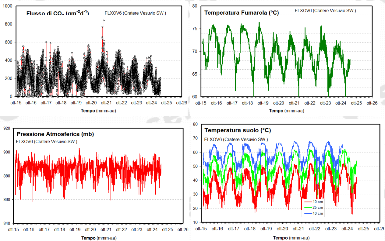
Figura 4.3 - Parametri misurati dalla stazione geochimica (FLXOV6) installata in area bordo cratere del Vesuvio (settor SW). I valori, eccetto il flusso di CO 2 dal suolo, sono riportati come medie giornaliere.
