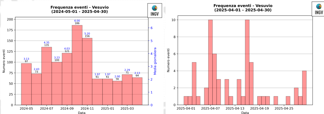
Figura 1.2 - A sinistra il numero di eventi registrati al Vesuvio nel corso degli ultimi 12 mesi (in totale 1181), mentre a destra quelli avvenuti nell'ultimo mese (in totale 64).
