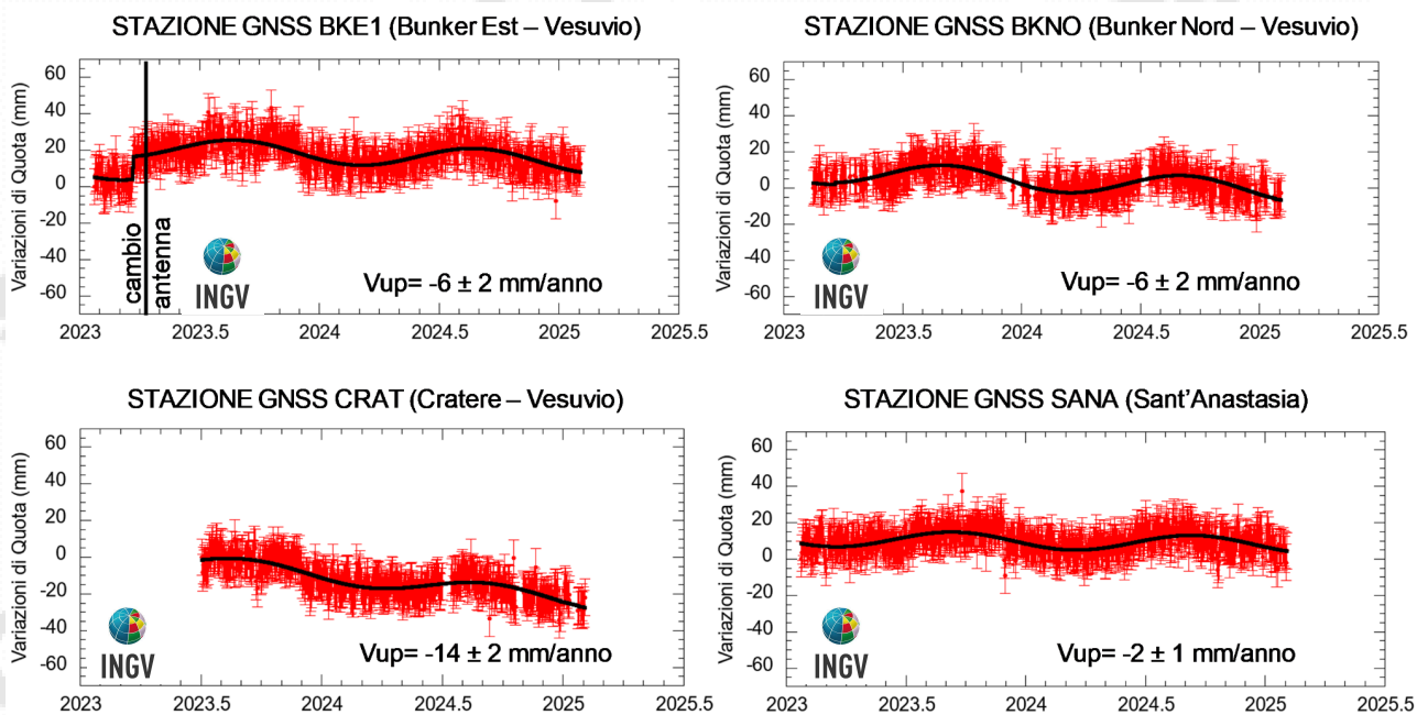
Figura 2.1.2 - Serie temporali delle variazioni giornaliere della componente verticale delle stazioni BKE1, BKNO, CRAT e SANA (Vesuvio) da gennaio 2023 a gennaio 2025.
