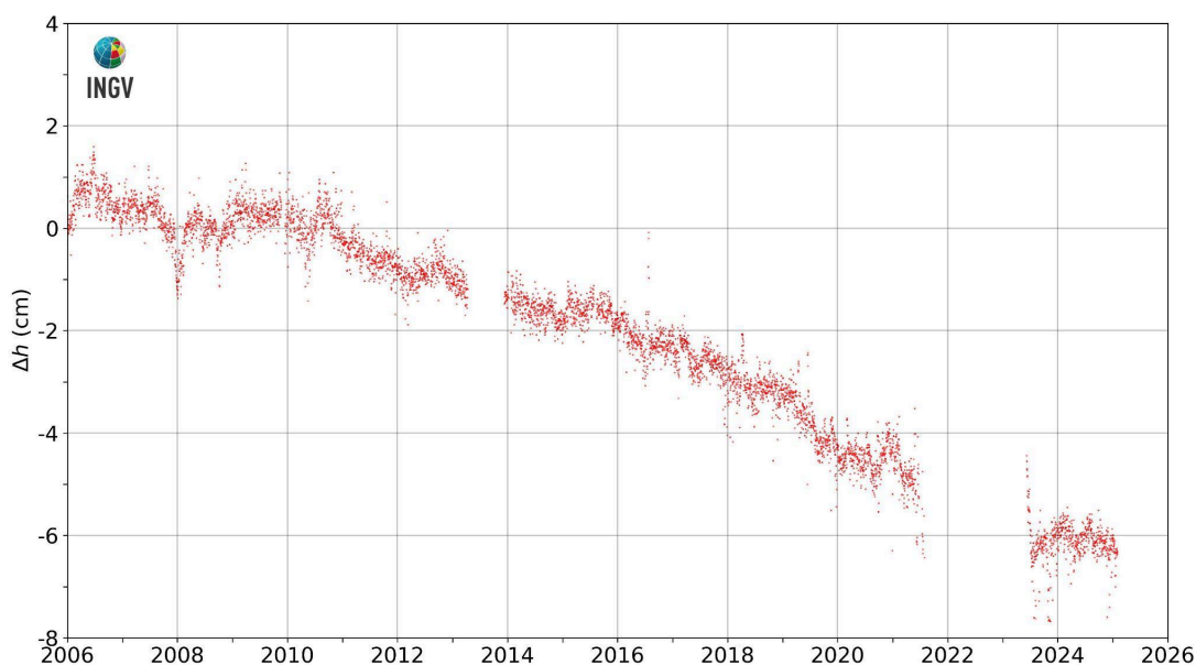
Figura 2.3.3 - Movimenti verticali del suolo, nel periodo gennaio 2006 – gennaio 2025, ottenuti dall'analisi dei dati acquisiti dalla stazione mareografica di Torre del Greco, molo Redentore (TRDG). Le variazioni, riportate in cm, rappresentano le medie giornaliere e sono riferite alla stazione mareografica di Napoli molo San Vincenzo (NAMM).
