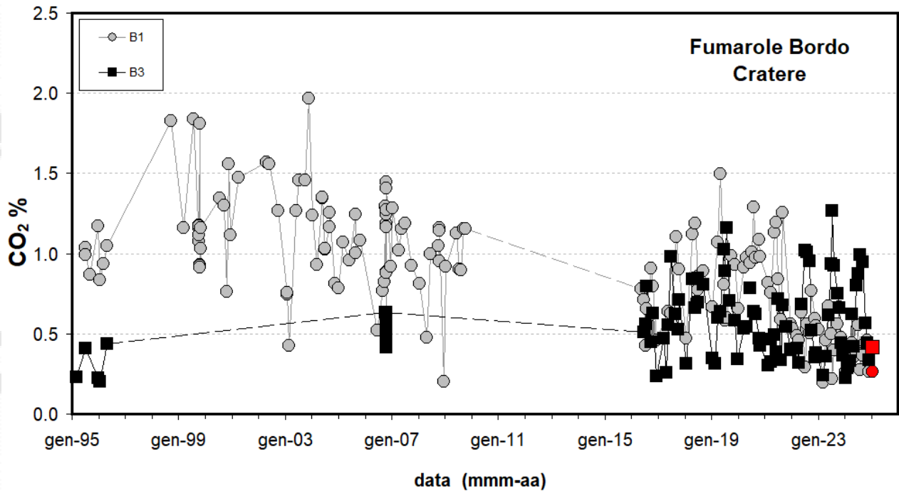
Figura 4.2 - Cronogramma della concentrazione di CO 2 delle fumarole di bordo cratere B1 (area anemometro) e B3 (settore SW). I campioni delle fumarole B1 e B3 del mese di gennaio 2025 sono riportati con il simbolo rosso.
