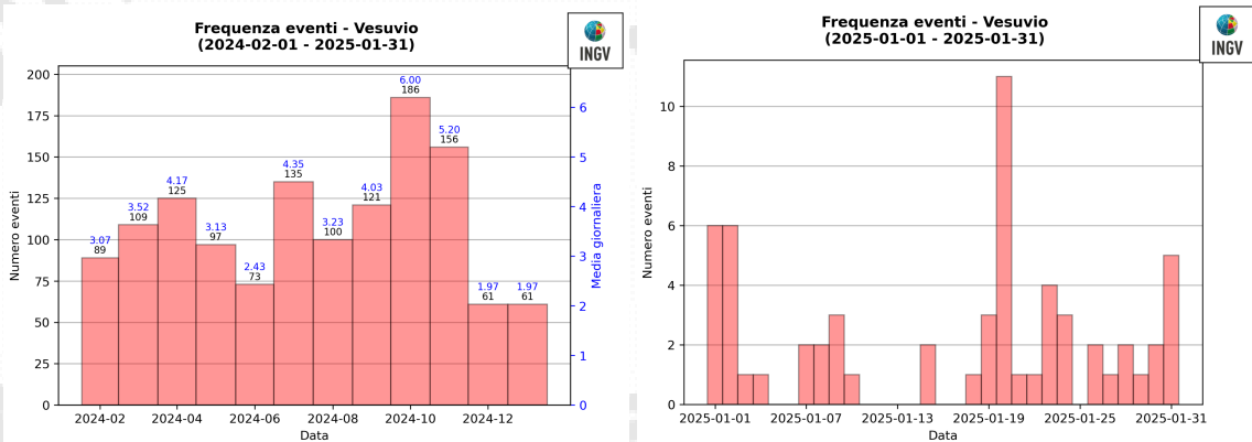
Figura 1.2 - A sinistra il numero di eventi registrati al Vesuvio nel corso degli ultimi 12 mesi (in totale 1313), mentre a destra quelli avvenuti nell'ultimo mese (in totale 61).
