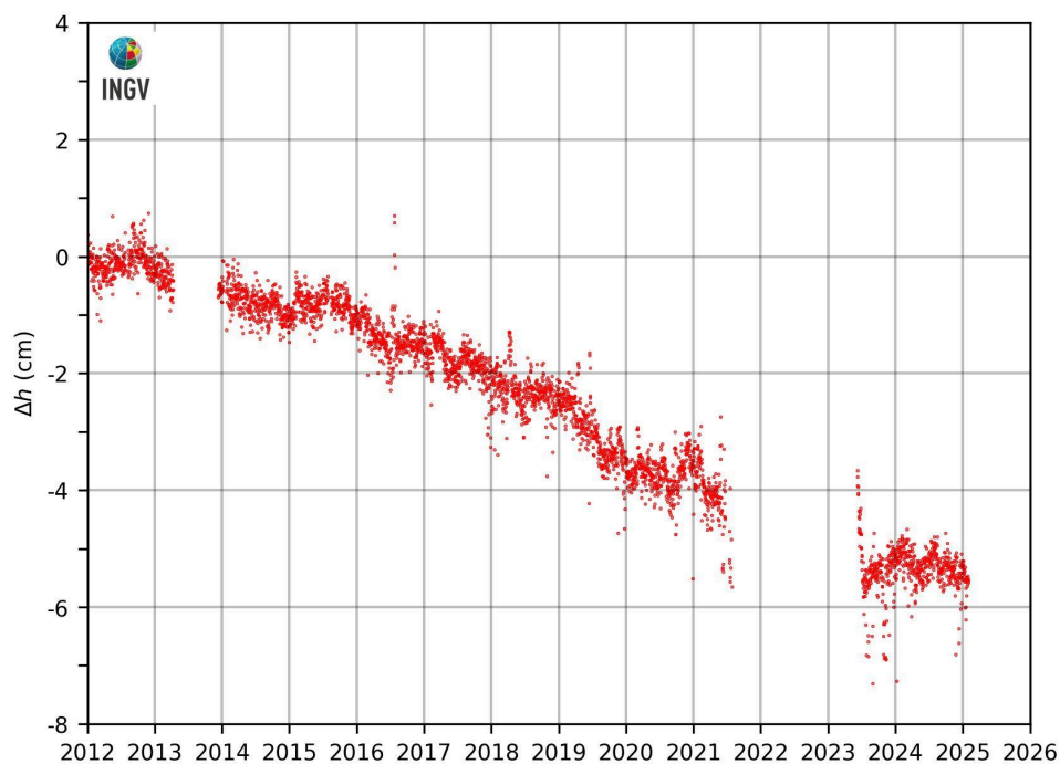
Figura 2.3.2 – Movimenti verticali del suolo, nel periodo gennaio 2012 – gennaio 2025, ottenuti dall'analisi dei dati acquisiti dalla stazione mareografica di Torre del Greco, molo Redentore (TRDG). Le variazioni, riportate in cm, rappresentano le medie giornaliere e sono riferite alla stazione mareografica di Napoli, molo San Vincenzo (NAMM).
