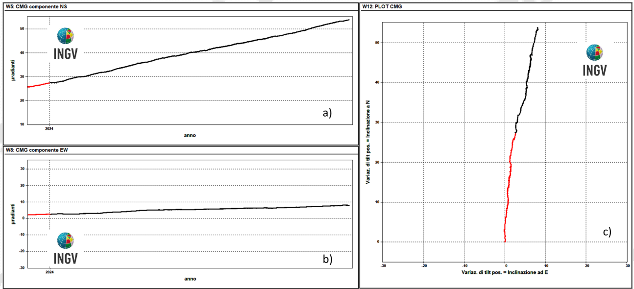
Figura 2.2.2 – Serie temporali (gennaio 2024 - dicembre 2024) e plot (gennaio 2023 - dicembre 2024) del tilt della stazione CMG della rete del Vesuvio.
