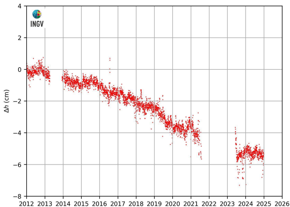
Figura 2.3.2 – Movimenti verticali del suolo, nel periodo gennaio 2012 – dicembre 2024, ottenuti dall’analisi dei dati acquisiti dalla stazione mareografica di Torre del Greco, molo Redentore (TRDG). Le variazioni, riportate in cm, rappresentano le medie giornaliere e sono riferite alla stazione mareografica di Napoli, molo San Vincenzo (NAMM).
