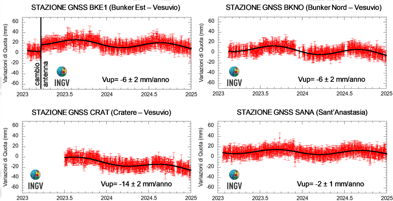
Figura 2.1.2 - Serie temporali delle variazioni giornaliere della componente verticale delle stazioni BKE1, BKNO, CRAT e SANA (Vesuvio) da gennaio 2023 a dicembre 2024.
