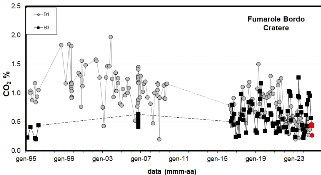
Figura 4.2 - Cronogramma della concentrazione di CO 2 delle fumarole di bordo cratere B1 (area anemometro) e B3 (settore SW). I campioni delle fumarole B1 e B3 del mese di dicembre 2024 sono riportati con il simbolo rosso.
