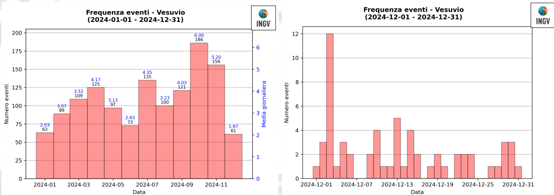
Figura 1.2 - A sinistra il numero di eventi registrati al Vesuvio nel corso degli ultimi 12 mesi (in totale 1315), mentre a destra quelli avvenuti nell'ultimo mese (in totale 61).
