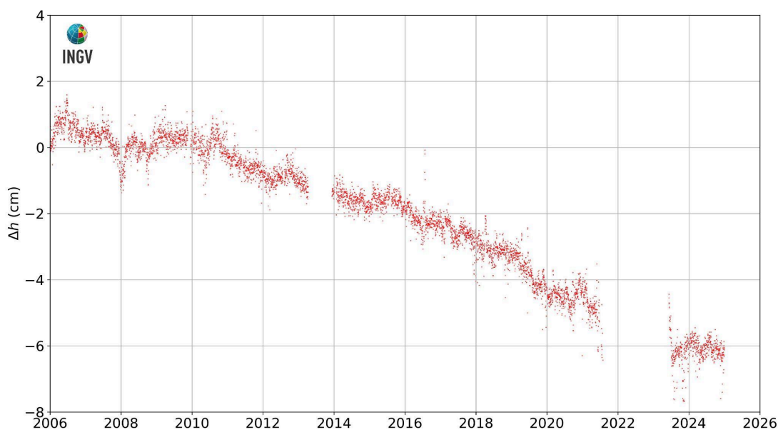
Figura 2.3.3 - Movimenti verticali del suolo, nel periodo gennaio 2006 – dicembre 2024, ottenuti dall’analisi dei dati acquisiti dalla stazione mareografica di Torre del Greco, molo Redentore (TRDG). Le variazioni, riportate in cm, rappresentano le medie giornaliere e sono riferite alla stazione mareografica di Napoli molo San Vincenzo (NAMM).
