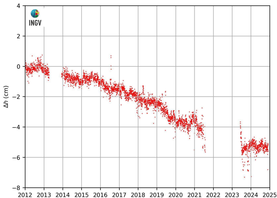
Figura 2.3.2 – Movimenti verticali del suolo, nel periodo gennaio 2012 – novembre 2024, ottenuti dall’analisi dei dati acquisiti dalla stazione mareografica di Torre del Greco, molo Redentore (TRDG). Le variazioni, riportate in cm, rappresentano le medie giornaliere e sono riferite alla stazione mareografica di Napoli, molo San Vincenzo (NAMM).
