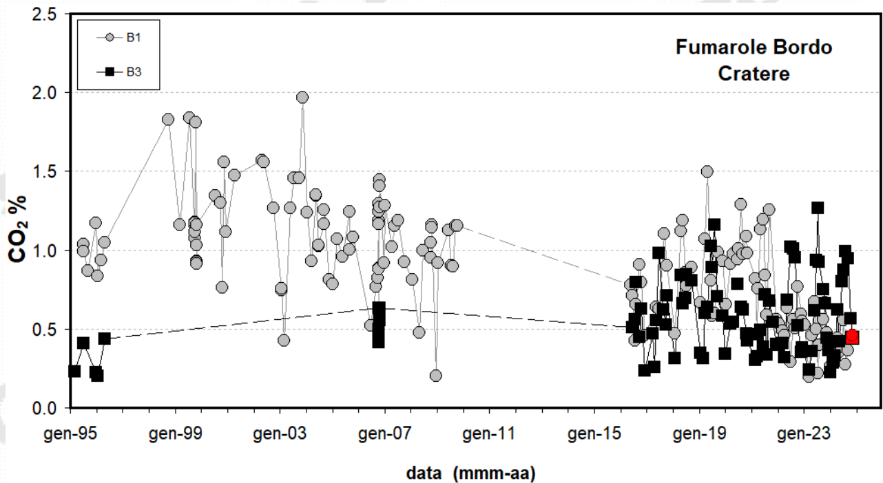
Figura 4.2 - Cronogramma della concentrazione di CO 2 delle fumarole di bordo cratere B1 (area anemometro) e B3 (settore SW). I campioni delle fumarole B1 e B3 del mese di novembre 2024 sono riportati con il simbolo rosso.
