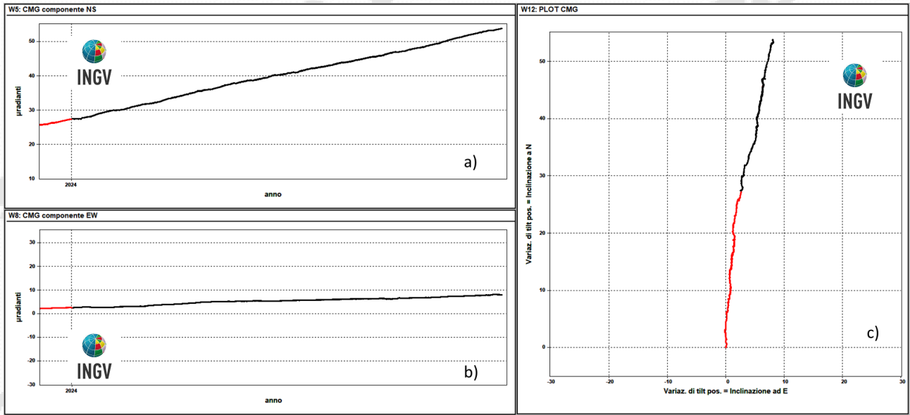
Figura 2.2.2 – Serie temporali e plot del tilt della stazione CMG della rete del Vesuvio registrati negli ultimi 12 mesi (dicembre 2023 - novembre 2024).
