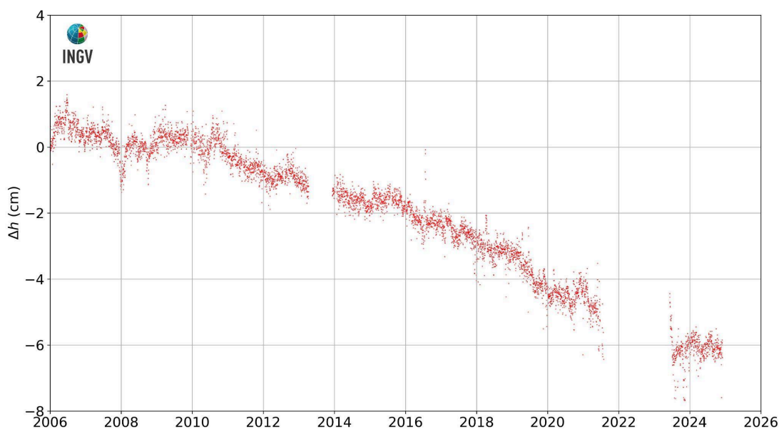
Figura 2.3.3 - Movimenti verticali del suolo, nel periodo gennaio 2006 – novembre 2024, ottenuti dall’analisi dei dati acquisiti dalla stazione mareografica di Torre del Greco, molo Redentore (TRDG). Le variazioni, riportate in cm, rappresentano le medie giornaliere e sono riferite alla stazione mareografica di Napoli molo San Vincenzo (NAMM).
