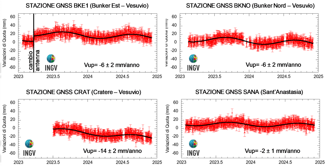
Figura 2.1.2 - Serie temporali delle variazioni giornaliere della componente verticale delle stazioni BKE1, BKNO, CRAT e SANA (Vesuvio) da gennaio 2023 a novembre 2024.
