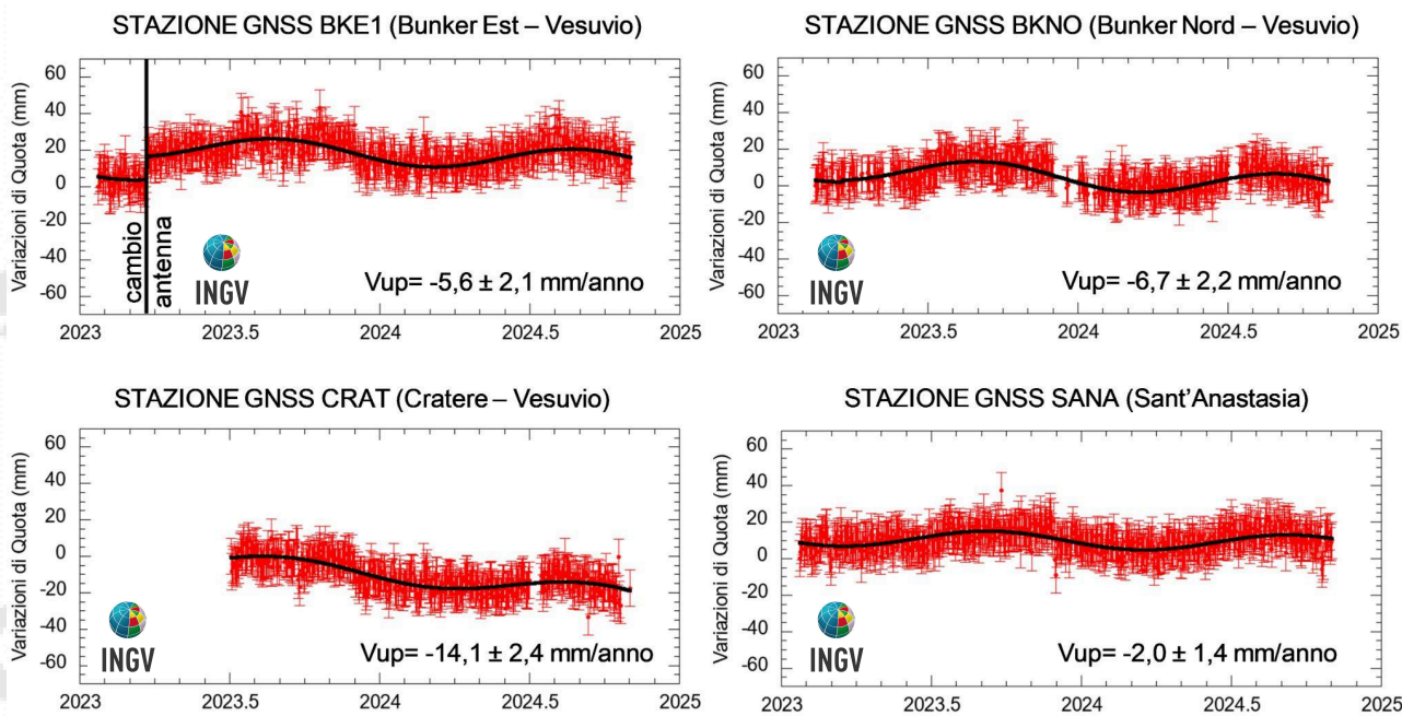
Figura 2.1.2 - Serie temporali delle variazioni giornaliere della componente verticale delle stazioni BKE1, BKNO, CRAT e SANA (Vesuvio) da gennaio 2023 a ottobre 2024.
