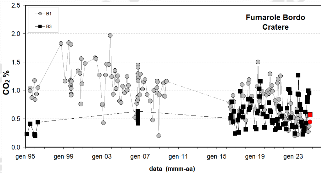
Figura 4.2 - Cronogramma della concentrazione di CO 2 delle fumarole di bordo cratere B1 (area anemometro) e B3 (setto SW). I campioni delle fumarole B1 e B3 del mese di ottobre 2024 sono riportati con il simbolo rosso.
