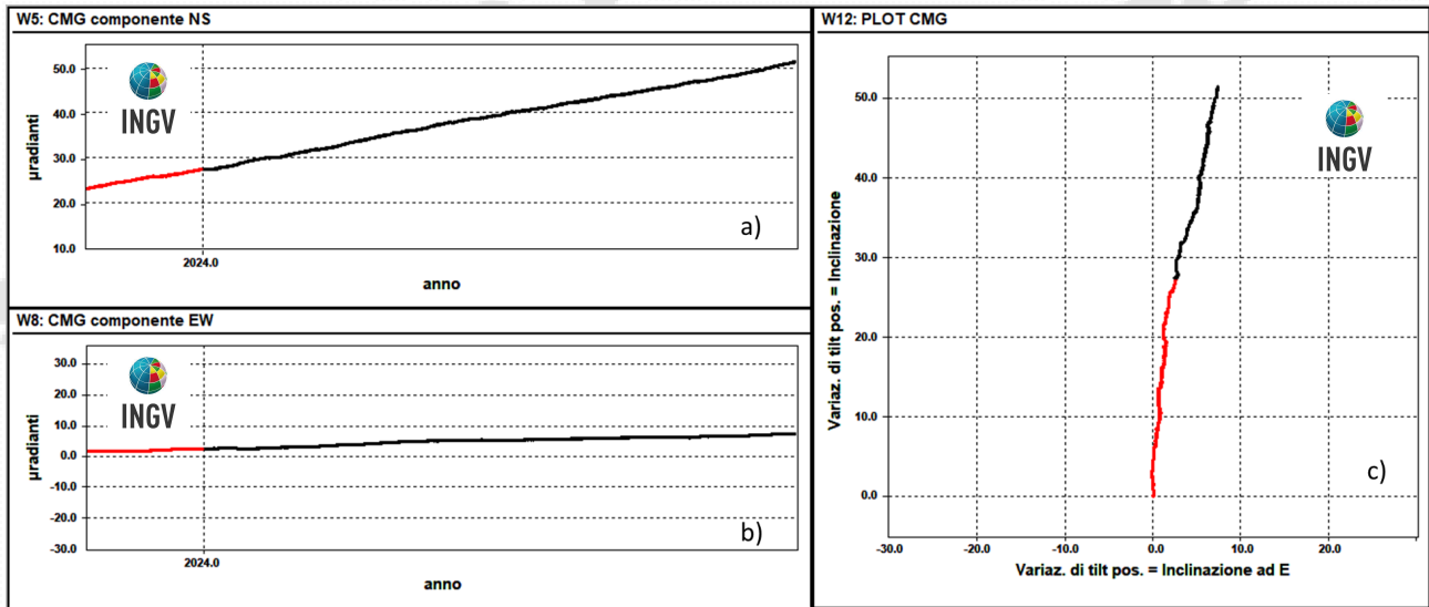
Figura 2.2.2 – Serie temporali e plot del tilt della stazione CMG della rete del Vesuvio registrati negli ultimi 12 mesi (novembre 2023 - ottobre 2024).
