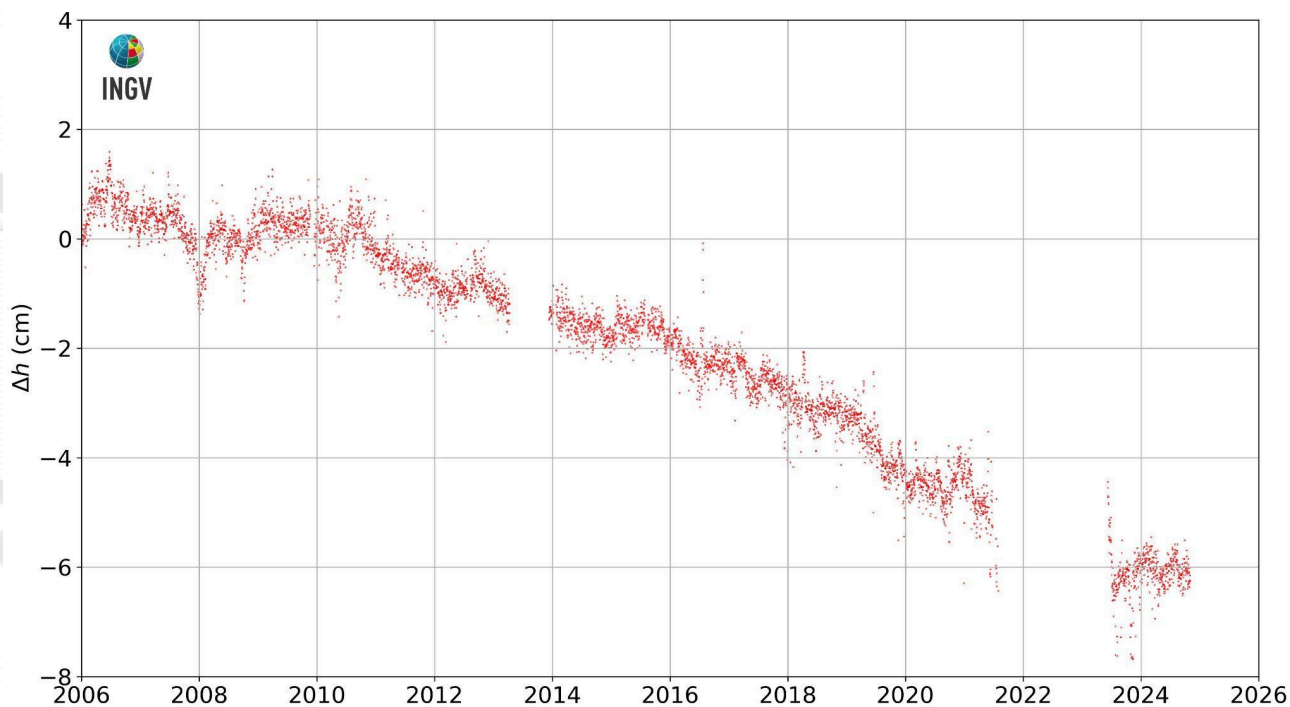
Figura 2.3.3 - Movimenti verticali del suolo, nel periodo gennaio 2006 – ottobre 2024, ottenuti dall'analisi dei dati acquisiti dalla stazione mareografica di Torre del Greco, molo Redentore (TRDG). Le variazioni, riportate in cm, rappresentano le medie giornaliere e sono riferite alla stazione mareografica di Napoli molo San Vincenzo (NAMM).
