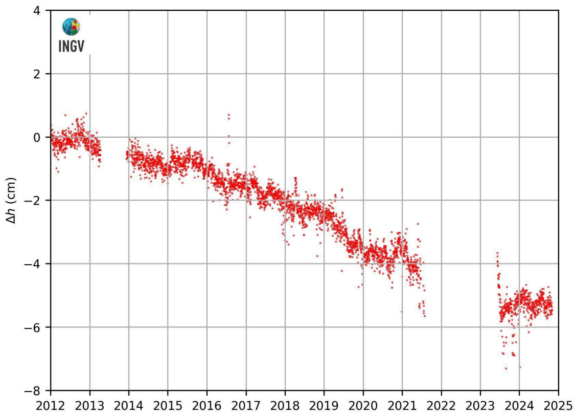
Figura 2.3.2 – Movimenti verticali del suolo, nel periodo gennaio 2012 – ottobre 2024, ottenuti dall’analisi dei dati acquisiti dalla stazione mareografica di Torre del Greco, molo Redentore (TRDG). Le variazioni, riportate in cm, rappresentano le medie giornaliere e sono riferite alla stazione mareografica di Napoli, molo San Vincenzo (NAMM).
