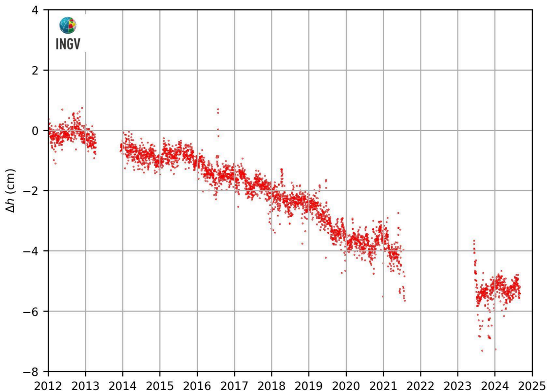
Figura 2.3.2 – Movimenti verticali del suolo, nel periodo gennaio 2012 – agosto 2024, ottenuti dall’analisi dei dati acquisiti dalla stazione mareografica di Torre del Greco, molo Redentore (TRDG). Le variazioni, riportate in cm, rappresentano le medie giornaliere e sono riferite alla stazione mareografica di Napoli, molo San Vincenzo (NAMM).
