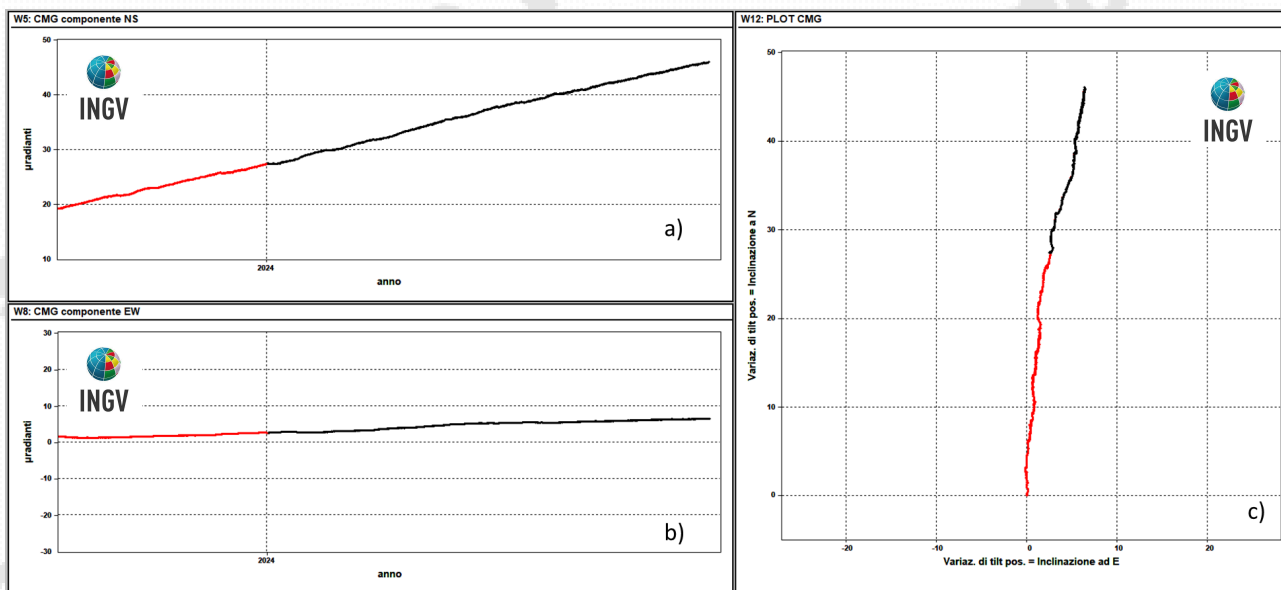
Figura 2.2.2 – Serie temporali e plot del tilt della stazione CMG della rete del Vesuvio registrati negli ultimi 12 mesi (settembre 2023 - agosto 2024).
