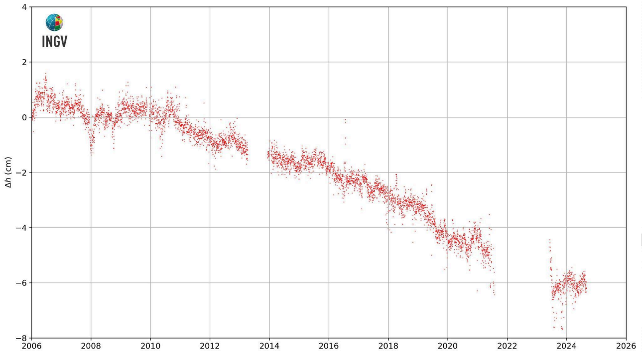
Figura 2.3.3 - Movimenti verticali del suolo, nel periodo gennaio 2006 - agosto 2024, ottenuti dall'analisi dei dati acquisiti dalla stazione mareografica di Torre del Greco, molo Redentore (TRDG). Le variazioni, riportate in cm, rappresentano le medie giornaliere e sono riferite alla stazione mareografica di Napoli molo San Vincenzo (NAMM).
