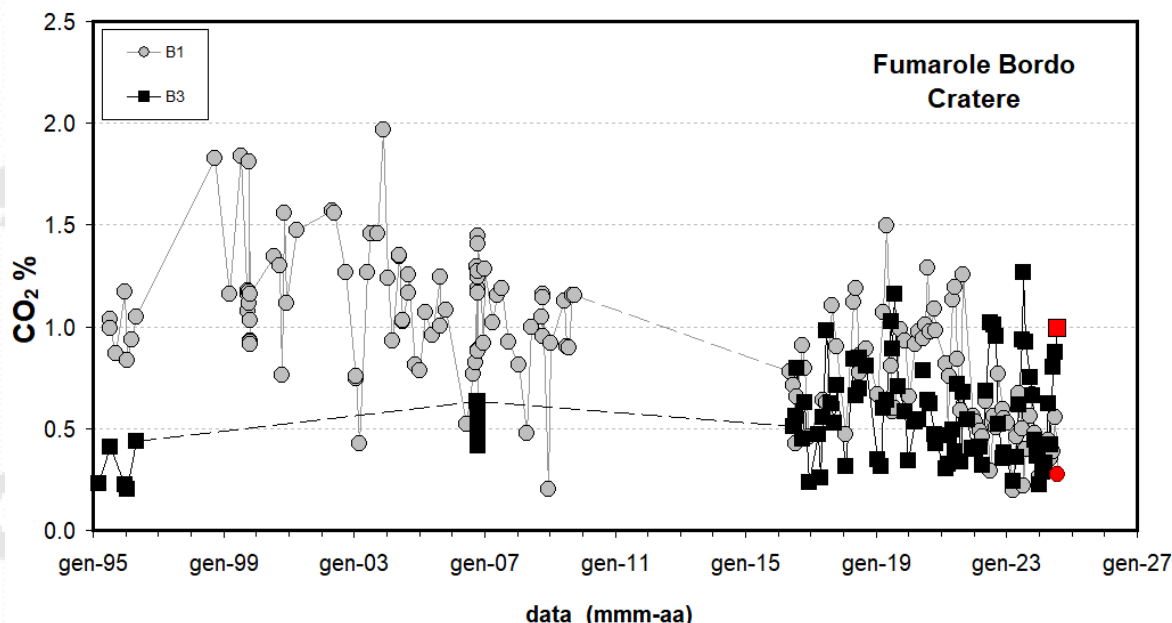
Figura 4.2 - Cronogramma della concentrazione di CO 2 delle fumarole di bordo cratere B1 (area anemometro) e B3 (settore SW). I campioni delle fumarole B1 e B3 del mese di agosto 2024 sono riportati con il simbolo rosso.
