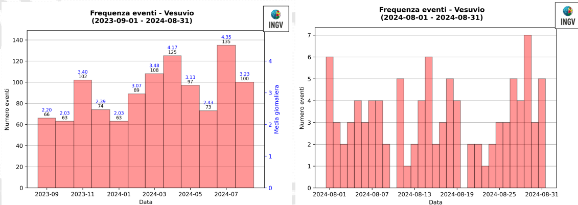
Figura 1.2 - A sinistra il numero di eventi registrati al Vesuvio nel corso degli ultimi 12 mesi (in totale 1095), mentre a destra quelli avvenuti nell'ultimo mese (in totale 100).
