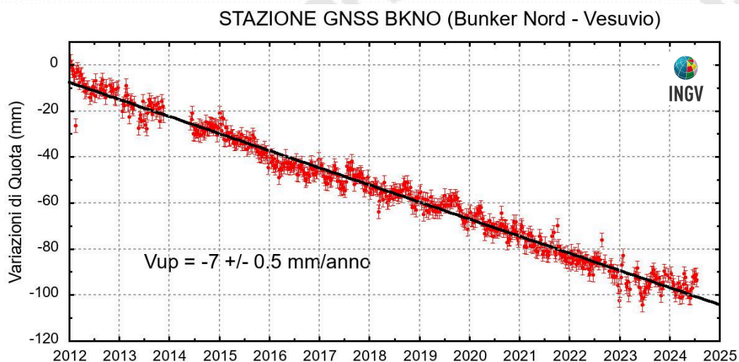
Figura 2.1.2 - Serie temporale delle variazioni settimanali in quota della stazione BKNO (Vesuvio) da gennaio 2012 a luglio 2024.
