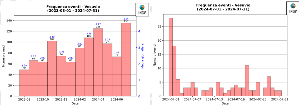
Figura 1.2 - A sinistra il numero di eventi registrati al Vesuvio nel corso degli ultimi 12 mesi (in totale 1044), mentre a destra quelli avvenuti nell'ultimo mese (in totale 135).
