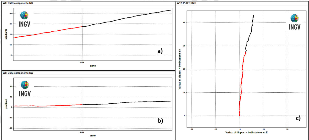
Figura 2.2.2 – Serie temporali e plot del tilt della stazione CMG della rete del Vesuvio registrati negli ultimi 12 mesi (agosto 2023 - luglio 2024).
