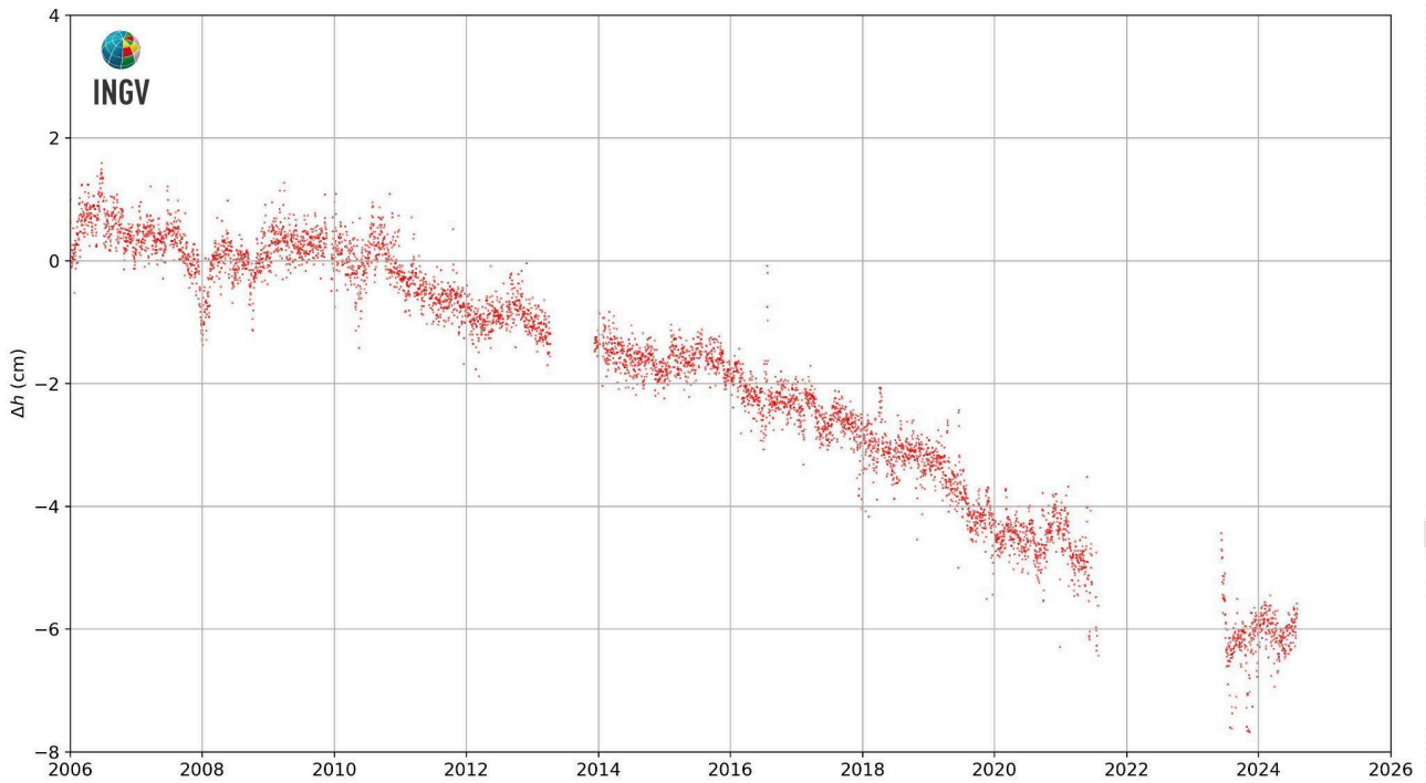
Figura 2.3.3 - Movimenti verticali del suolo, nel periodo gennaio 2006 - luglio 2024, ottenuti dall'analisi dei dati acquisiti dalla stazione mareografica di Torre del Greco, molo Redentore (TRDG). Le variazioni, riportate in cm, rappresentano le medie giornaliere e sono riferite alla stazione mareografica di Napoli molo San Vincenzo (NAMM).
