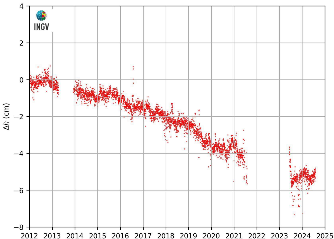
Figura 2.3.2 – Movimenti verticali del suolo, nel periodo gennaio 2012 – luglio 2024, ottenuti dall'analisi dei dati acquisiti dalla stazione mareografica di Torre del Greco, molo Redentore (TRDG). Le variazioni, riportate in cm, rappresentano le medie giornaliere e sono riferite alla stazione mareografica di Napoli, molo San Vincenzo (NAMM).
