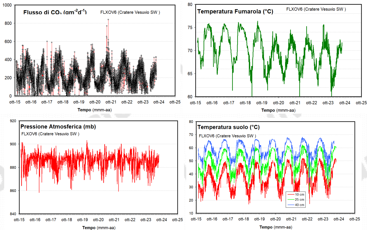
Figura 4.5 - Parametri misurati dalla stazione geochimica (FLXOV6) installata in area bordo cratere del Vesuvio (settore SW). I valori, eccetto il flusso di CO 2 dal suolo, sono riportati come medie giornaliere.
