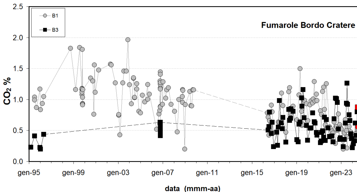
Figura 4.4 - Cronogramma della concentrazione di CO 2 delle fumarole di bordo cratere B1 (area anemometro) e B3 (settore SW). I campioni delle fumarole B1 e B3 del mese di giugno 2024 sono riportati con il simbolo rosso.
