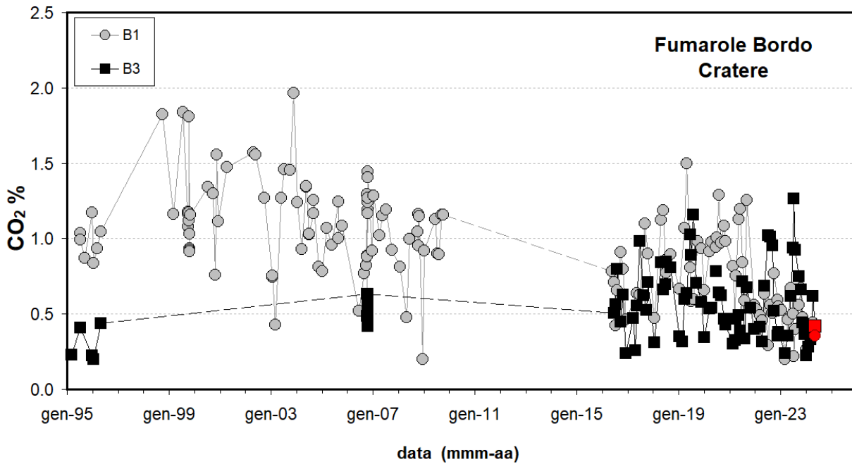
Figura 4.2 - Cronogramma della concentrazione di CO 2 delle fumarole di bordo cratere B1 (area anemometro) e B3 (settore SW). I campioni delle fumarole B1 e B3 del mese di giugno 2024 sono riportati con il simbolo rosso.
