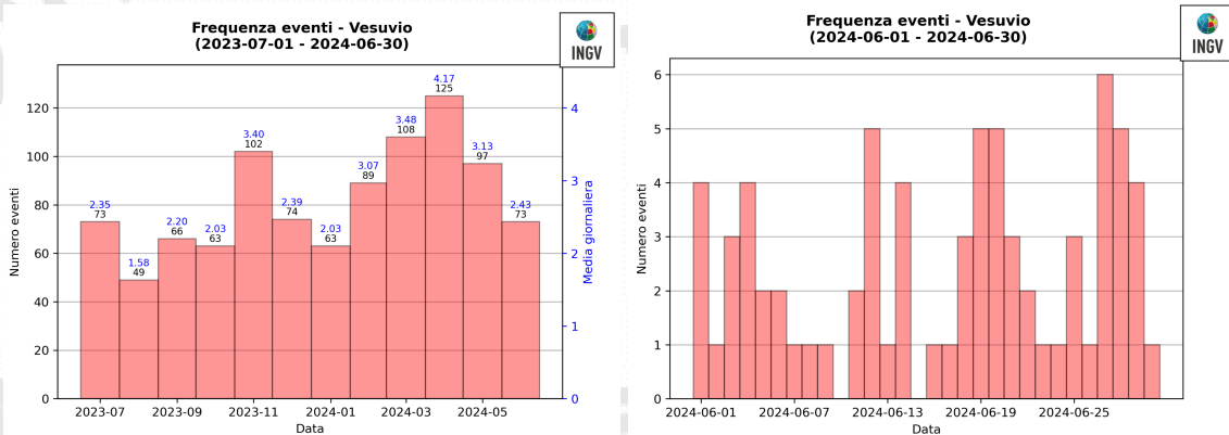
Figura 1.2 - A sinistra il numero di eventi registrati al Vesuvio nel corso degli ultimi 12 mesi (in totale 982), mentre a destra quelli avvenuti nell'ultimo mese (in totale 73).
