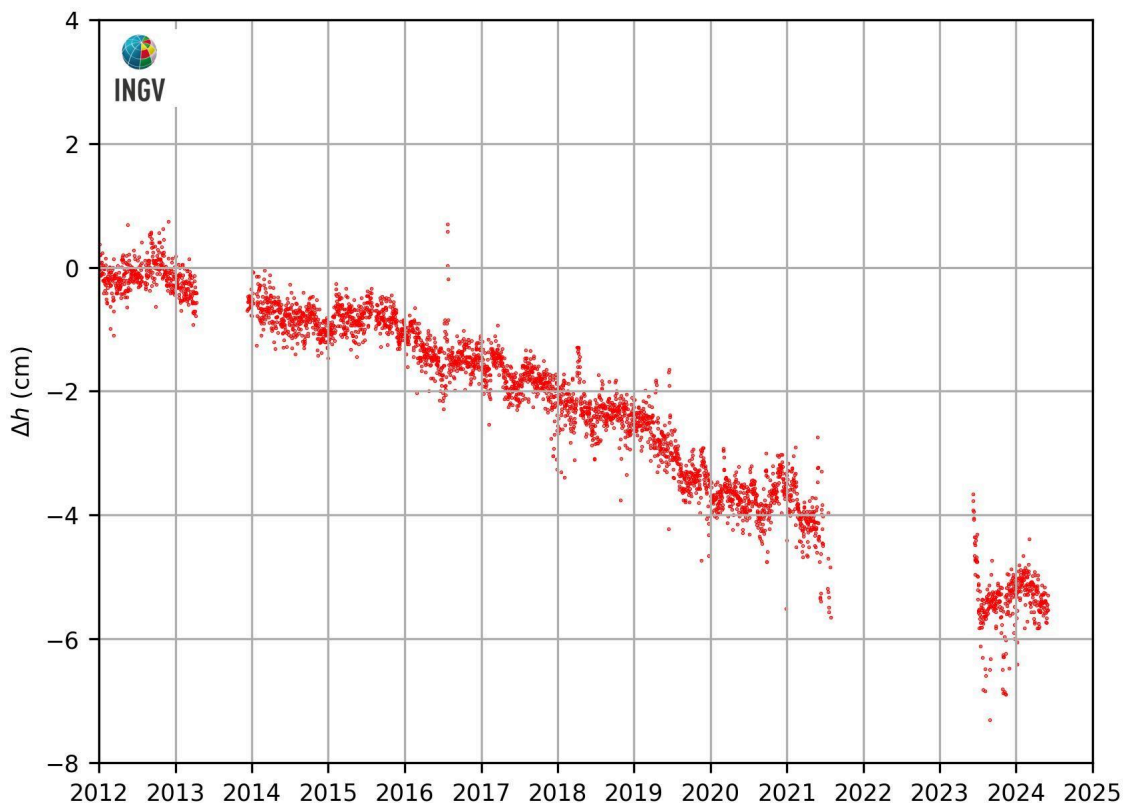
Figura 2.3.2 – Movimenti verticali del suolo, nel periodo gennaio 2012 – maggio 2024, ottenuti dall’analisi dei dati acquisiti dalla stazione mareografica di Torre del Greco, molo Redentore (TRDG). Le variazioni, riportate in cm, rappresentano le medie giornaliere e sono riferite alla stazione mareografica di Napoli, molo San Vincenzo (NAMM).
