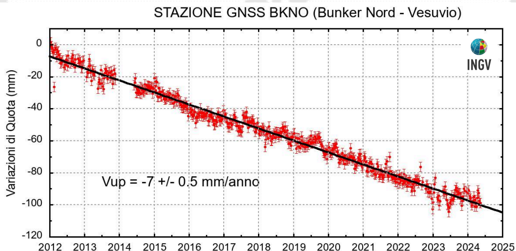
Figura 2.1.2 - Serie temporale delle variazioni settimanali in quota della stazione BKNO (Vesuvio) da gennaio 2012 a maggio 2024.
