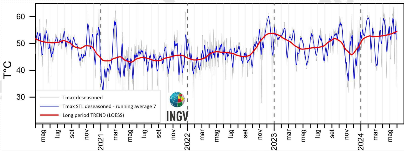
Figura 3.1.2 - Stazione Vesuvio VES1. Serie temporali dei valori di temperatura massima giornaliera rilevata nelle immagini IR, destagionalizzate mediante applicazione dell' algoritmo BR (medie settimanali termocamera 640x480). Il trend a lungo termine è ottenuto applicando un fitting LOESS di 2° alle temperature massime destagionalizzate.
