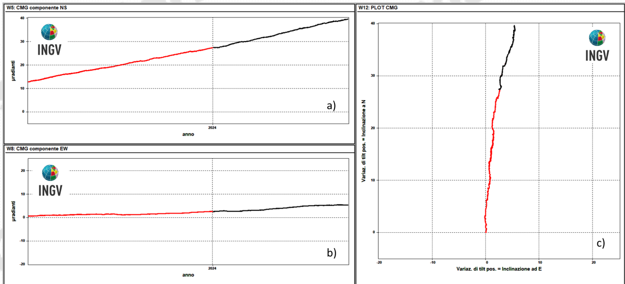
Figura 2.2.2 – Serie temporali e plot del tilt della stazione CMG della rete del Vesuvio registrati negli ultimi 12 mesi (giugno 2023 - maggio 2024).
