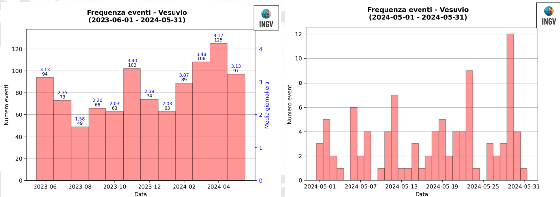
Figura 1.2 - A sinistra il numero di eventi registrati al Vesuvio nel corso degli ultimi 12 mesi (in totale 1119), mentre a destra quelli avvenuti nell'ultimo mese (in totale 97).
