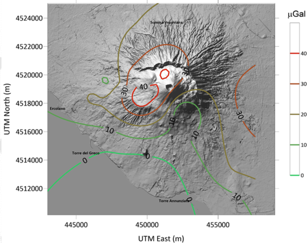
Figura 2.4.2 Variazioni di gravità \Delta g , con riferimento al vertice di Napoli S. Marcellino, ottenute tra la campagna di aprile 2024 e maggio 2023. L'equidistanza delle isolinee è di 10\mu\text{Gal} , l'errore totale stimato sulla rete nel 2023 è pari a \pm 8\mu\text{Gal} e a \pm 10\mu\text{Gal} per la campagna 2024.
