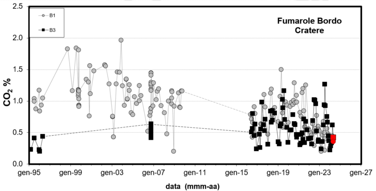
Figura 4.2 - Cronogramma della concentrazione di CO 2 delle fumarole di bordo cratere B1 (area anemometro) e B3 (settore SW). I campioni delle fumarole B1 e B3 del mese di maggio 2024 sono riportati con il simbolo rosso.
