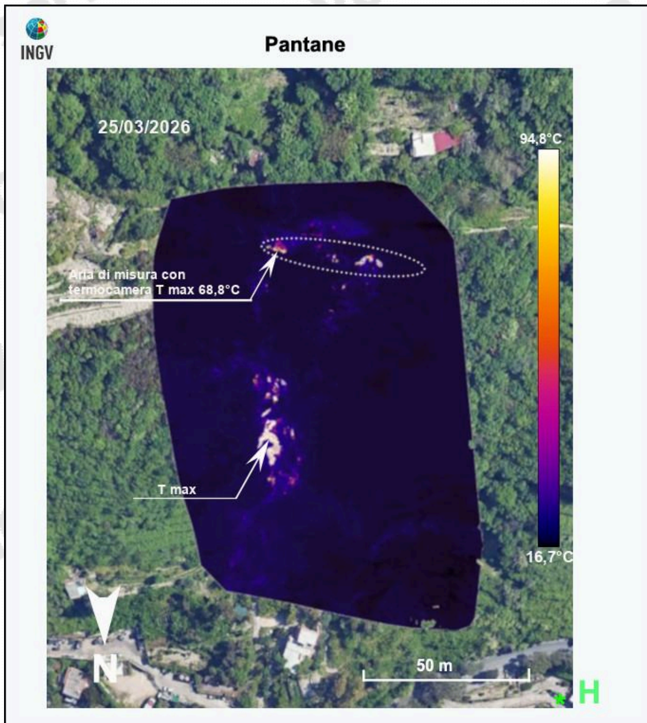
Figura 3.4 – Località Pantane. Fotocomposizione di immagini termiche rilevate da drone nel mese di marzo 2026. H* indica il sito di decollo e di atterraggio del drone. L'area racchiusa dalla linea tratteggiata bianca è quella vengono effettuate le misure termiche mensili (sito "Pan" di Figura 3.1).
