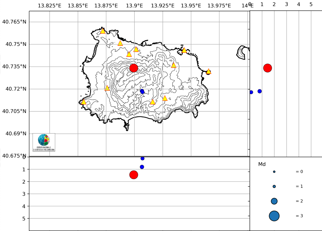
Figura 1.2 - Localizzazioni ipocentrali ad Ischia nel corso degli ultimi 12 mesi (in blu) e dell'ultimo mese (In rosso). La dimensione dei simboli è proporzionale alla magnitudo, come indicato nel riquadro in basso.
