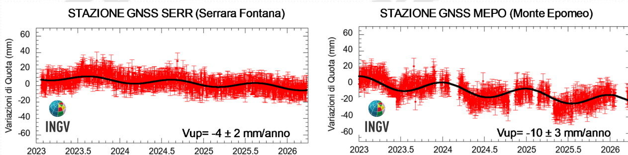
Figura 2.1.2 - Serie temporali delle variazioni giornaliere della componente verticale delle stazioni di SERR e MEPO (Ischia) da gennaio 2023 a marzo 2026.
