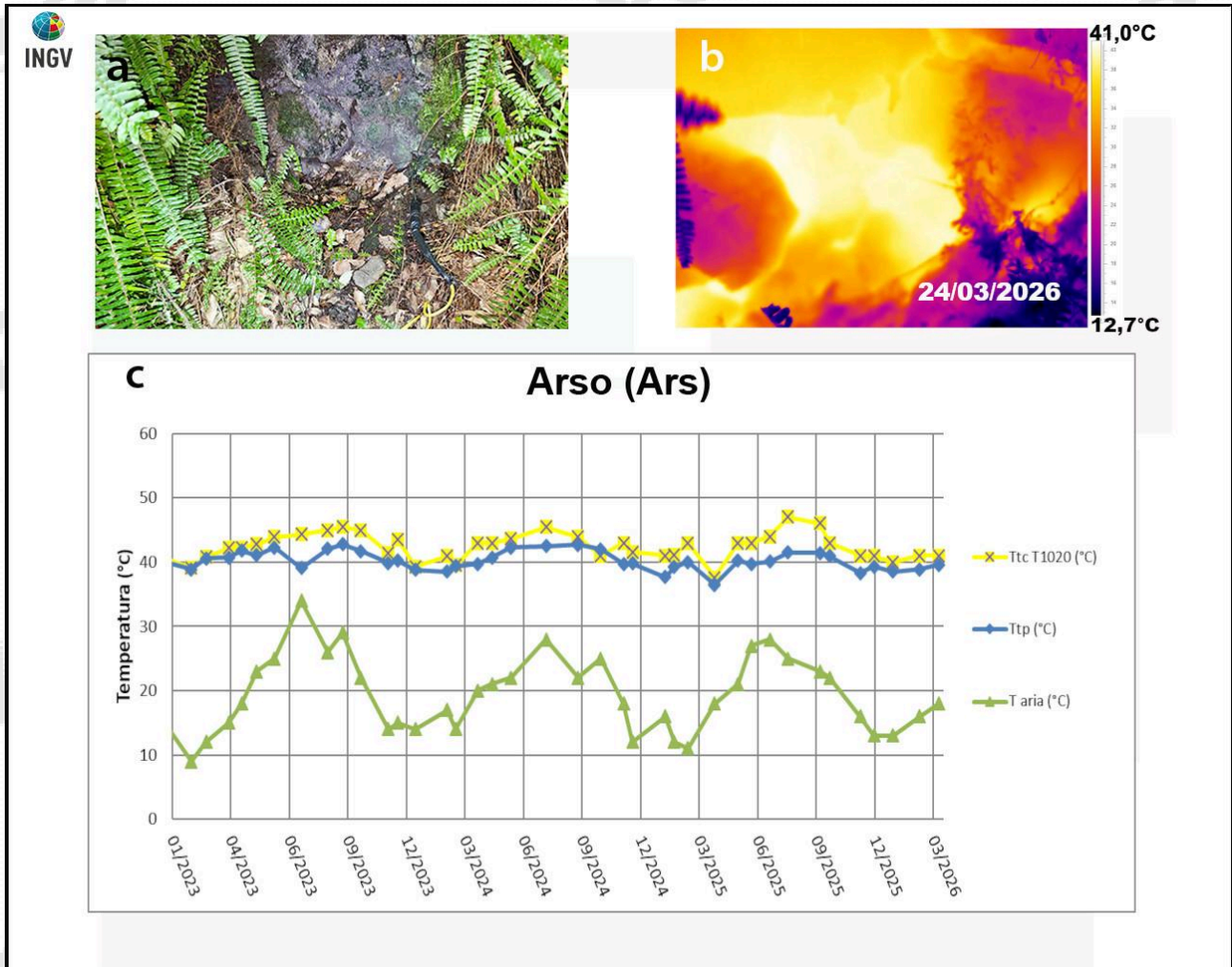
Figura 3.2 - Cratere dell'Arso a Ischia. Immagini nel visibile (a) e termica (b) riprese dal punto stazione Ars di Figura 3.1. Il grafico (c) riporta la serie temporale (gennaio 2023 – marzo 2026) dei valori massimi di temperatura con termocamera FLIR T1020 (TtcT1020) e con termocoppia (Ttp), confrontati con la temperatura dell'aria (Taria) misurata nel momento del rilievo termico.
