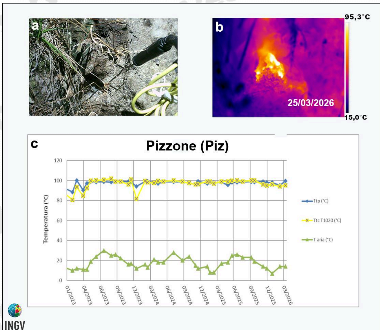
Figura 3.5 – Fumarola in località Pizzone a Ischia. Immagini nel visibile (a) e termica (b) riprese dal punto stazione Piz di Fig. 3.1. Il grafico (c) riporta la serie temporale (gennaio 2023 – marzo 2026) dei valori massimi di temperatura con termocamera FLIR T1020 (TtcT1020) e con termocoppia (Ttp), confrontati con la temperatura dell’aria (Taria) misurata nel momento del rilievo termico.
