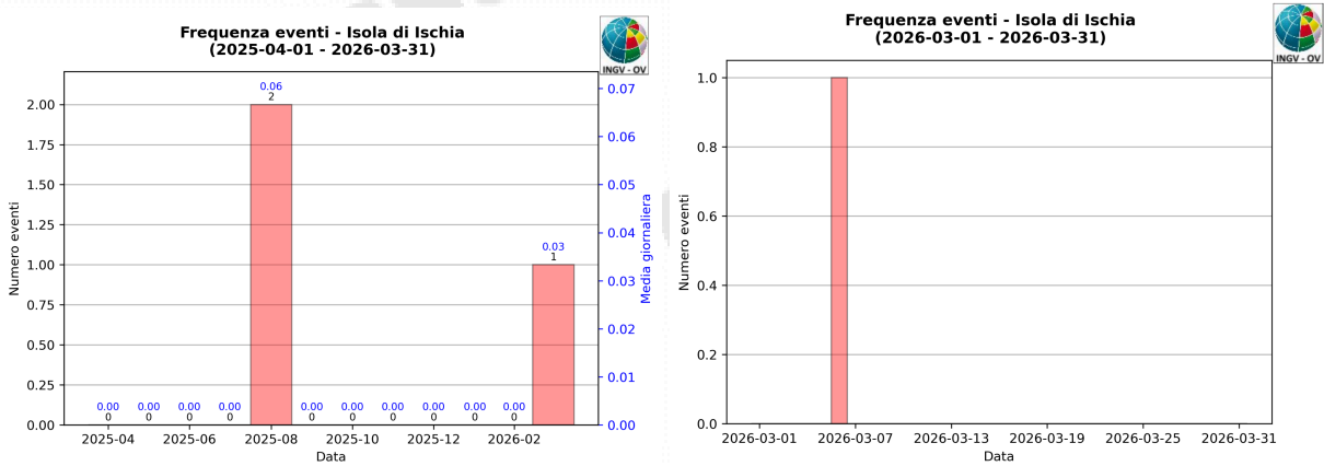
Figura 1.3 – Numero di eventi registrati ad Ischia nel corso degli ultimi 12 mesi (in totale 3), a sinistra, e nel corso dell'ultimo mese (in totale 1), a destra.
