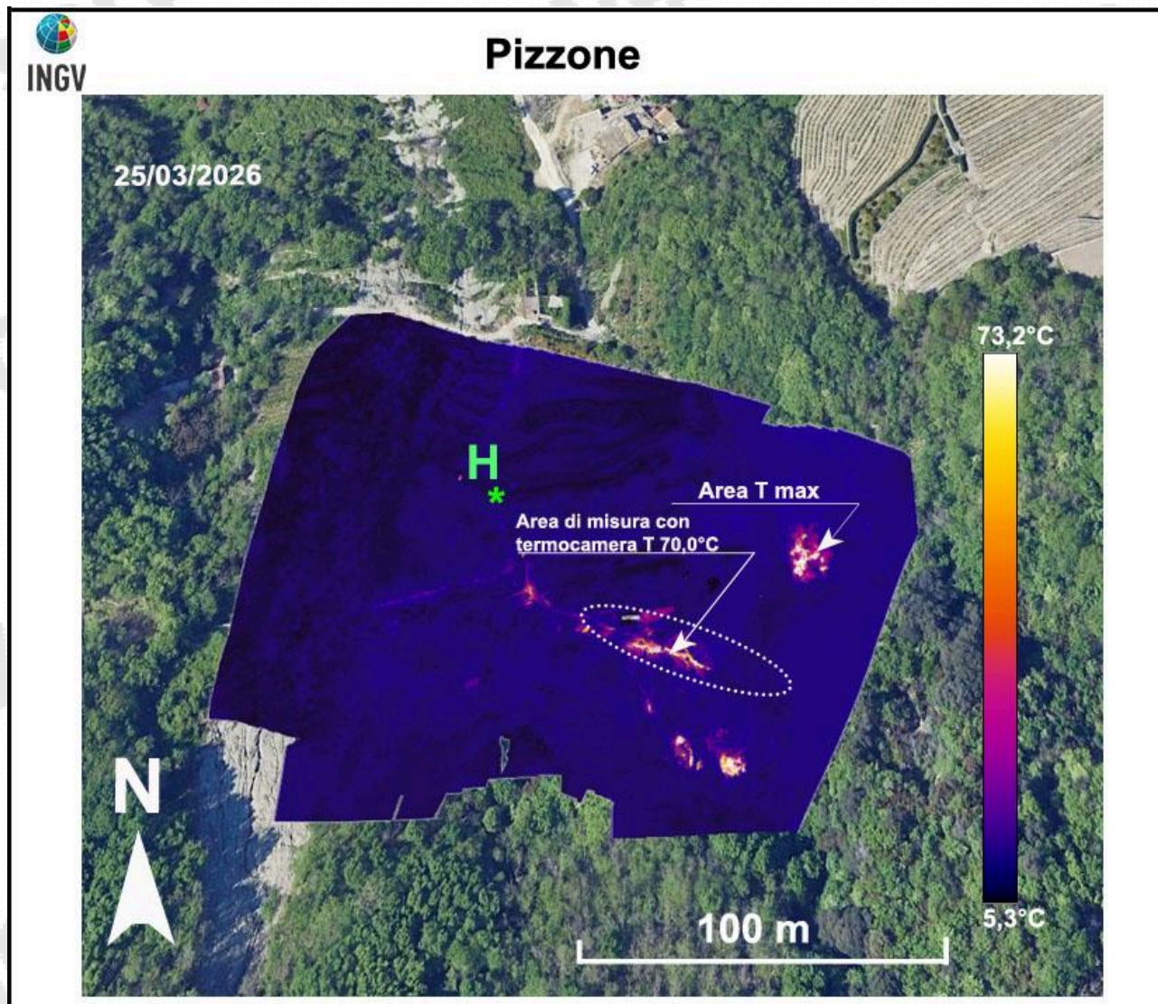
Figura 3.6 – Località Pizzone. Fotocomposizione di immagini termiche rilevate da drone nel mese di marzo 2026. H* indica il sito di decollo e di atterraggio del drone. L'area racchiusa dalla linea tratteggiata bianca è quella dove vengono effettuate le misure termiche mensili (sito "Piz" di Figura 3.1).
