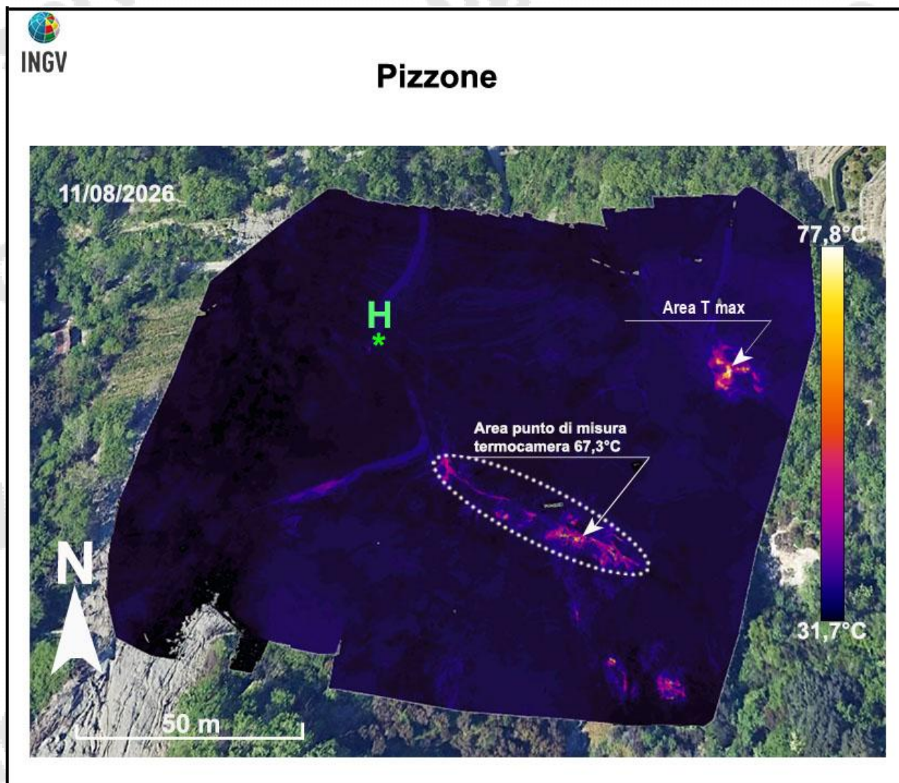
Figura 3.5 – Località Pizzone. Fotocomposizione di immagini termiche rilevate da drone nel mese di agosto 2026 (area rosa “Piz” in Figura 3.1). H* indica il sito di decollo e di atterraggio del drone. L’area racchiusa dalla linea tratteggiata bianca è quella dove vengono effettuate le misure termiche discrete (sito “Piz” di Figura 3.1).
