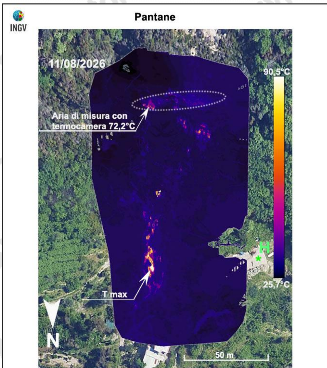
Figura 3.3 – Località Pantane. Fotocomposizione di immagini termiche rilevate da drone nel mese di agosto 2026 (area rosa "Pan" in Figura 3.1). H* indica il sito di decollo e di atterraggio del drone. L'area racchiusa dalla linea tratteggiata bianca è quella vengono effettuate le misure termiche discrete (sito "Pan" di Figura 3.1).
