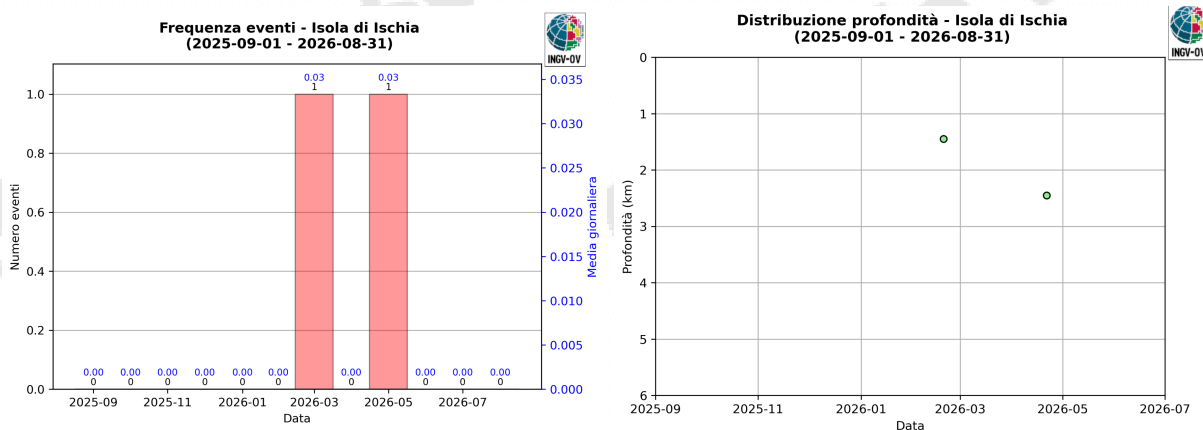
Figura 1.3 – (A sinistra) Numero di eventi registrati ad Ischia nel corso degli ultimi 12 mesi (in totale 2). (A destra) Profondità ipocentrali degli eventi registrati ad Ischia nel corso degli ultimi 12 mesi.
