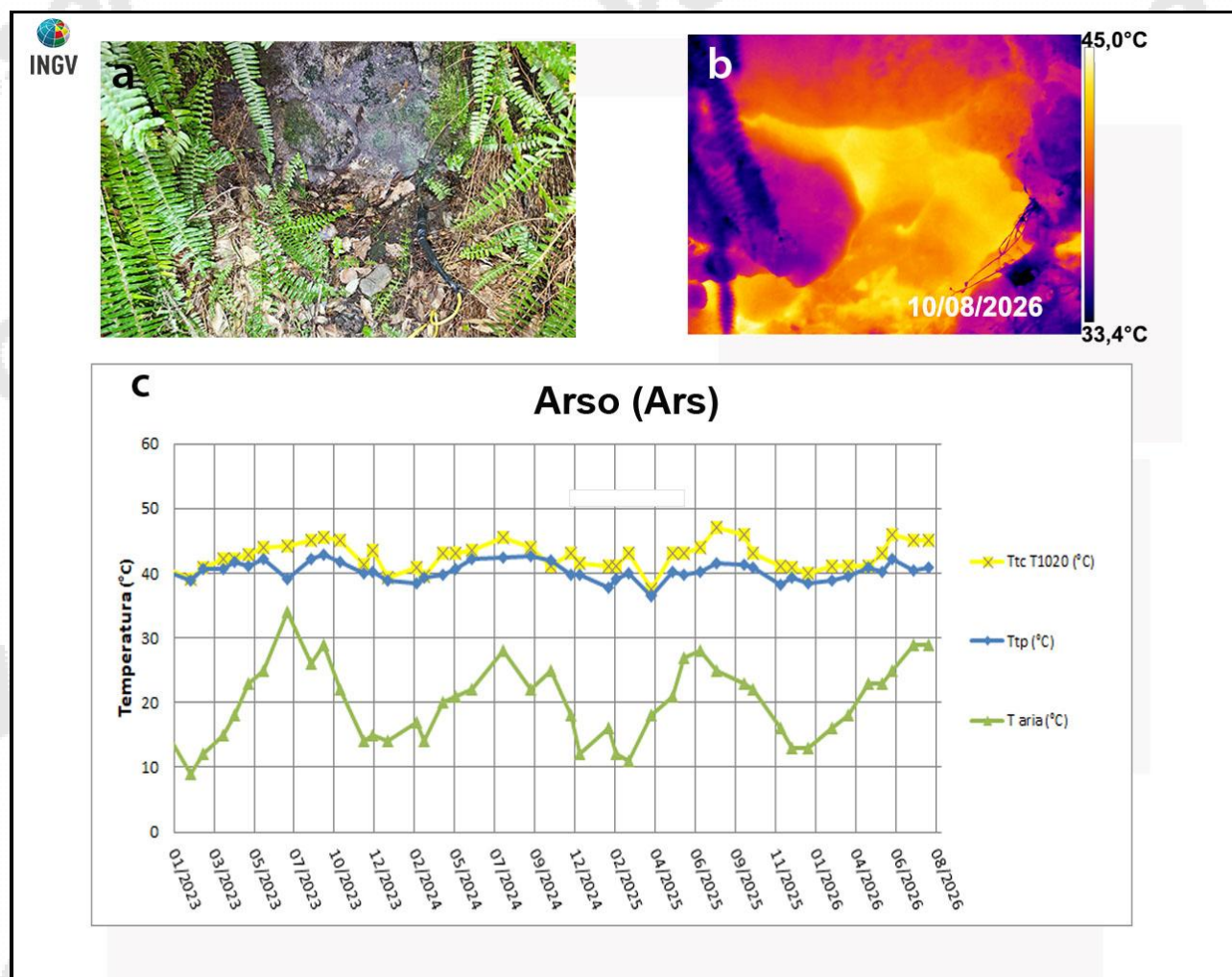
Figura 3.2 - Cratere dell'Arso a Ischia. Immagini nel visibile (a) e termica (b) riprese dal punto stazione Ars di Figura 3.1. Il grafico (c) riporta la serie temporale (gennaio 2023 – agosto 2026) dei valori massimi di temperatura con termocamera FLIR T1020 (TtcT1020) e con termocoppia (Ttp), confrontati con la temperatura dell'aria (Taria) misurata nel momento del rilievo termico.
