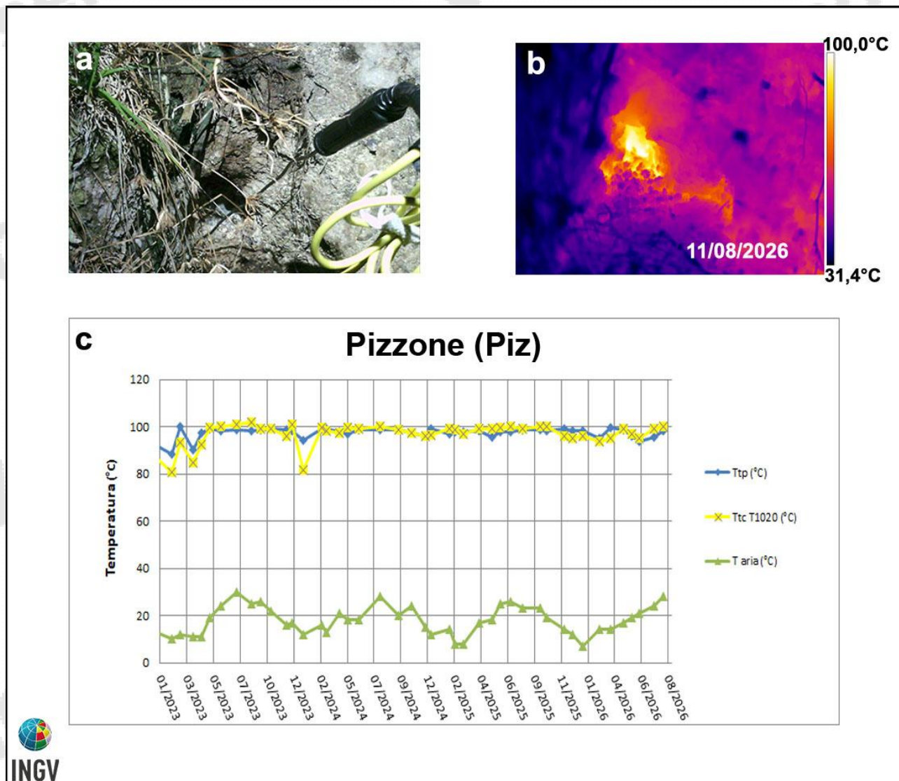
Figura 3.4 – Fumarola in località Pizzone a Ischia. Immagini nel visibile (a) e termica (b) riprese dal punto stazione Piz di Fig. 3.1. Il grafico (c) riporta la serie temporale (gennaio 2023 – agosto 2026) dei valori massimi di temperatura con termocamera FLIR T1020 (TtcT1020) e con termocoppia (Ttp), confrontati con la temperatura dell'aria (Taria) misurata nel momento del rilievo termico.
