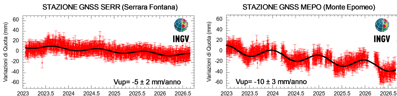
Figura 2.1.2 - Serie temporali delle variazioni giornaliere della componente verticale delle stazioni di SERR e MEPO (Ischia) da gennaio 2023 ad agosto 2026.
