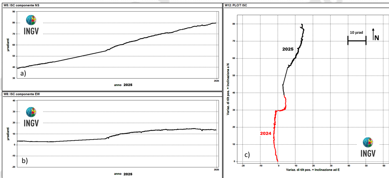
Figura 2.2.2 - Serie temporali (ultimi 12 mesi) e plot (2024-2025) del tilt della stazione ISC della rete di Ischia.
