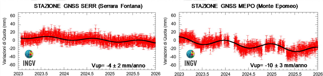
Figura 2.1.2 - Serie temporali delle variazioni giornaliere della componente verticale delle stazioni di SERR e MEPO (Ischia) da gennaio 2023 a dicembre 2025.
