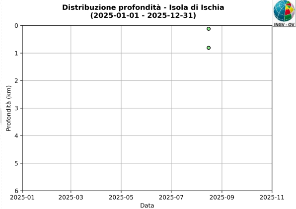
Figura 1.3 – (A sinistra) Numero di eventi registrati ad Ischia nel corso degli ultimi 12 mesi (in totale 2). (A destra) profondità ipocentrali degli eventi registrati ad Ischia nel corso degli ultimi 12 mesi.
