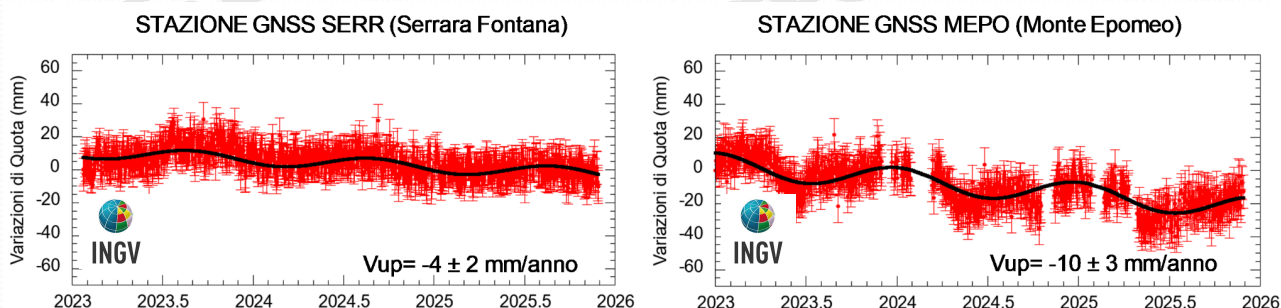
Figura 2.1.2 - Serie temporali delle variazioni giornaliere della componente verticale delle stazioni di SERR e MEPO (Ischia) da gennaio 2023 a novembre 2025.
