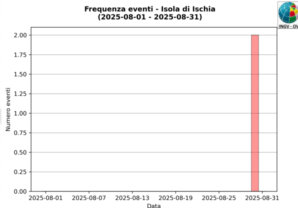
Figura 1.3 – Numero di eventi registrati ad Ischia nel corso degli ultimi 24 mesi (in totale 8), a sinistra, e nel corso dell'ultimo mese (in totale 2), a destra.
