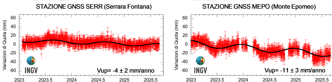
Figura 2.1.2 - Serie temporali delle variazioni giornaliere della componente verticale delle stazioni di SERR e MEPO (Ischia) da gennaio 2023 ad agosto 2025.
