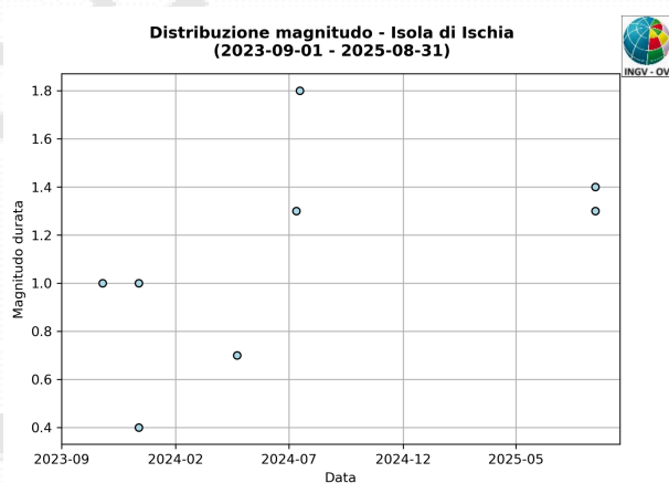
Figura 1.5 – Magnitudo degli eventi registrati ad Ischia nel corso degli ultimi 24 mesi, a sinistra, e nel corso dell'ultimo mese, a destra.
