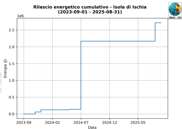
Figura 1.6 – Rilascio cumulativo di energia sismica ad Ischia nel corso degli ultimi 24 mesi, a sinistra, e nel corso dell'ultimo mese, a destra.
