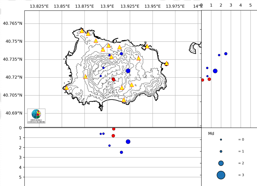
Figura 1.2 - Localizzazioni ipocentrali ad Ischia nel corso degli ultimi 24 mesi (in blu) e dell'ultimo mese (In rosso). La dimensione dei simboli è proporzionale alla magnitudo, come indicato nel riquadro in basso.
