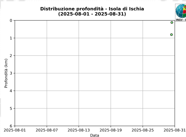
Figura 1.4 – Profondità degli eventi registrati ad Ischia nel corso degli ultimi 24 mesi, a sinistra, e nel corso dell'ultimo mese, a destra,
