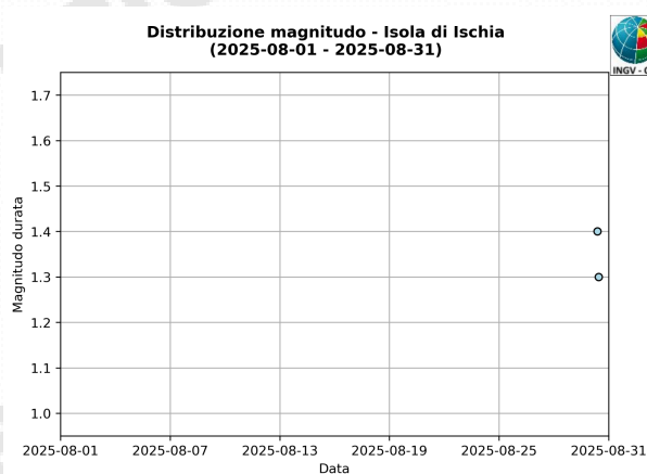
Figura 1.5 – Magnitudo degli eventi registrati ad Ischia nel corso degli ultimi 24 mesi, a sinistra, e nel corso dell'ultimo mese, a destra.
