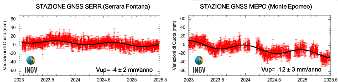
Figura 2.1.2 - Serie temporali delle variazioni giornaliere della componente verticale delle stazioni di SERR e MEPO (Ischia) da gennaio 2023 a giugno 2025.
