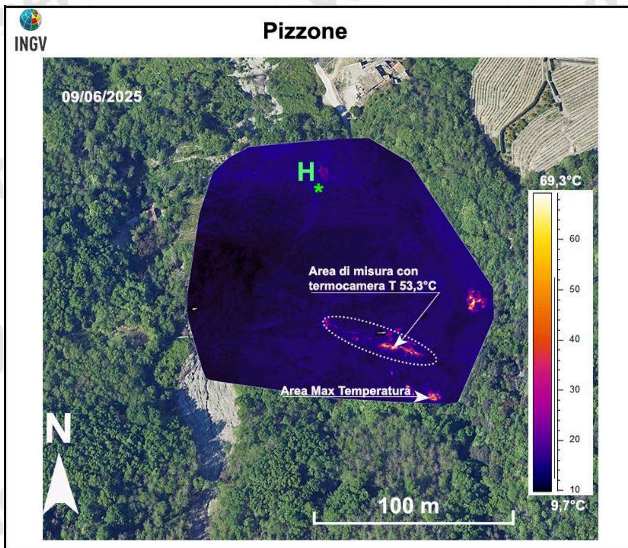
Figura 3.6 – Fotocomposizione di immagini termiche rilevate da drone nel mese di giugno 2025. H indica il sito di decollo e di atterraggio del drone. L'area racchiusa dalla linea tratteggiata è quella dove vengono effettuate le misure termiche mensili nell'area di Pizzone (Fig. 3.1h).
