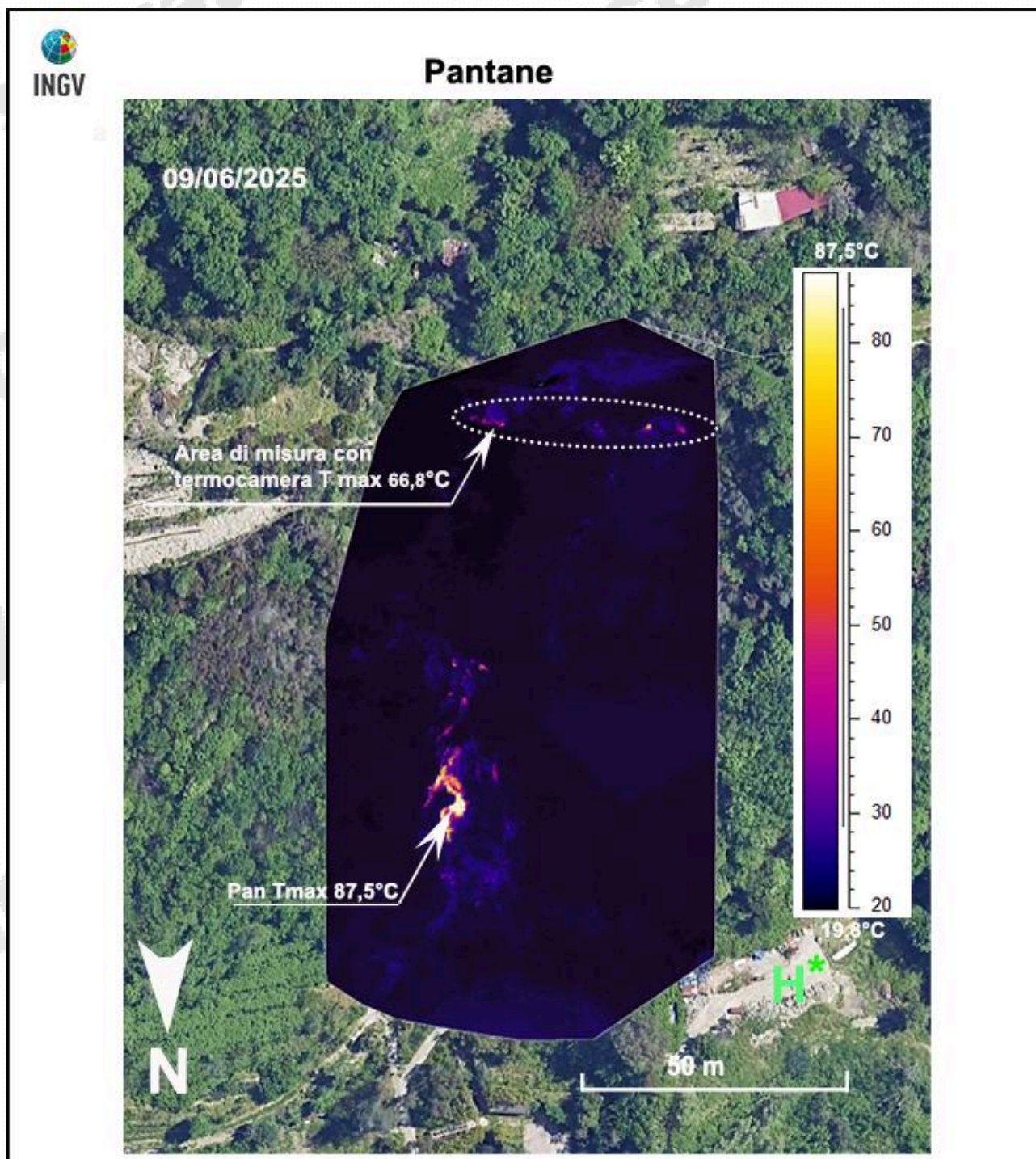
Figura 3.4 – Fotocomposizione di immagini termiche rilevate da drone nel mese di giugno 2025. H* indica il sito di decollo e di atterraggio del drone. L'area racchiusa dalla linea tratteggiata è quella dove vengono effettuate le misure termiche mensili nell'area di Pantane (Fig. 3.1a).
