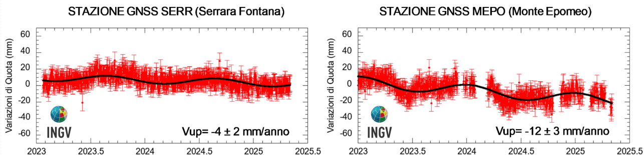
Figura 2.1.2 - Serie temporali delle variazioni giornaliere della componente verticale delle stazioni di SERR e MEPO (Ischia) da gennaio 2023 ad aprile 2025.
